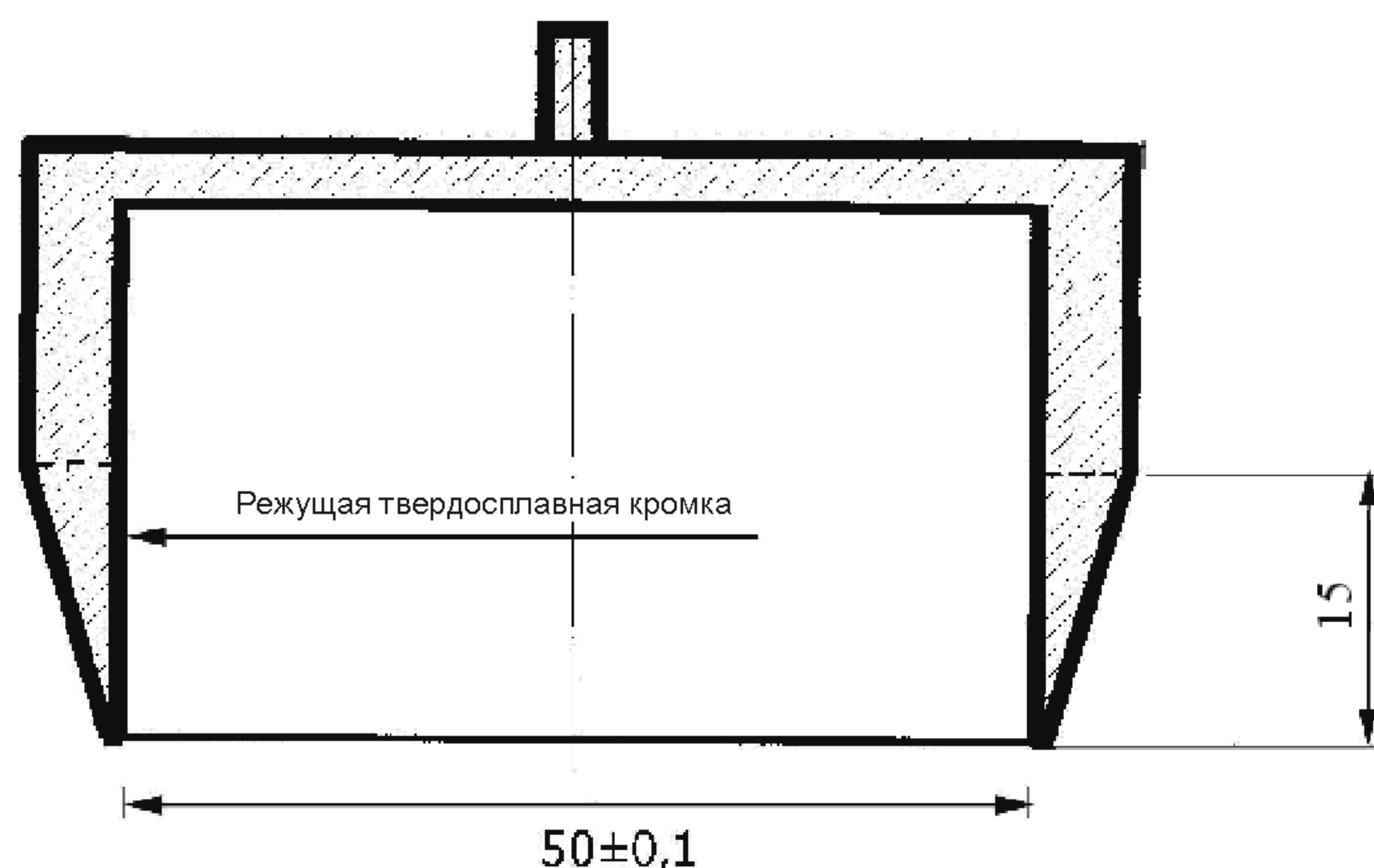
Рисунок 2 — Сверло-коронка с режущей твердосплавной кромкой
