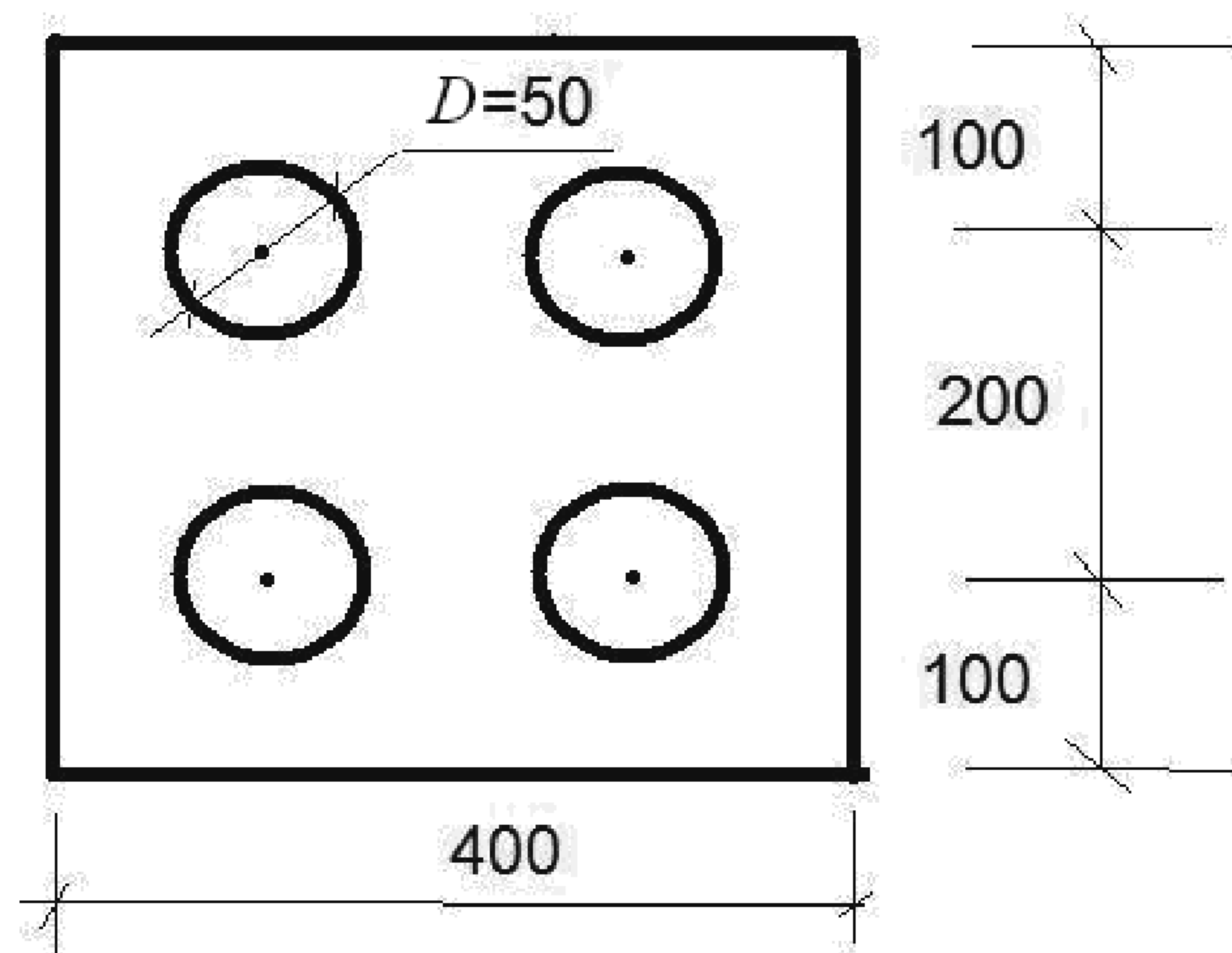
Рисунок 3 — Расположение анкеров на поверхности образца
