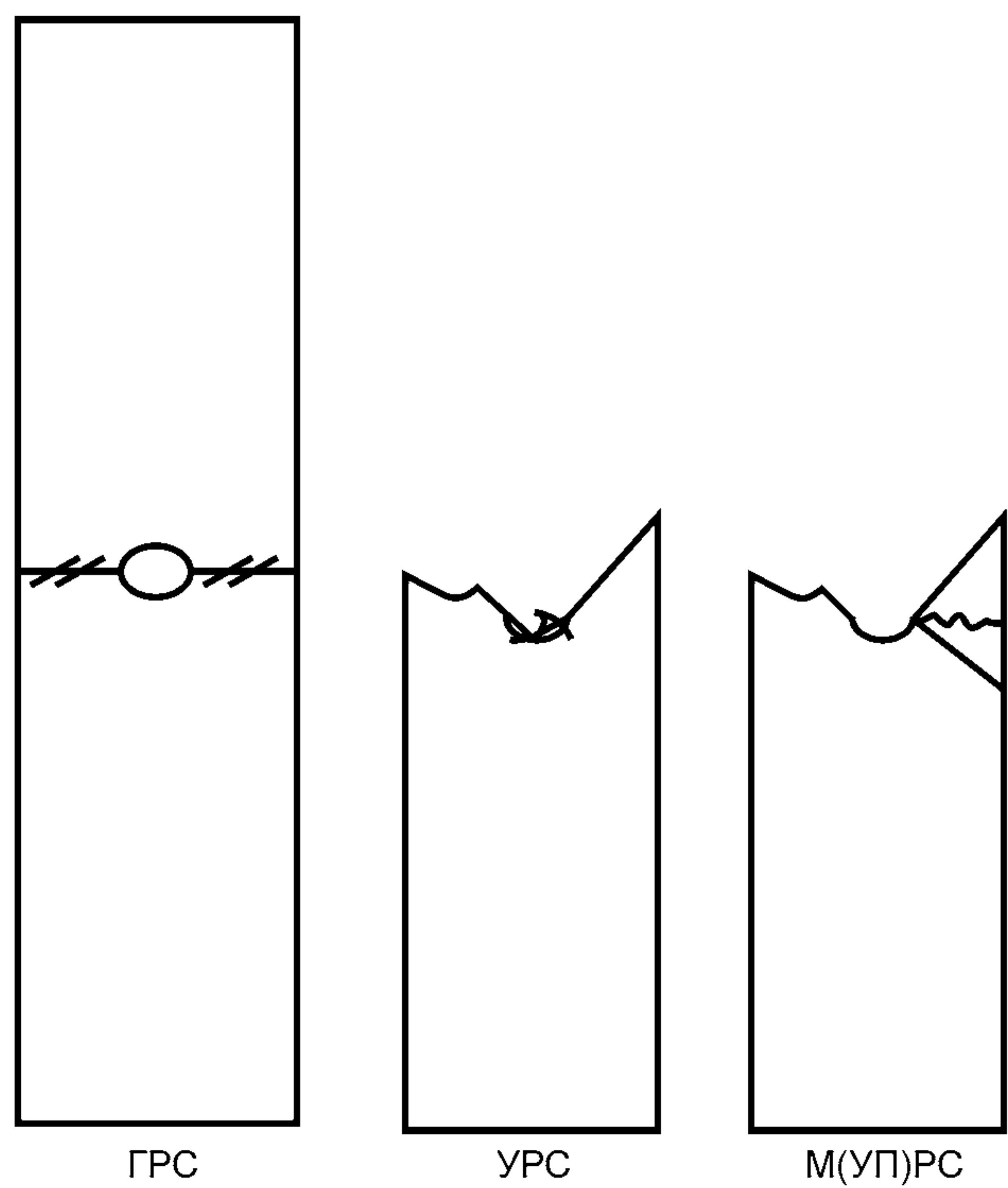
Рисунок 8 — Примеры обозначения типовых разрушений
