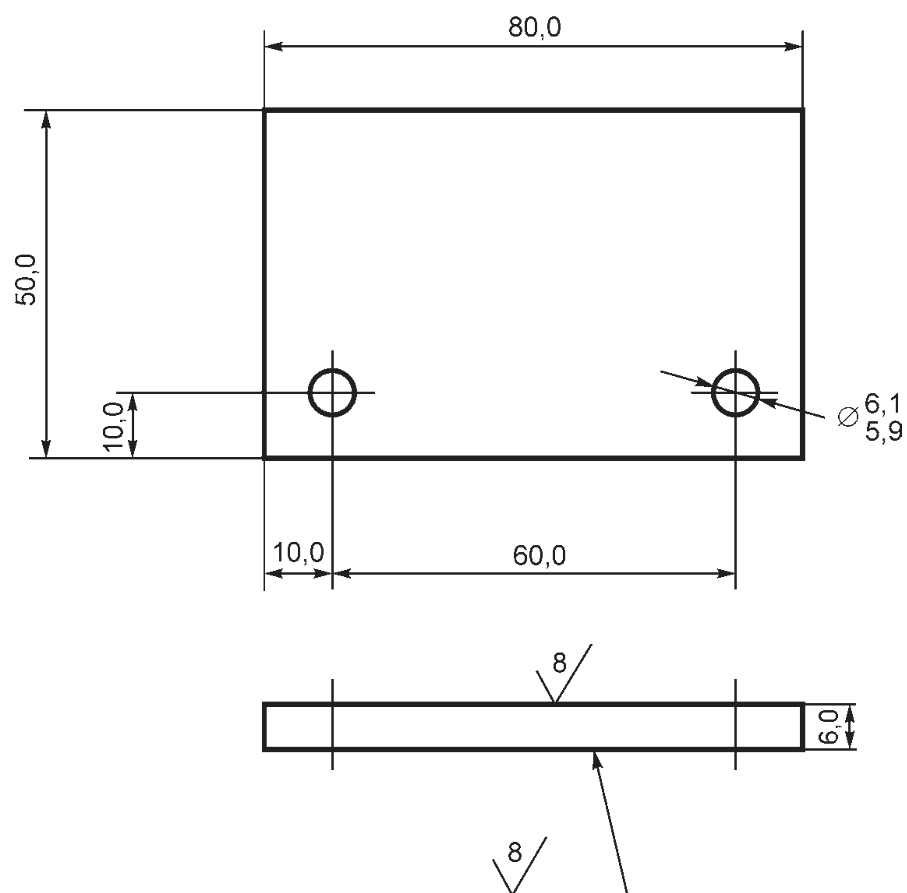
Рисунок 4 — Короткий захват
