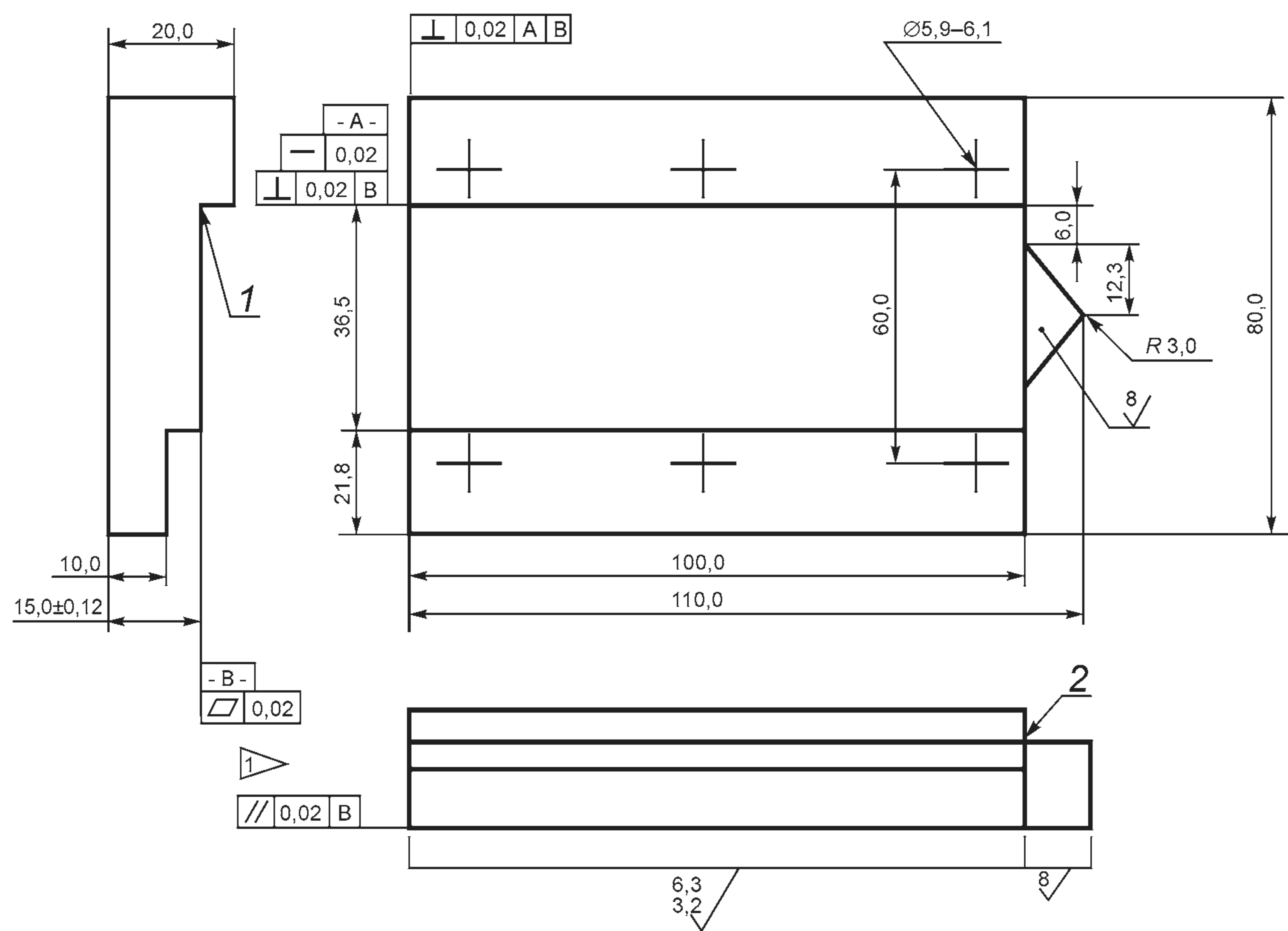
Рисунок 4 — Короткий захват
