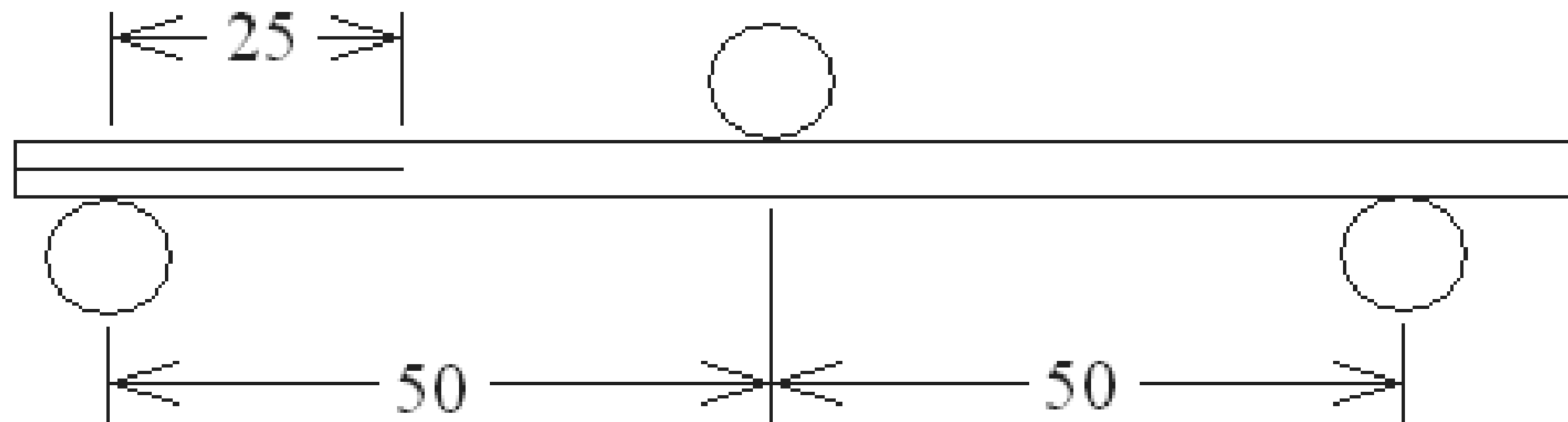
Рисунок 5 – Начальное положение образца на испытательной оснастке
