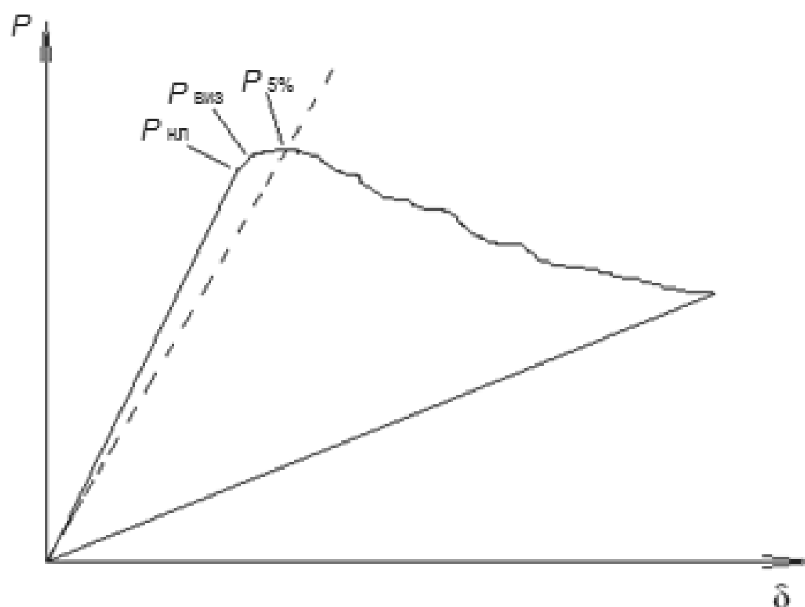
Рисунок 1 – Типовая диаграмма нагрузка – перемещение
