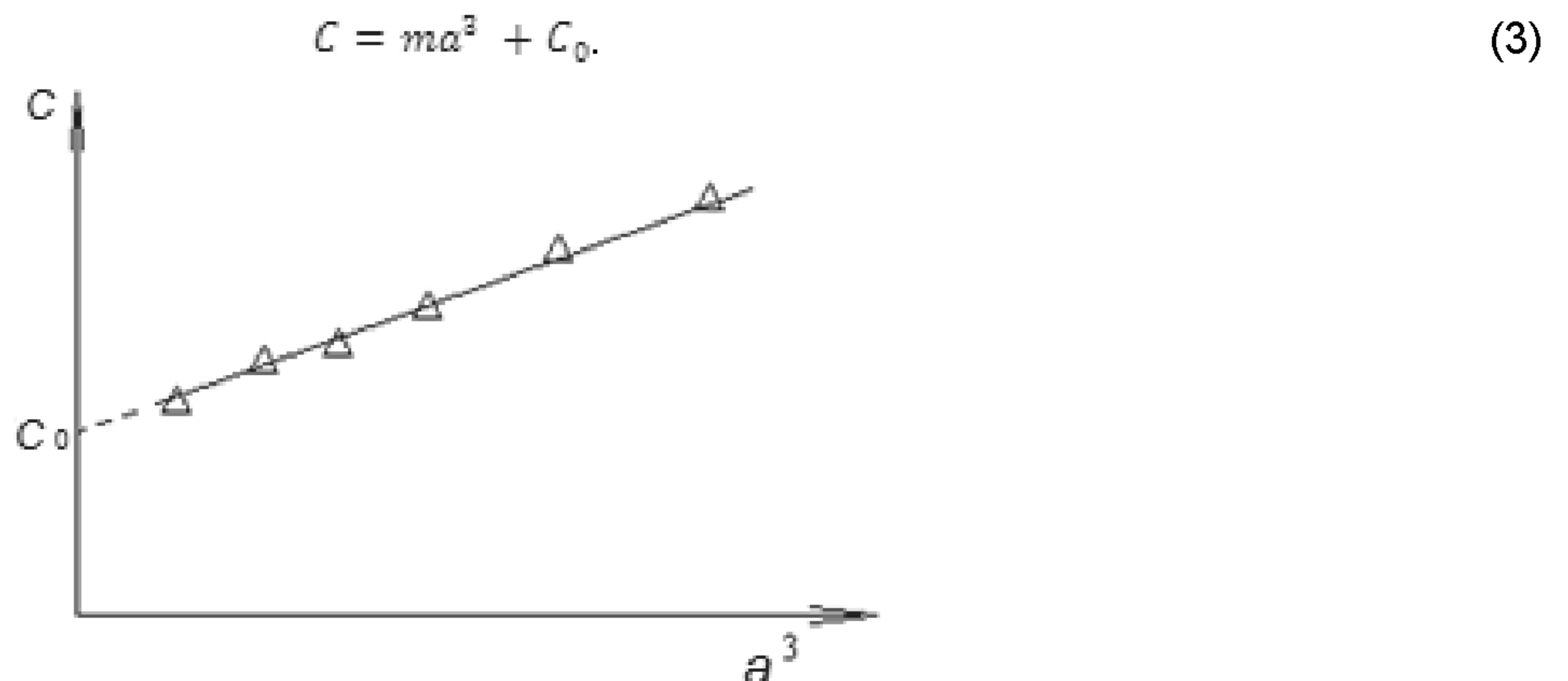
Рисунок 4 – Зависимость податливости образца от длины трещины
