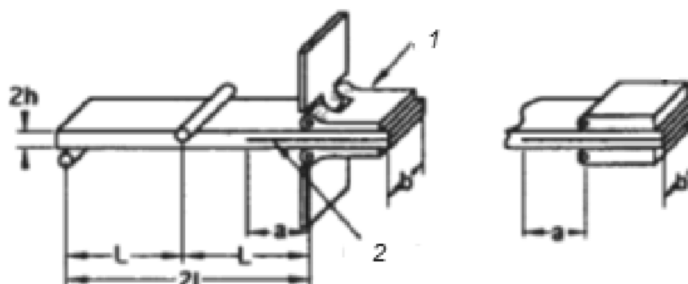
1 – шарнир; 2 – расслаивание
