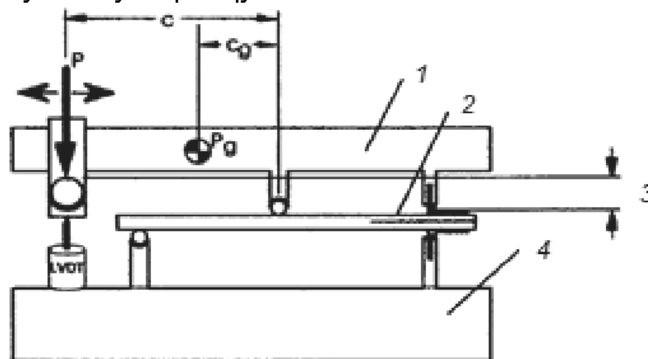
1 – рычаг; 2 – образец испытаний; 3 – погрузочная высота; 4 – основание Рисунок 1 – Оснастка для испытаний по смешанной моде нагружения I + II
