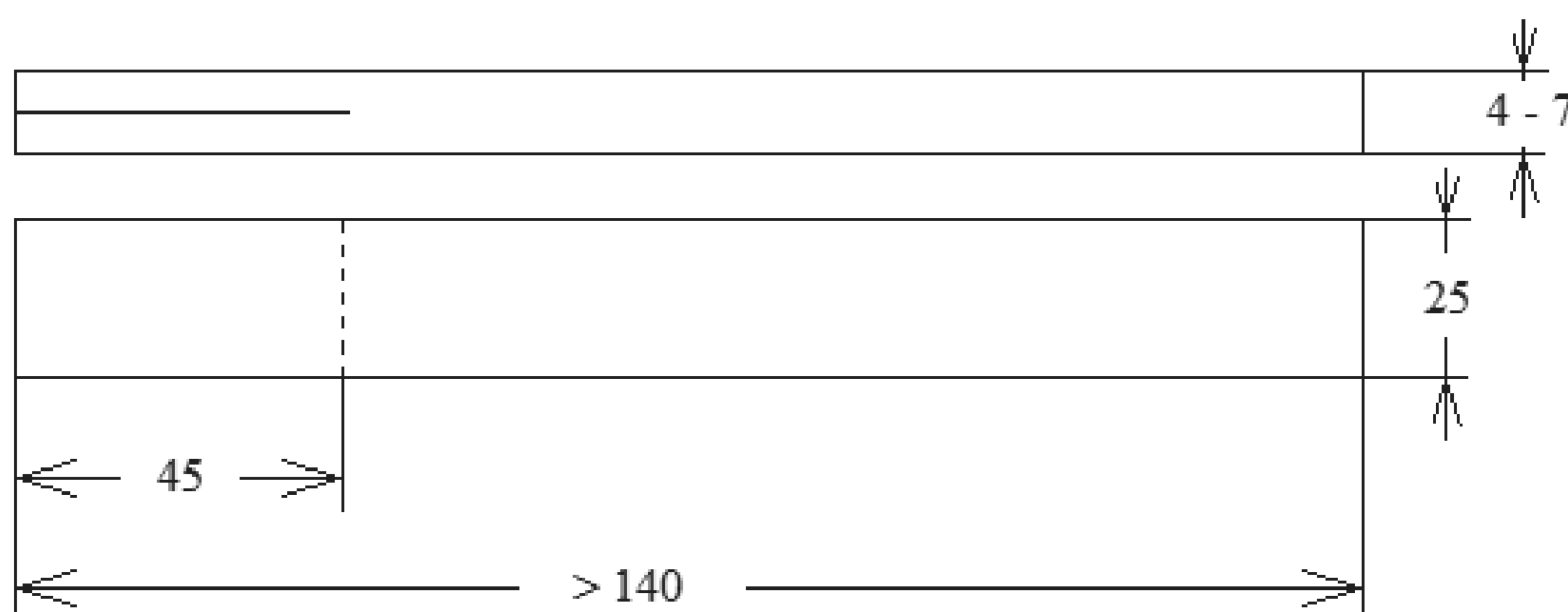
Рисунок 2 – Эскиз образца в форме двухконсольной балки
