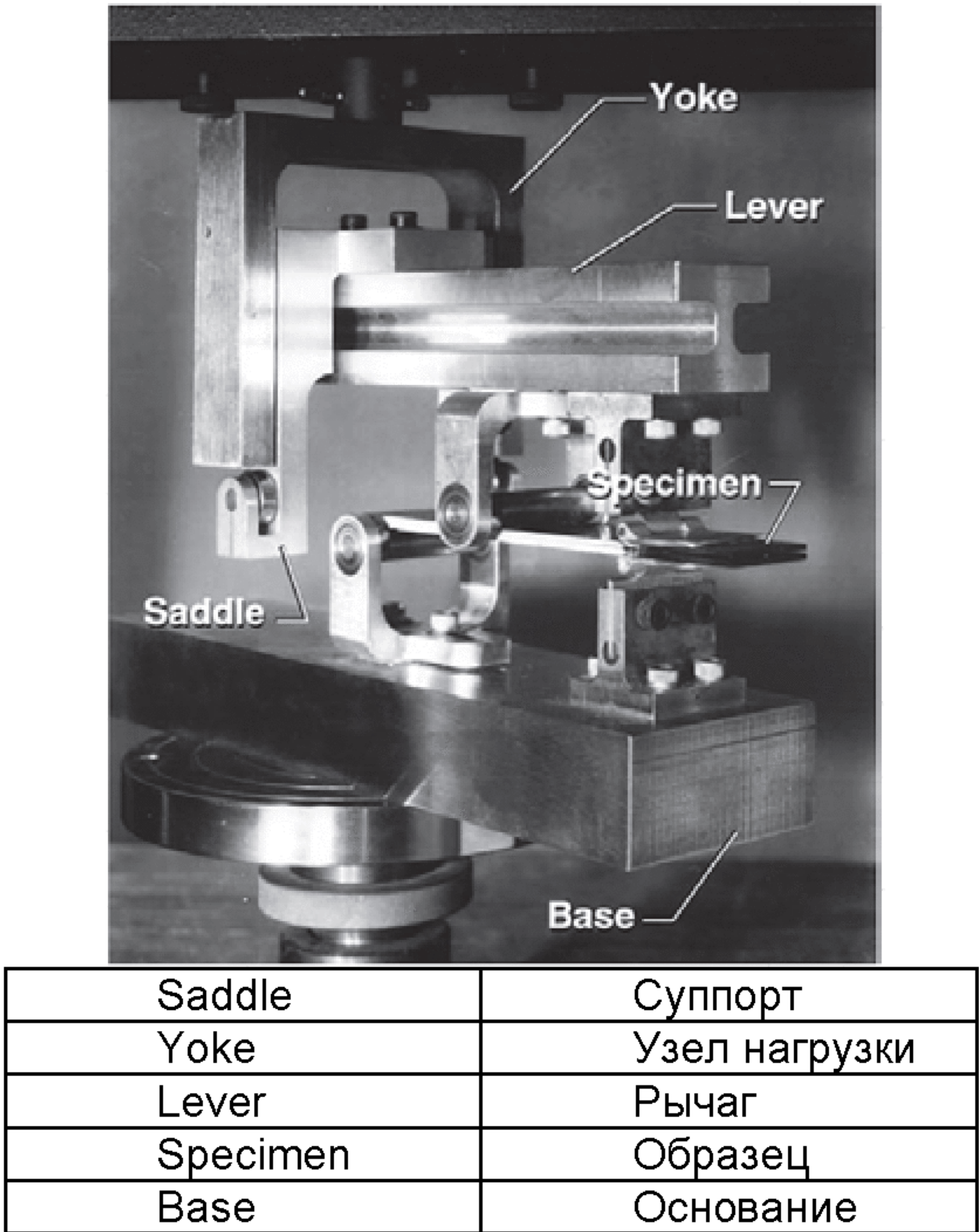
Рисунок 5 – Оснастка для по смешанной моды
