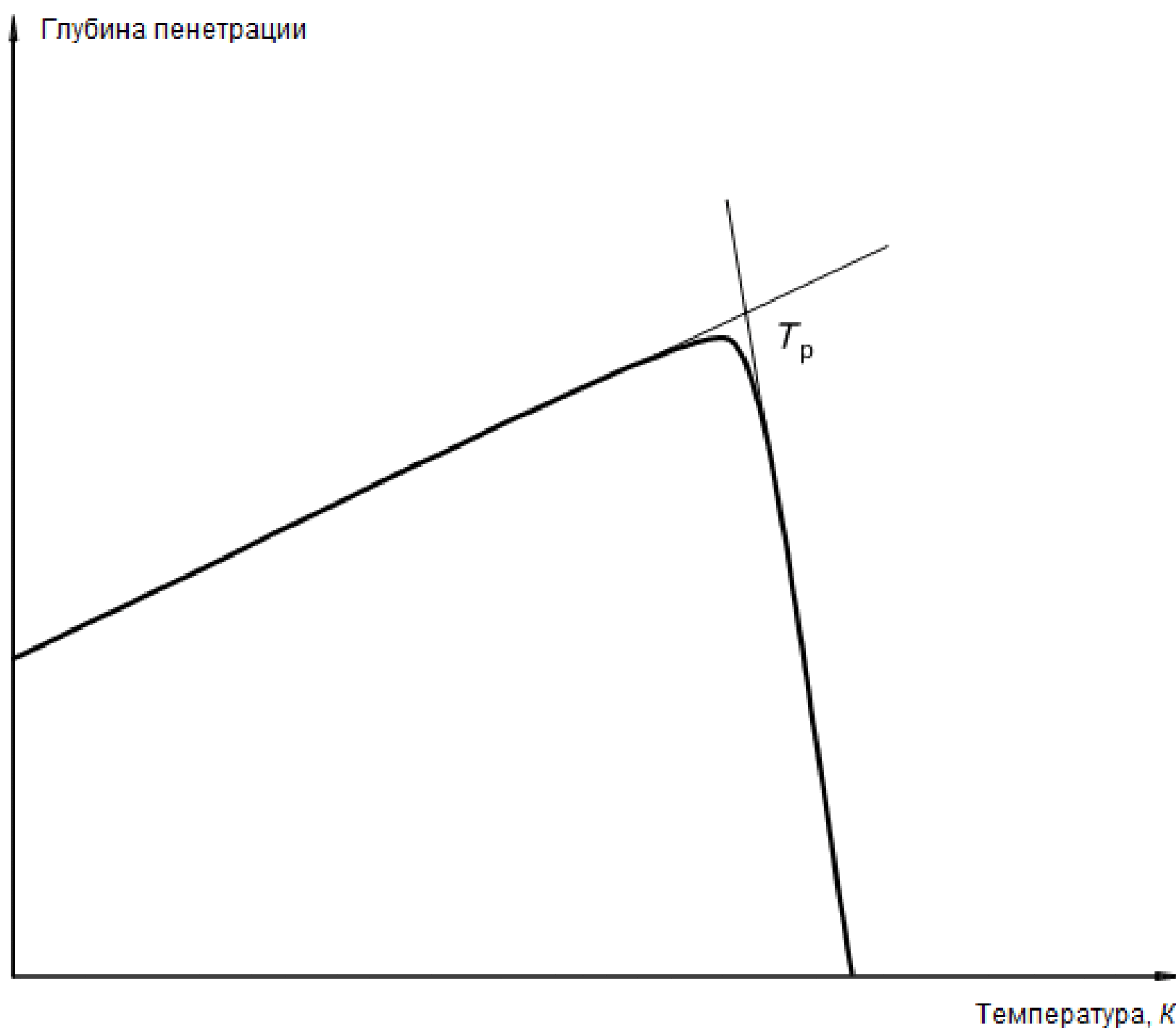
Рисунок 1 — Определение температуры пенетрации
