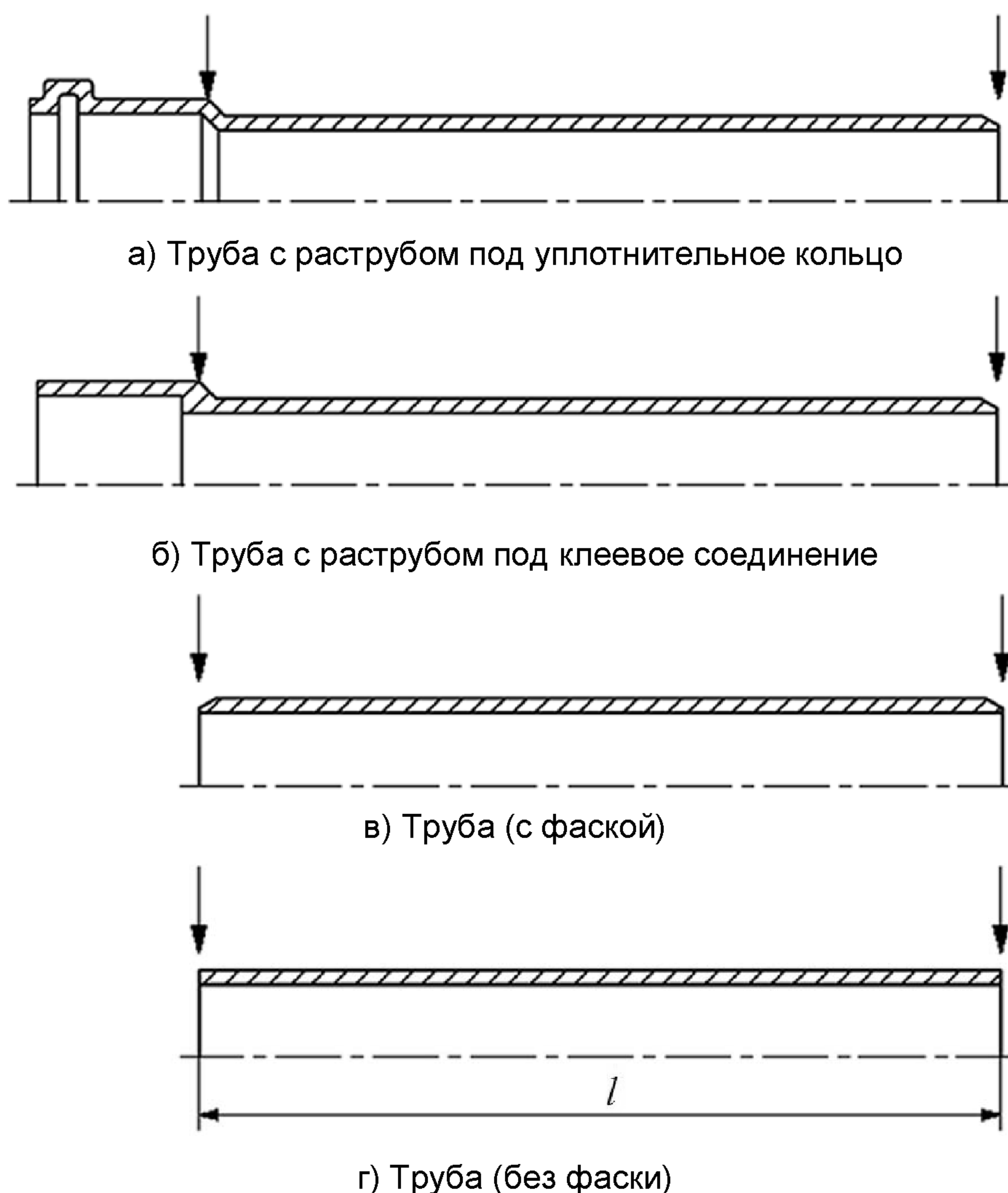
Рисунок 1 – Эффективная длина труб
