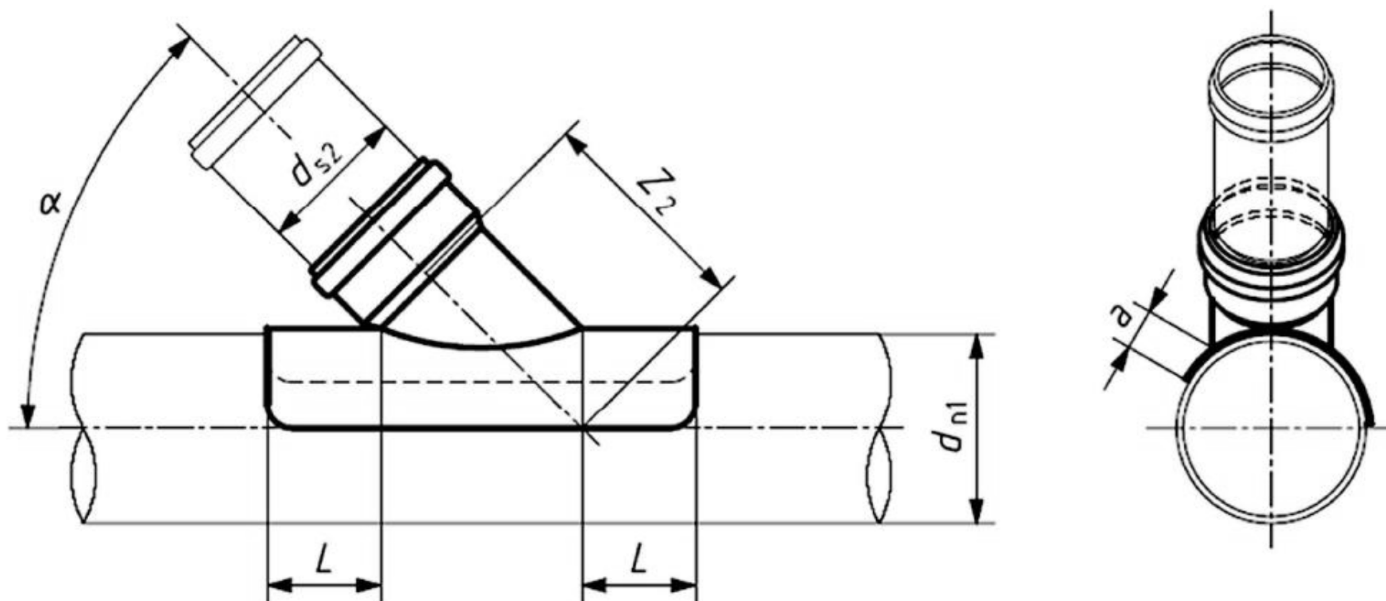
Рисунок 10 – Седловой отвод
