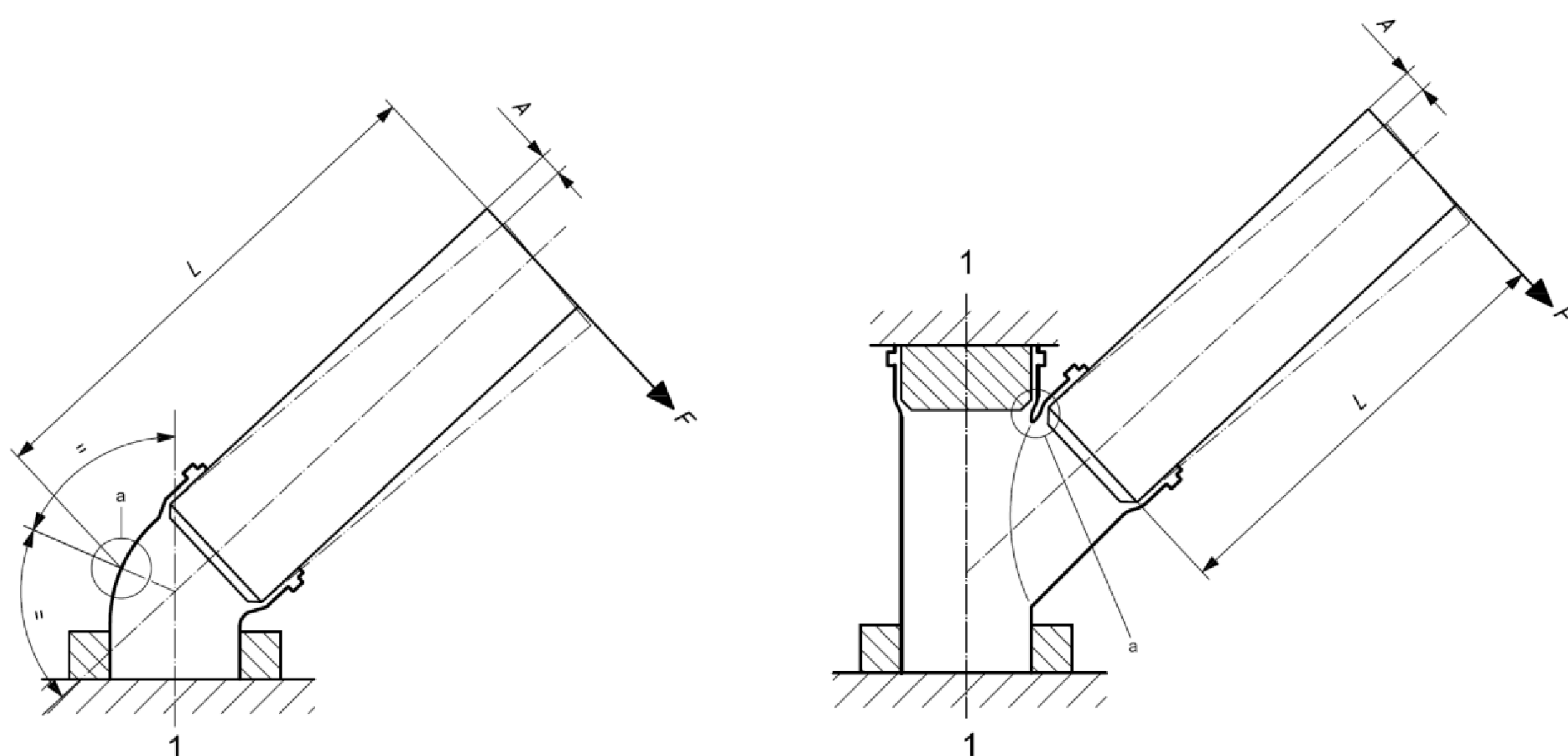
1 – фиксирующие элементы; а – зона возможного разрушения
