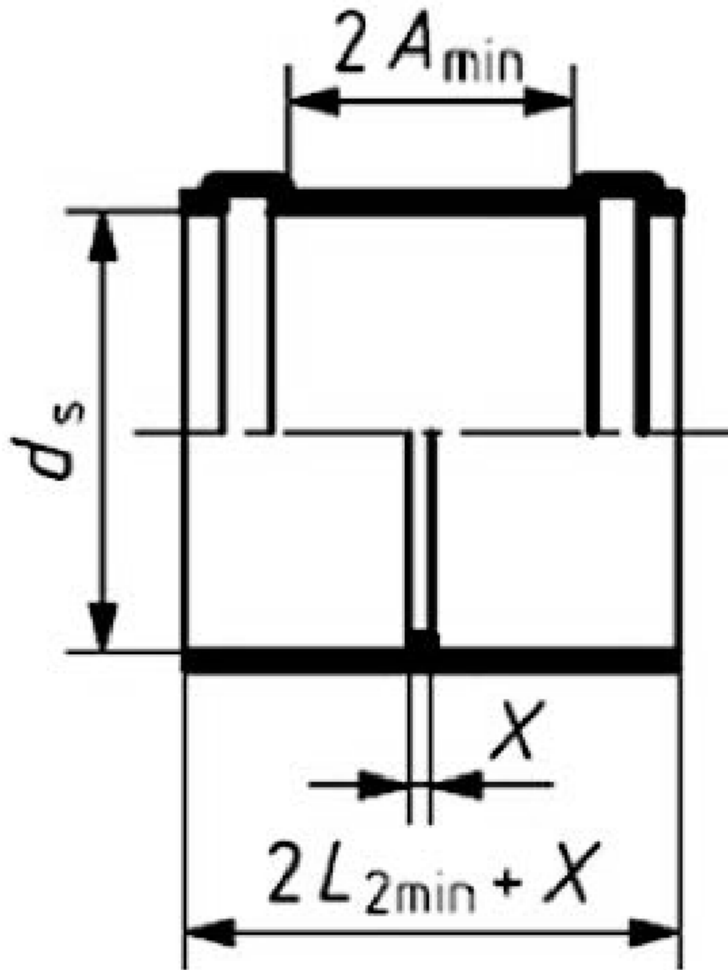
Рисунок 7 – Муфта
