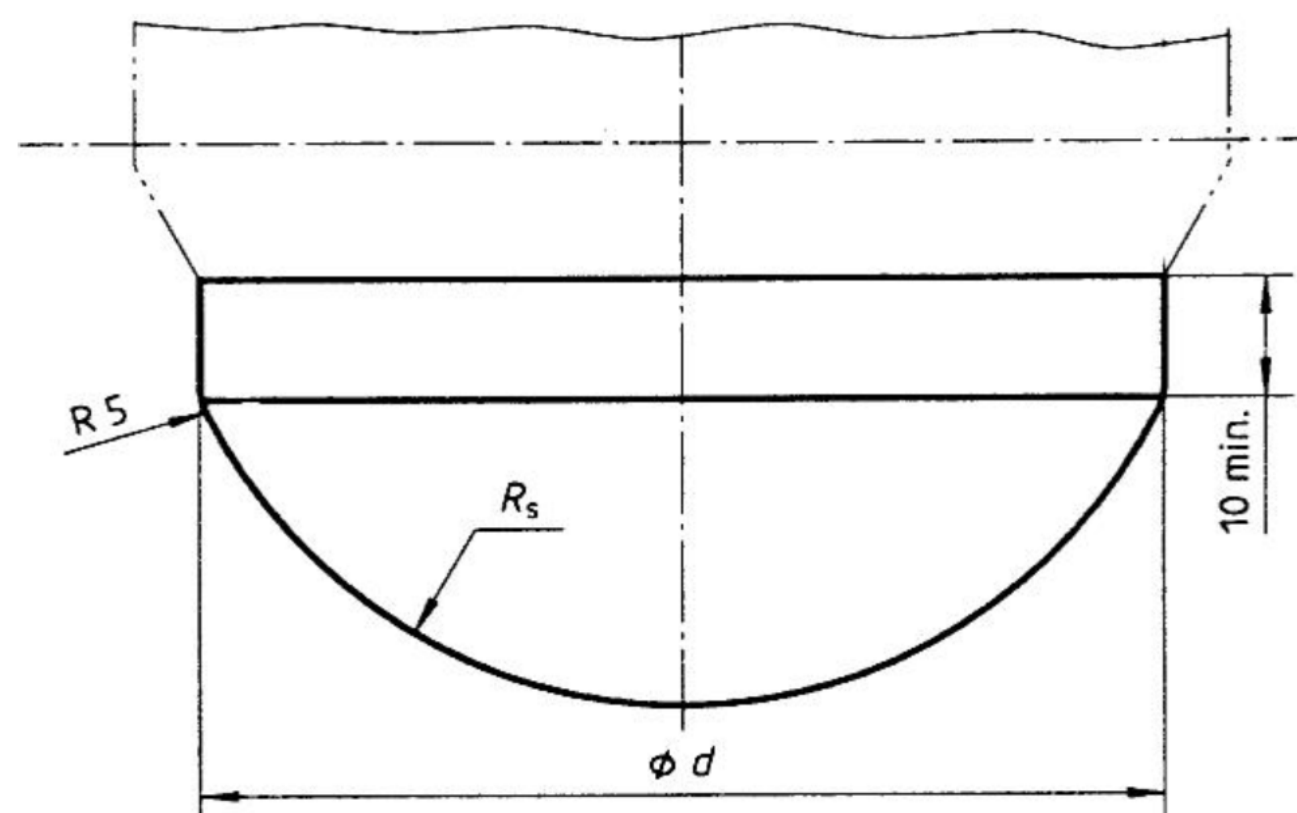
Рисунок 12 – Боек падающего груза
