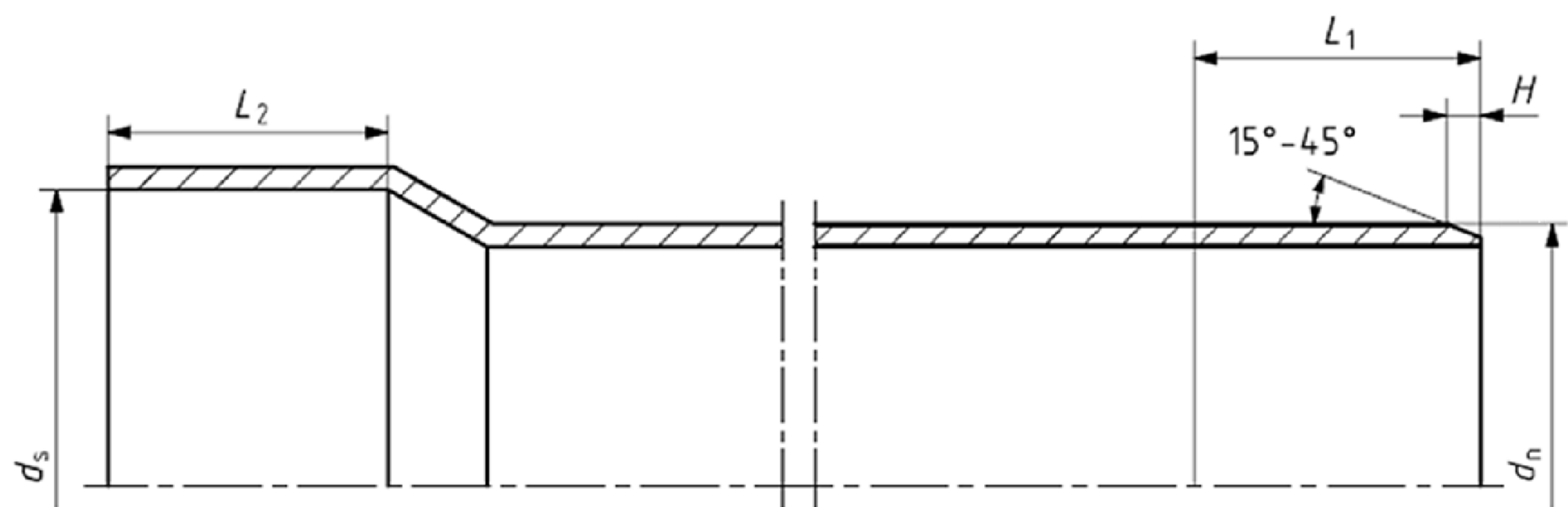
d_s – внутренний диаметр раструба; L_1 – длина трубного конца; L_2 – длина раструба
