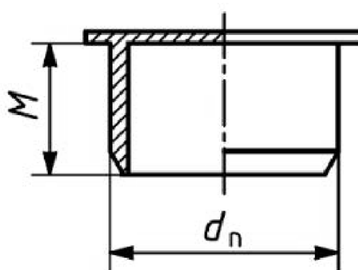
Рисунок 11 – Заглушка
