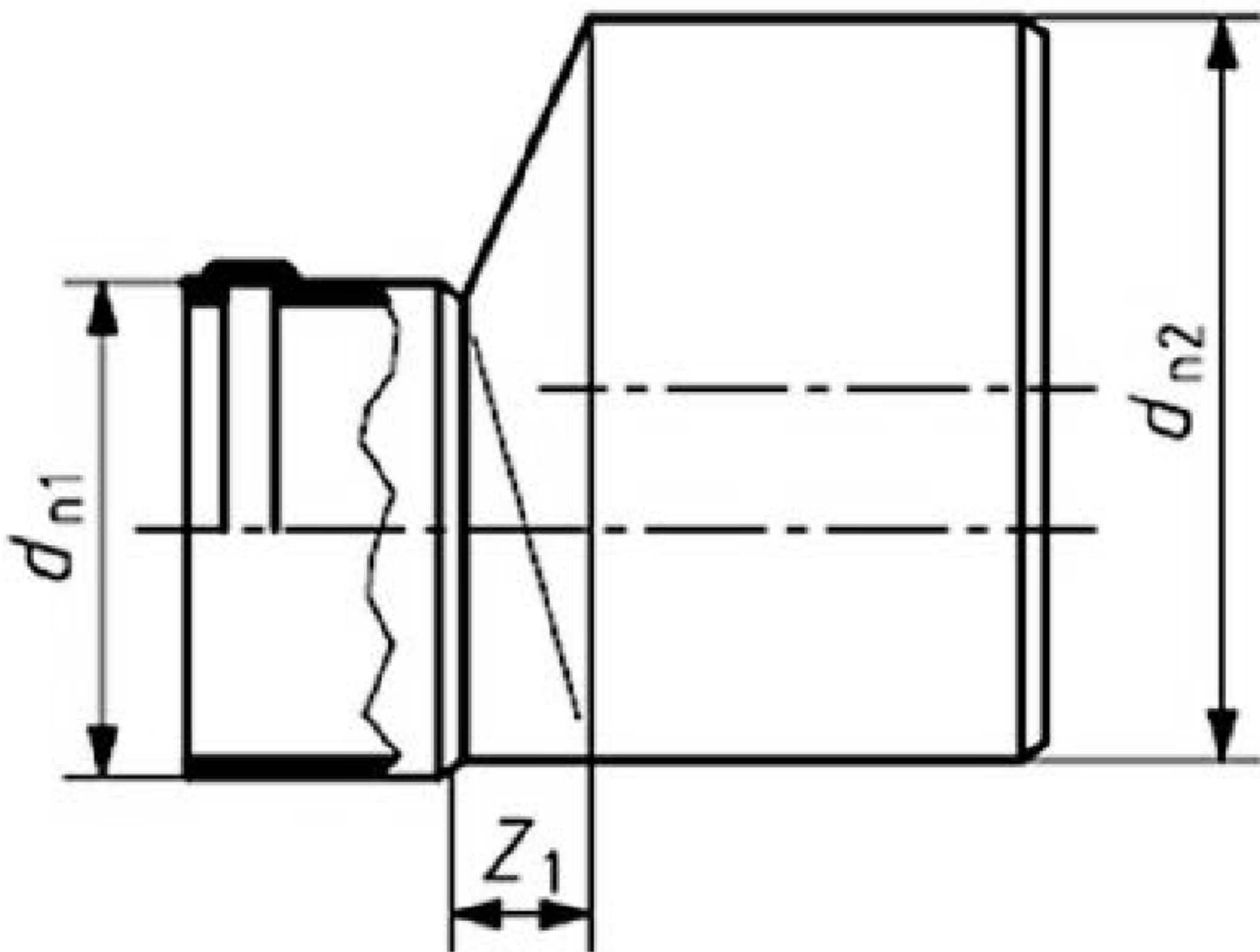
Рисунок 8 – Патрубок переходной
