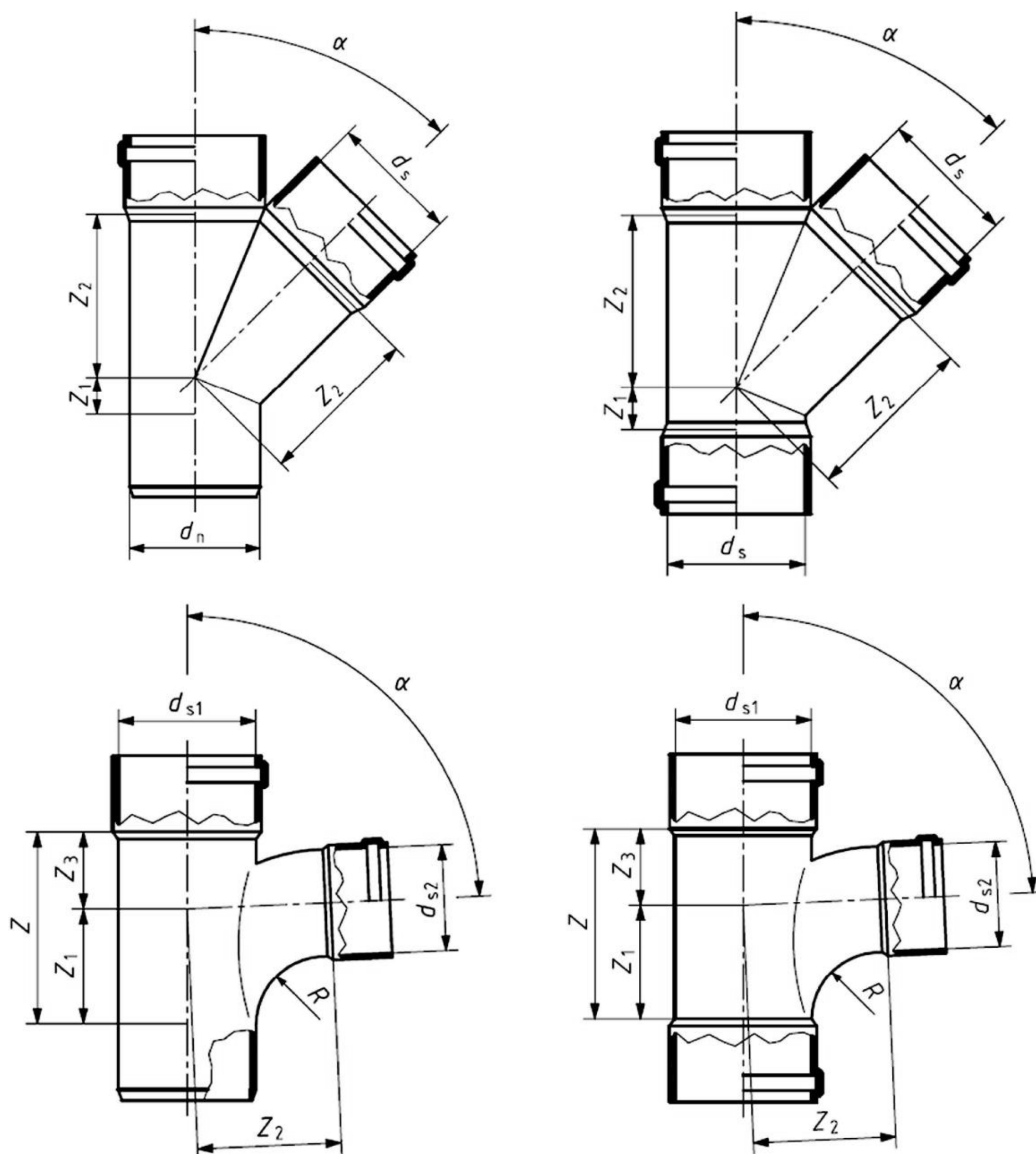
Рисунок 9 – Тройник
