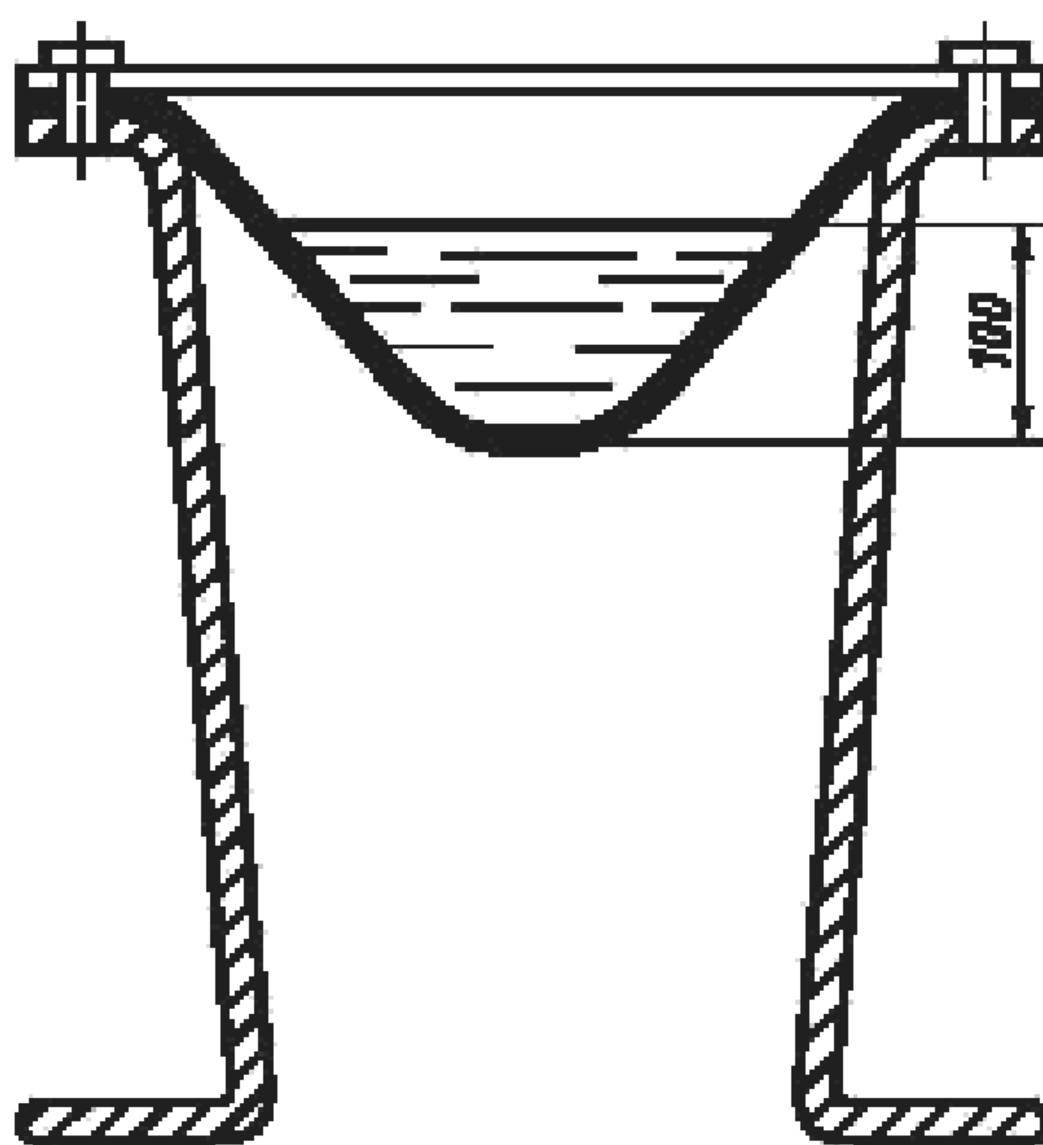
Рисунок 4 — Приспособление для определения водопроницаемости методом кошеля
