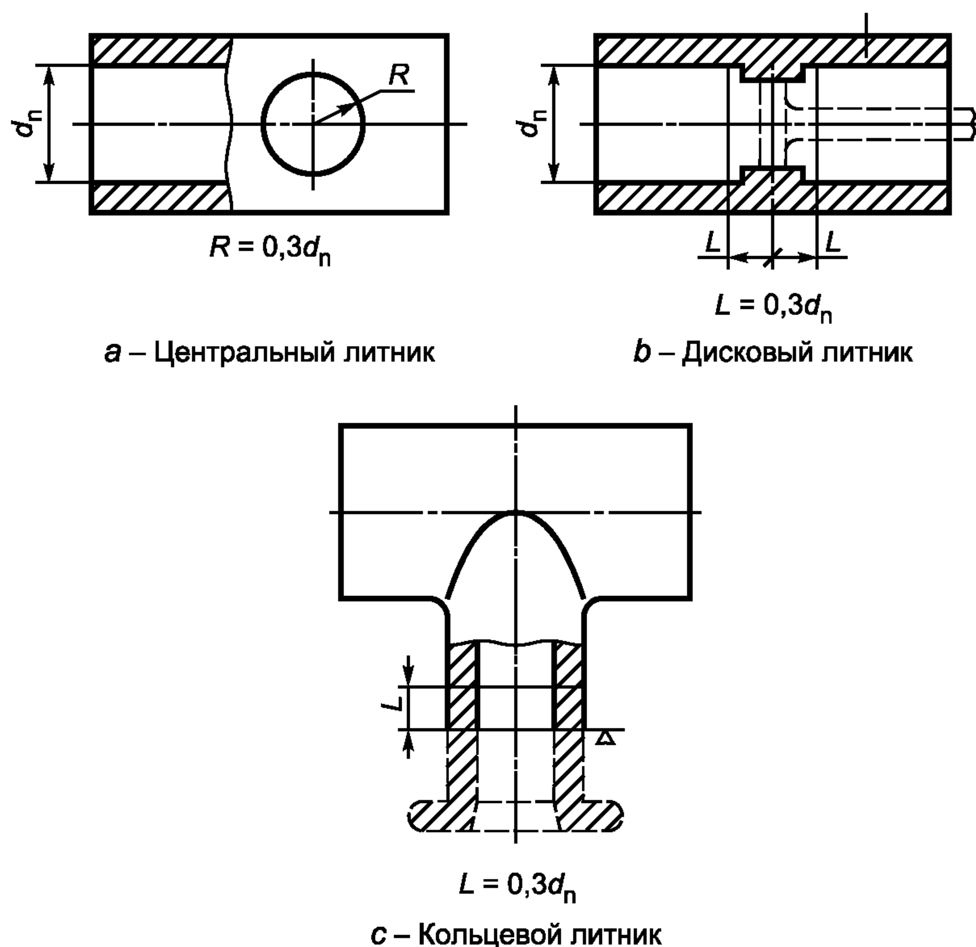
Рисунок 1 — Литниковые системы
