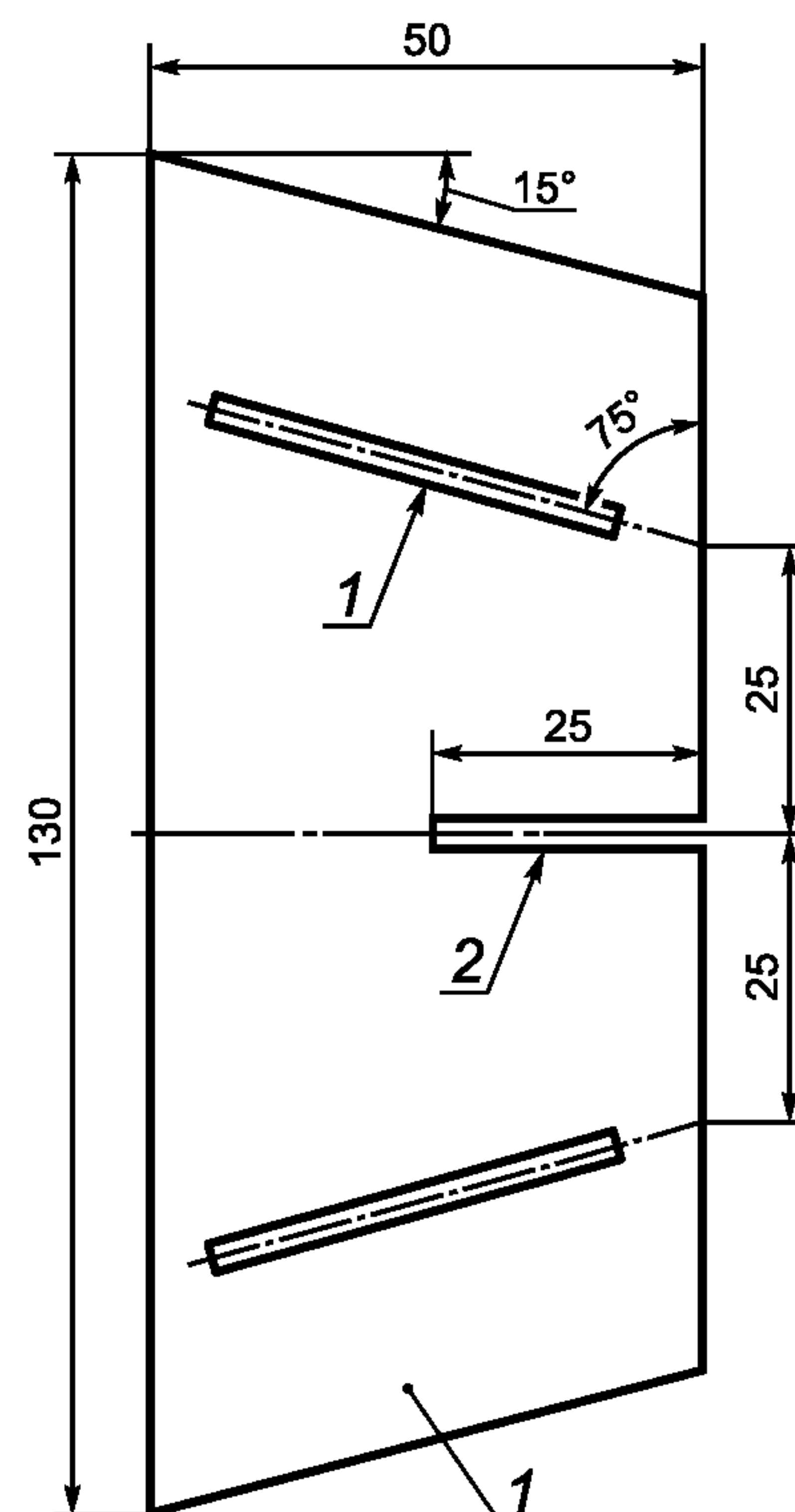
1 — маркировка для зажима; 2 — надрез
