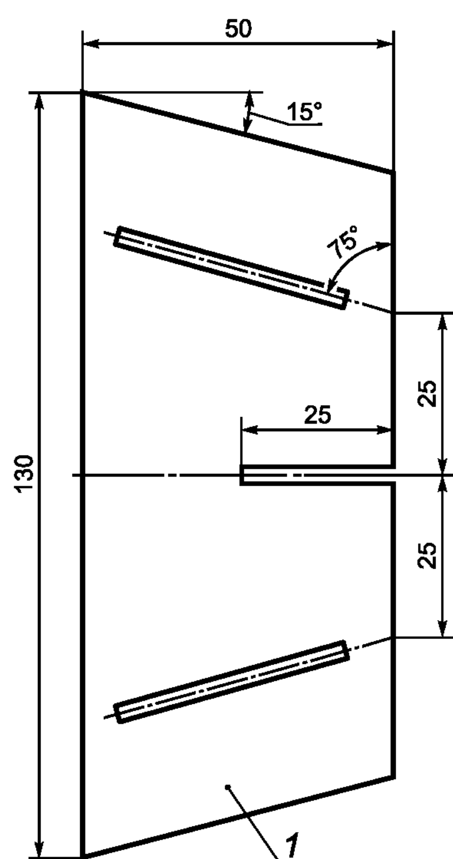
1 — шаблон толщиной от 2 мм до 3 мм
