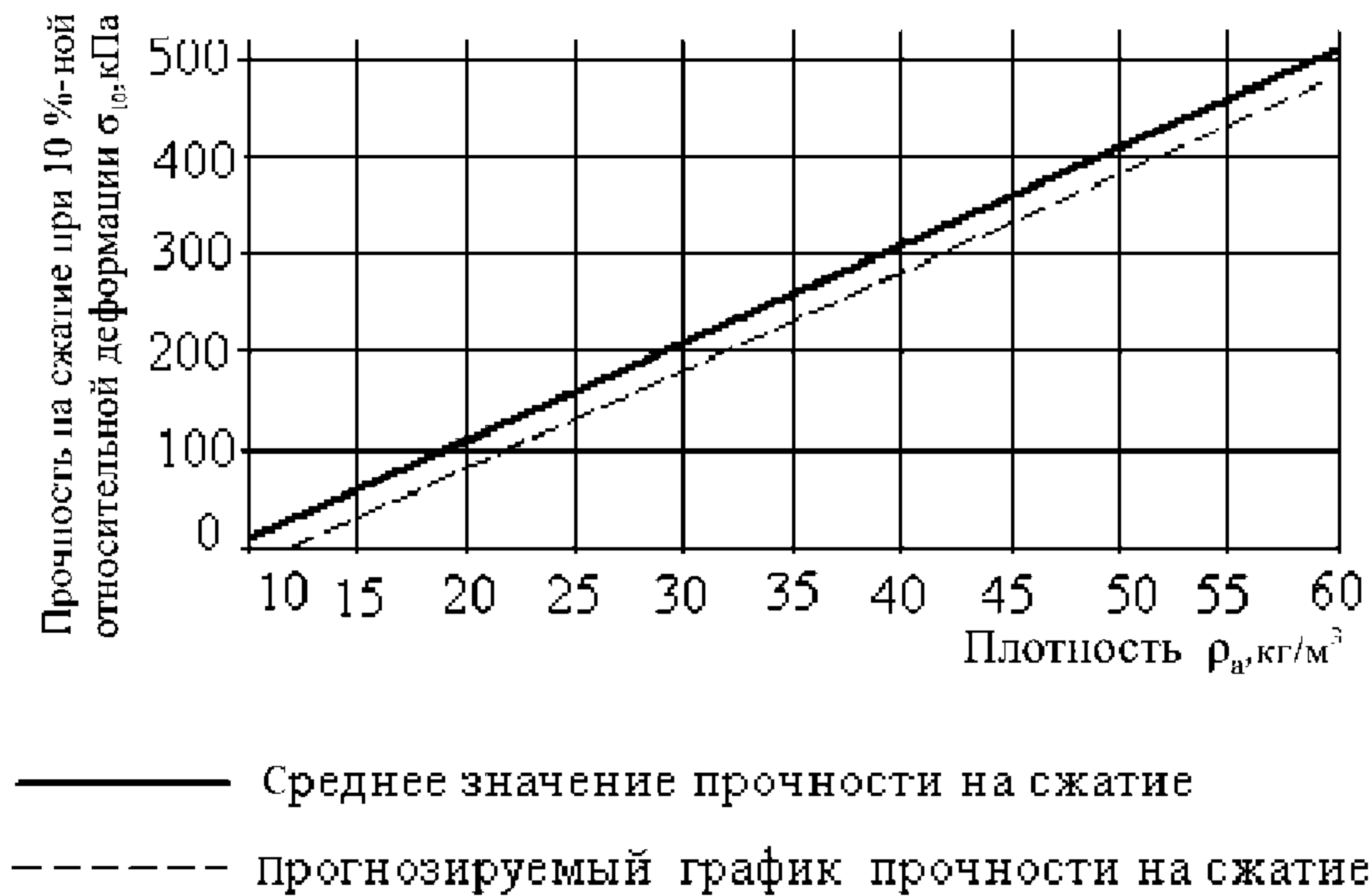
Рисунок В.1 – Зависимость прочности на сжатие при 10 %-ной относительной деформации от плотности (косвенный метод); 1– а = 0,90; n = 495
