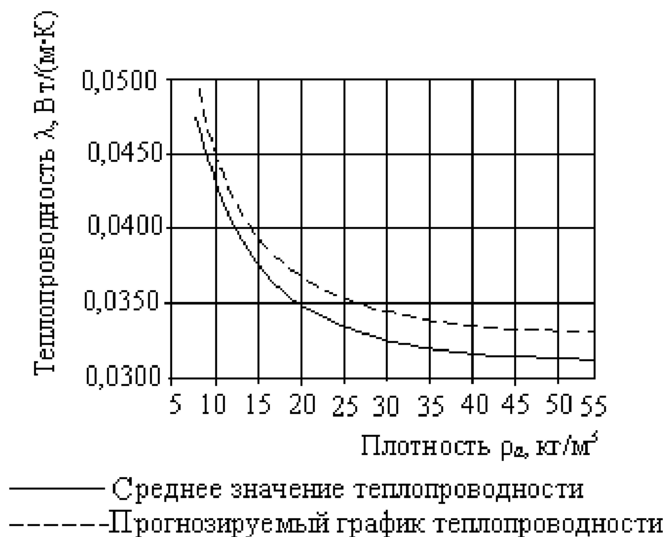
Рисунок В.2 – Зависимость теплопроводности от плотности (косвенный метод) [толщина материала 50 мм; средняя температура 10 °С; (1 – α) = 0,90; n = 3873]
