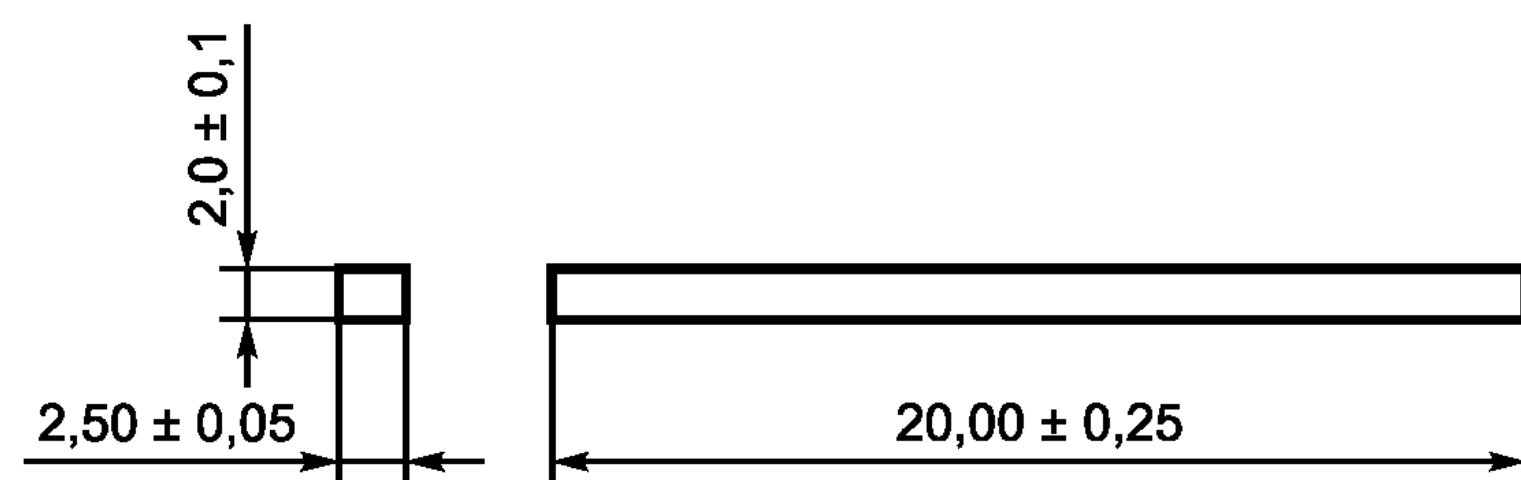
Рисунок 4 — Размеры образца для испытаний
