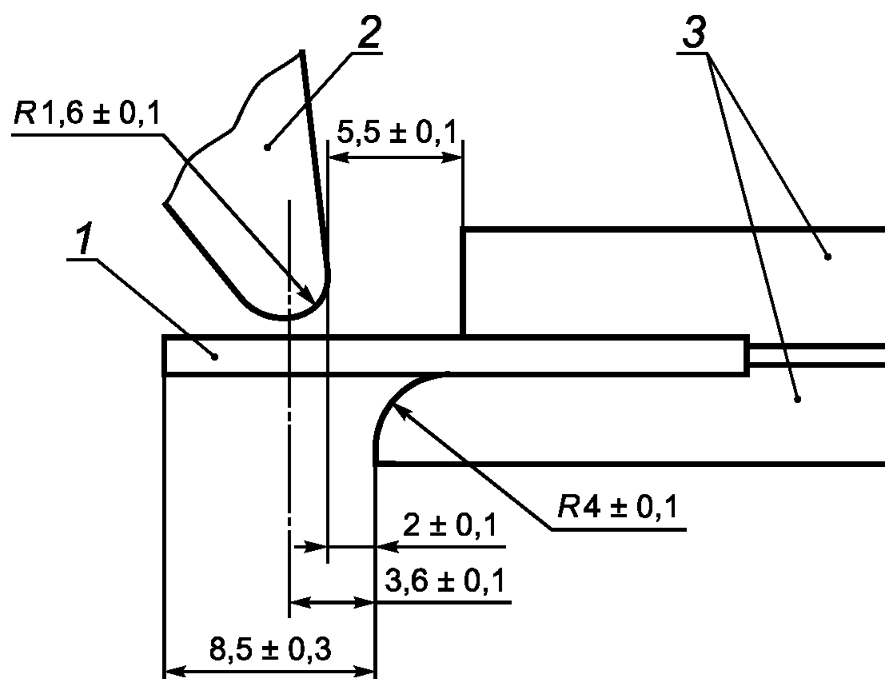
1 — испытываемый образец; 2 — зажимное приспособление; 3 — ударный боек
