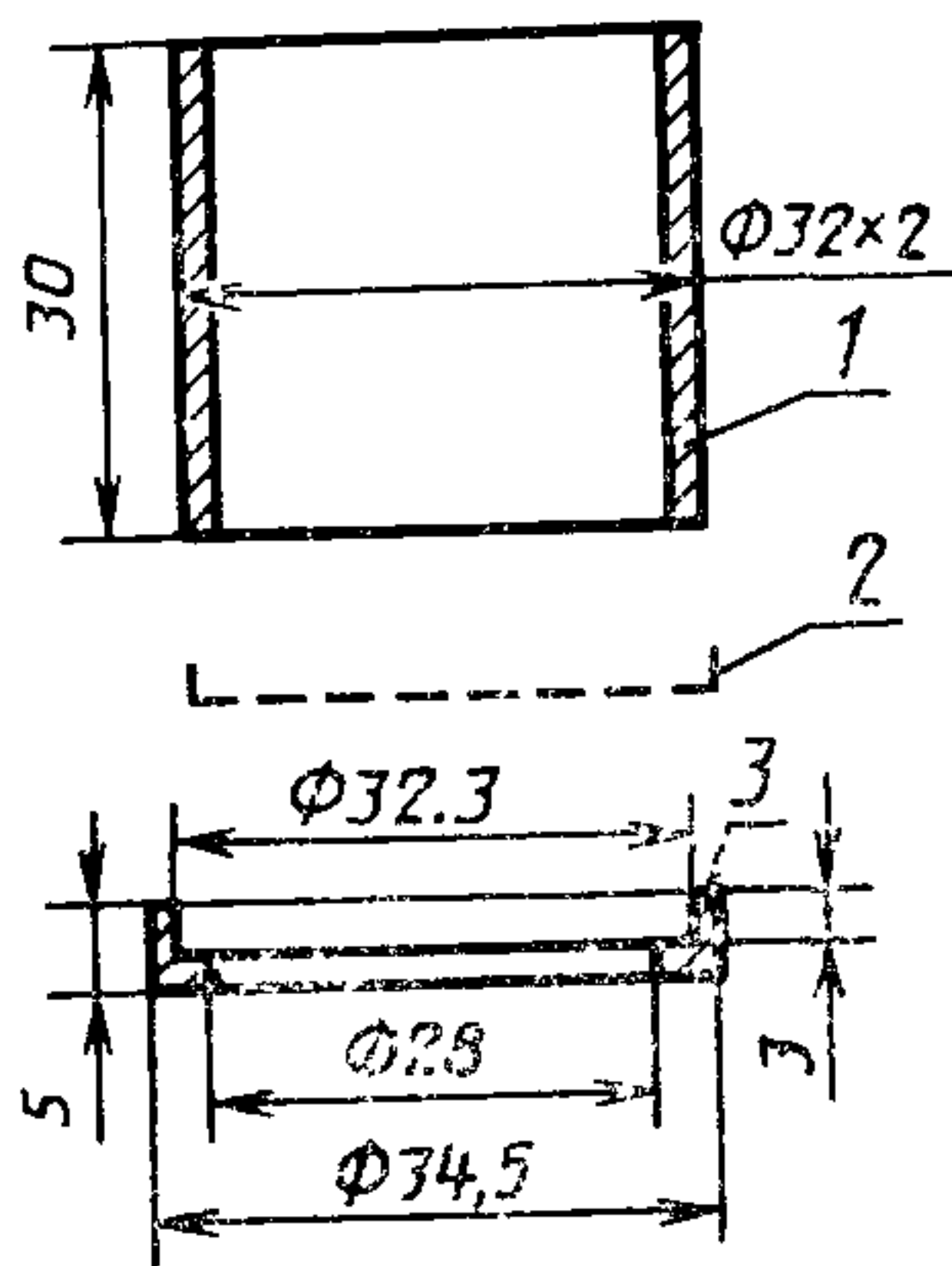
Фильтрующее устройство
