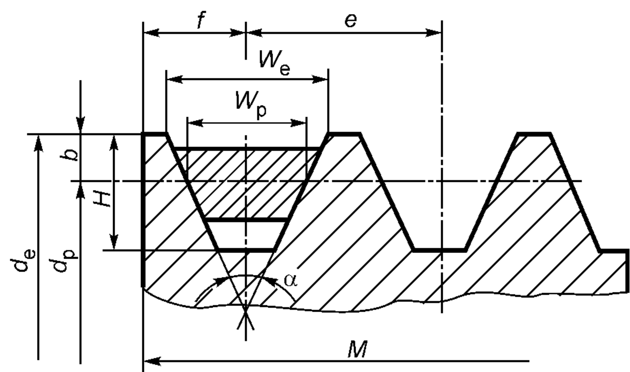
d_p — расчетный диаметр шкива; d_e — наружный диаметр шкива; W_p — расчетная ширина канавки шкива; W_e — ширина канавки по наружному диаметру; H — глубина канавки; b — глубина канавки над расчетной шириной; \alpha — угол канавки шкива; f — расстояние между осью крайней канавки и торцом шкива; e — расстояние между осями канавок (шаг); M — ширина шкива
