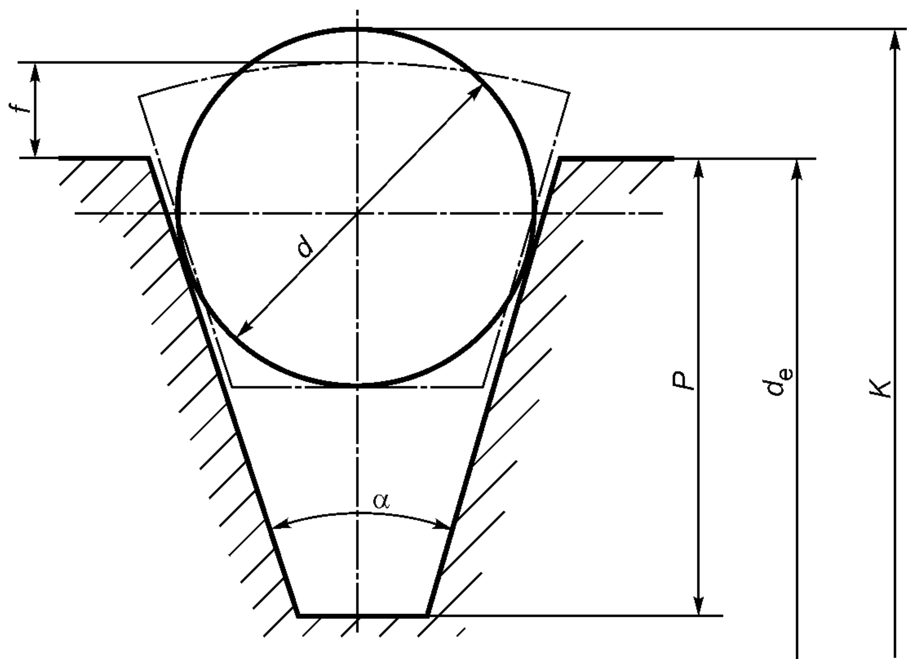
\alpha — угол канавки шкива; d_e ( \sim d_0 ) — эффективный (наружный) диаметр шкива; d — диаметр измерительного ролика или шара; P — глубина канавки; f — расстояние от эффективного (наружного) диаметра до верхнего основания ремня; K — расстояние между внешними касательными плоскостями к роликам, расположенными параллельно оси шкива, или шарами
