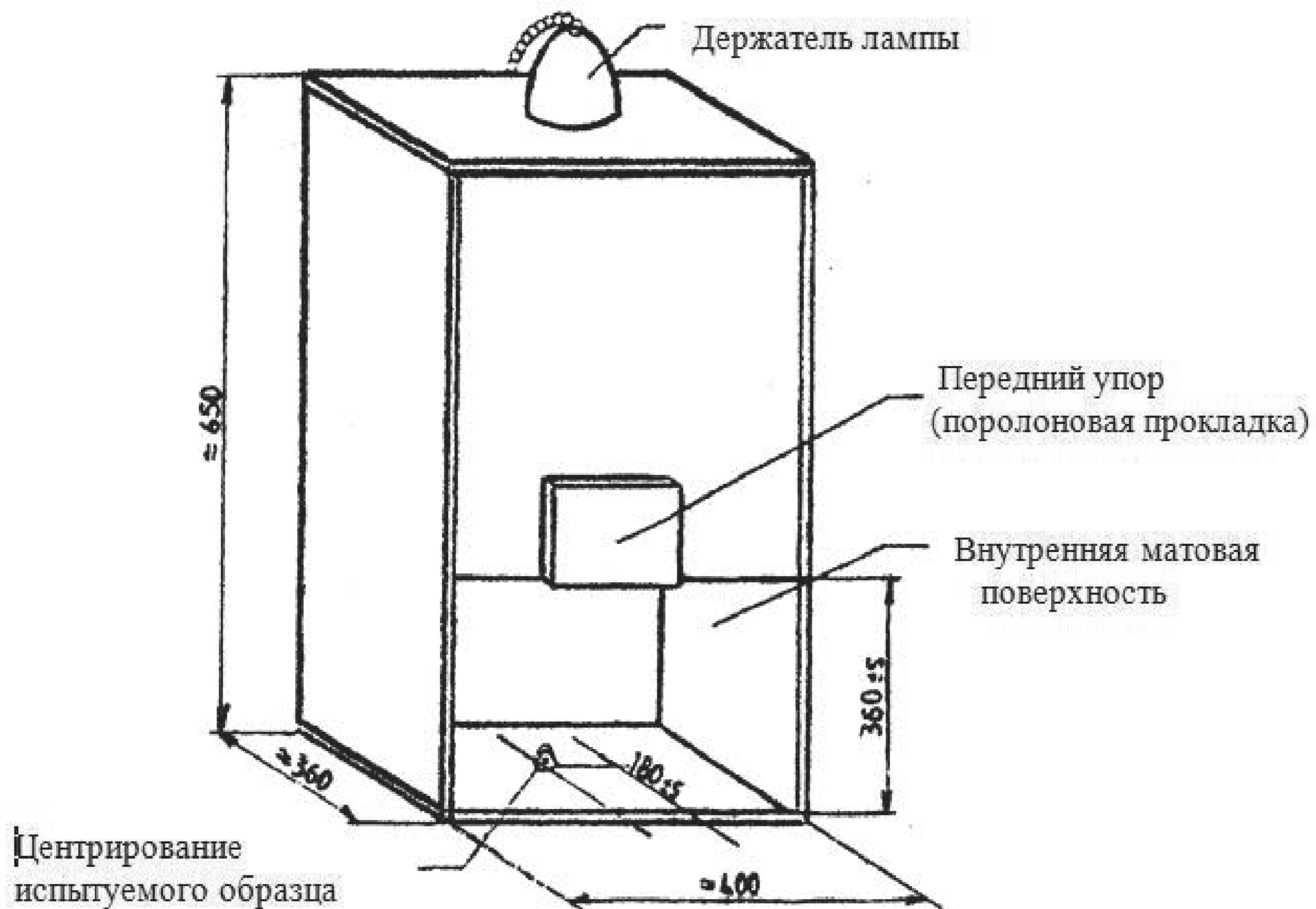
Рисунок Е.3 – Пример смотровой камеры
