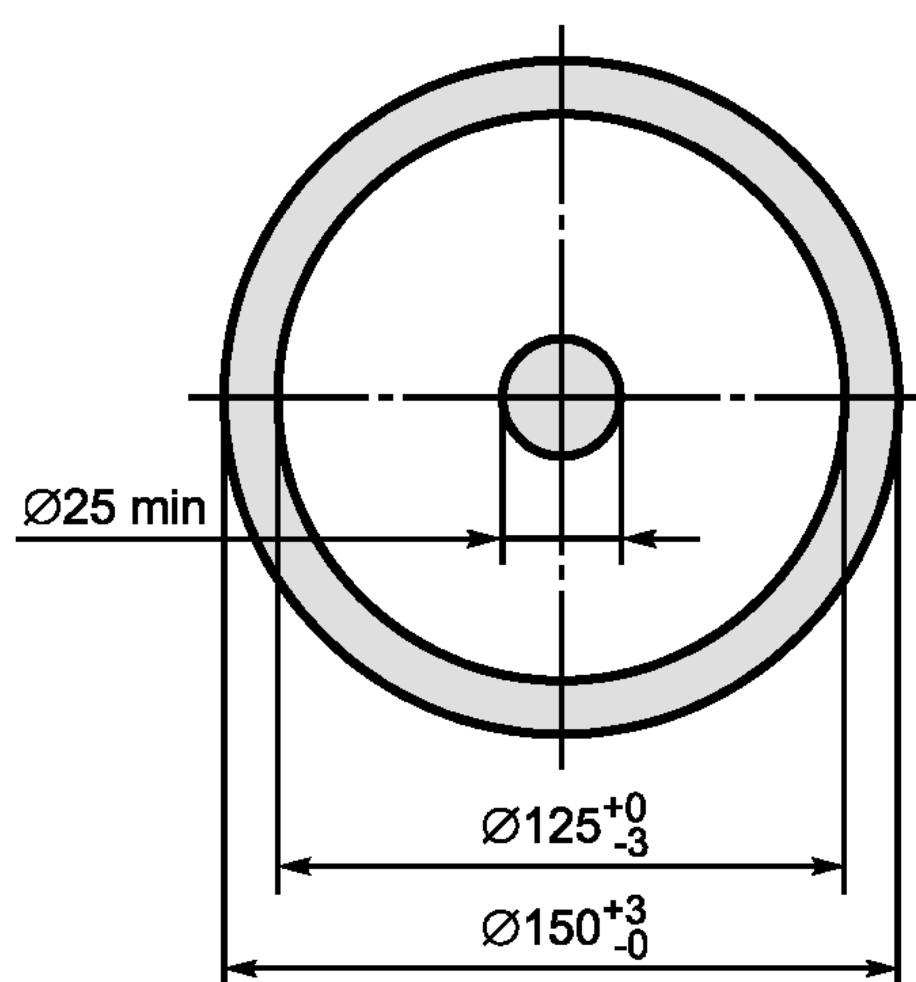
Рисунок В.2 — Шаблон
