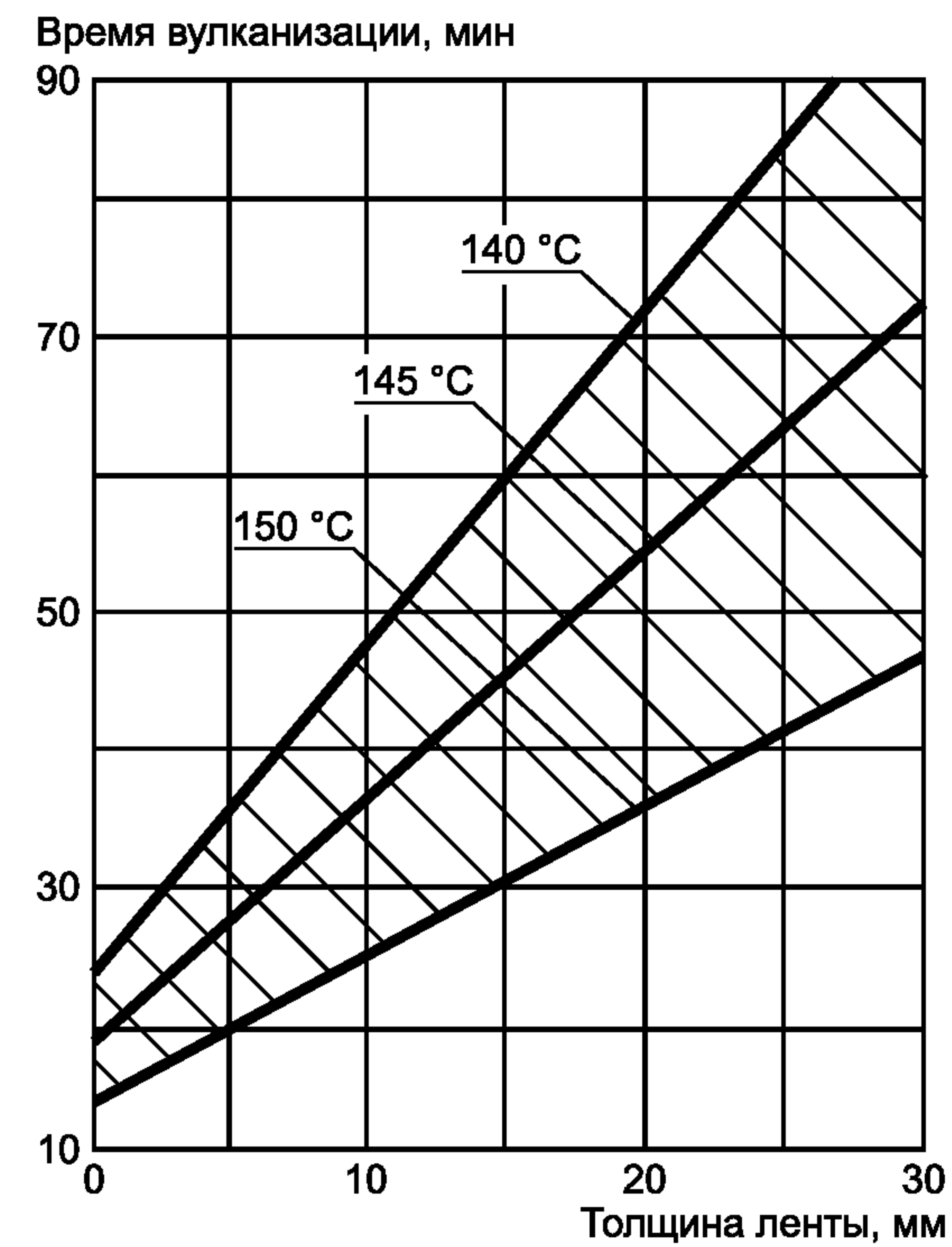
Рисунок Б.3 — Режим вулканизации стыка ленты
