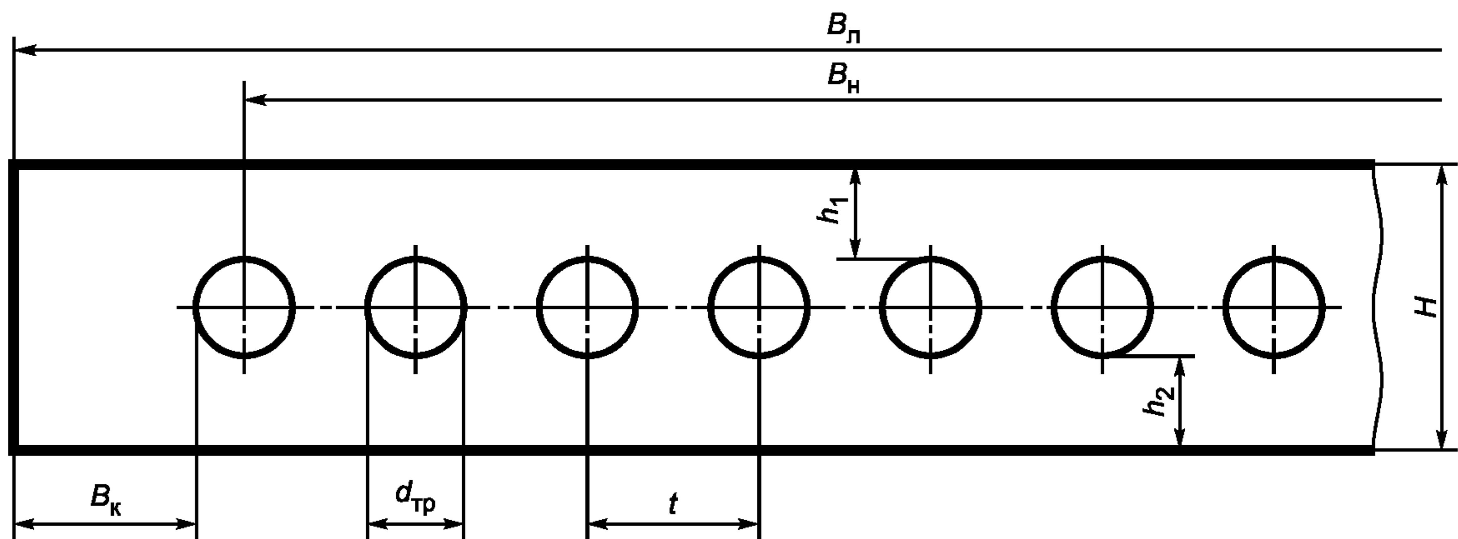
а — Бестканевая конструкция (РТЛ)
