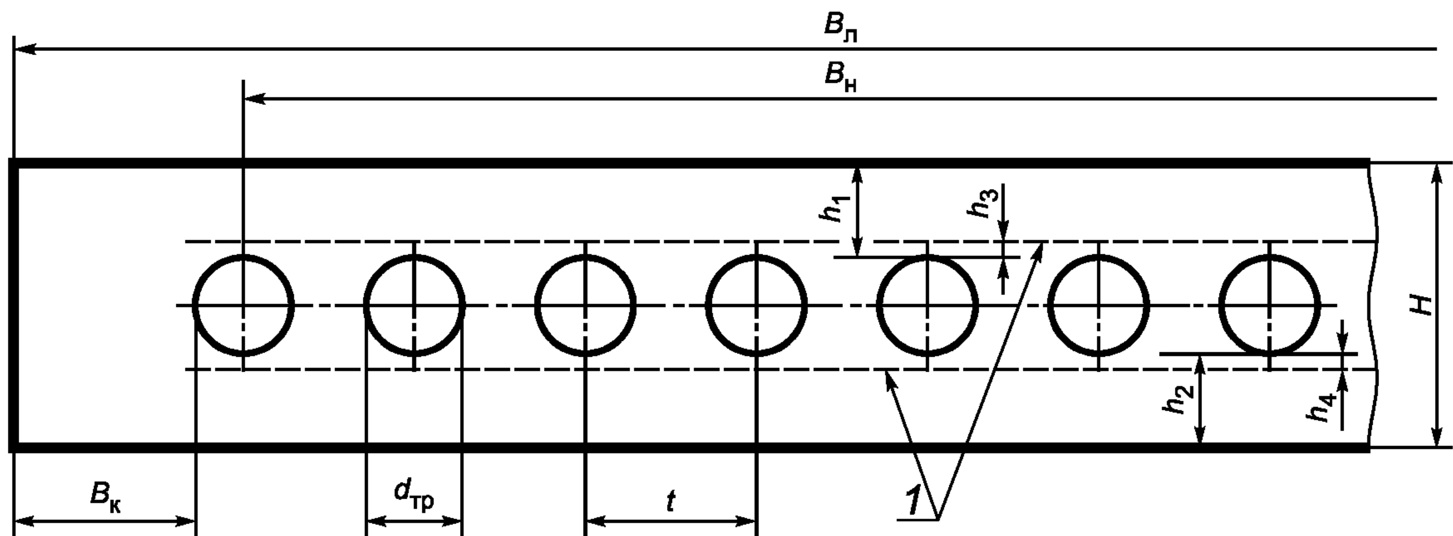
в — С двумя защитными тканевыми прокладками (2РТЛ)
