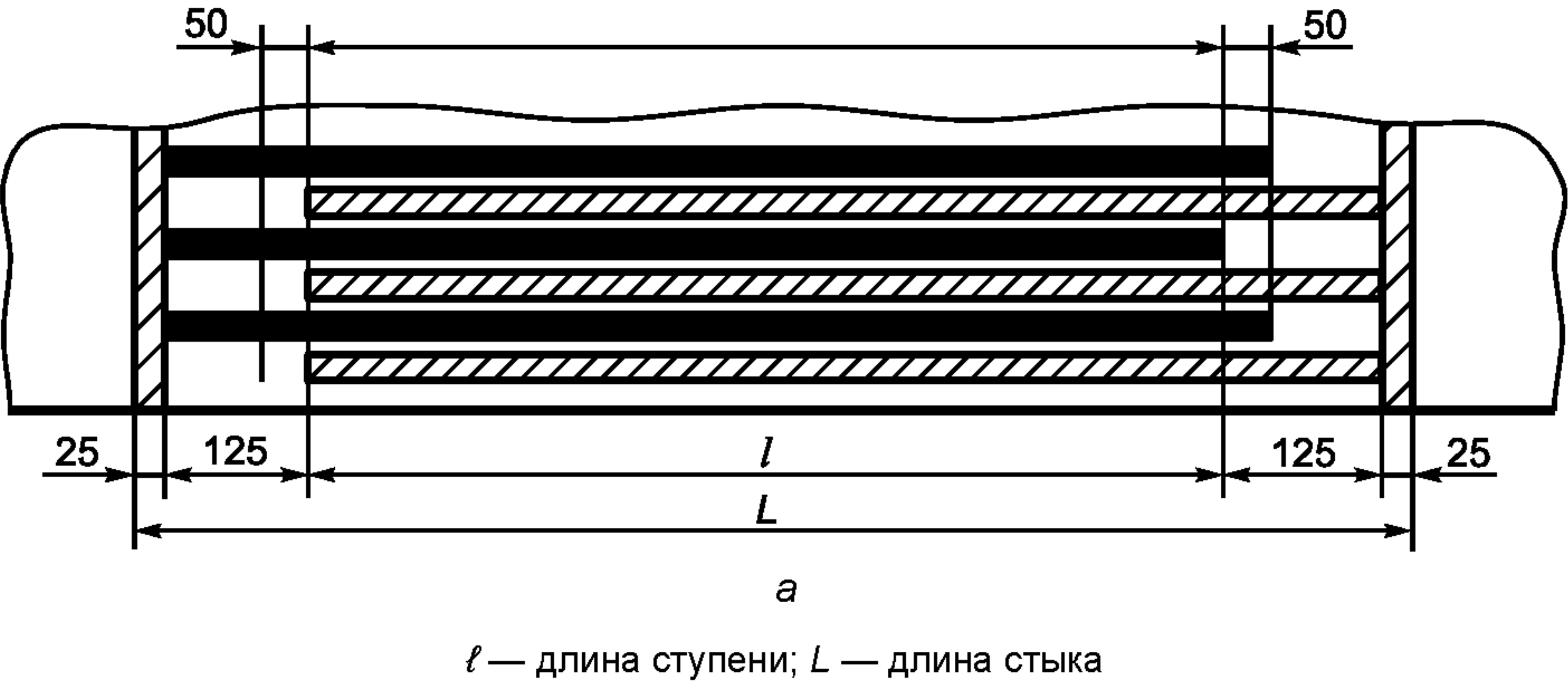
Рисунок Б.1 — Одноступенчатые схемы стыковки
