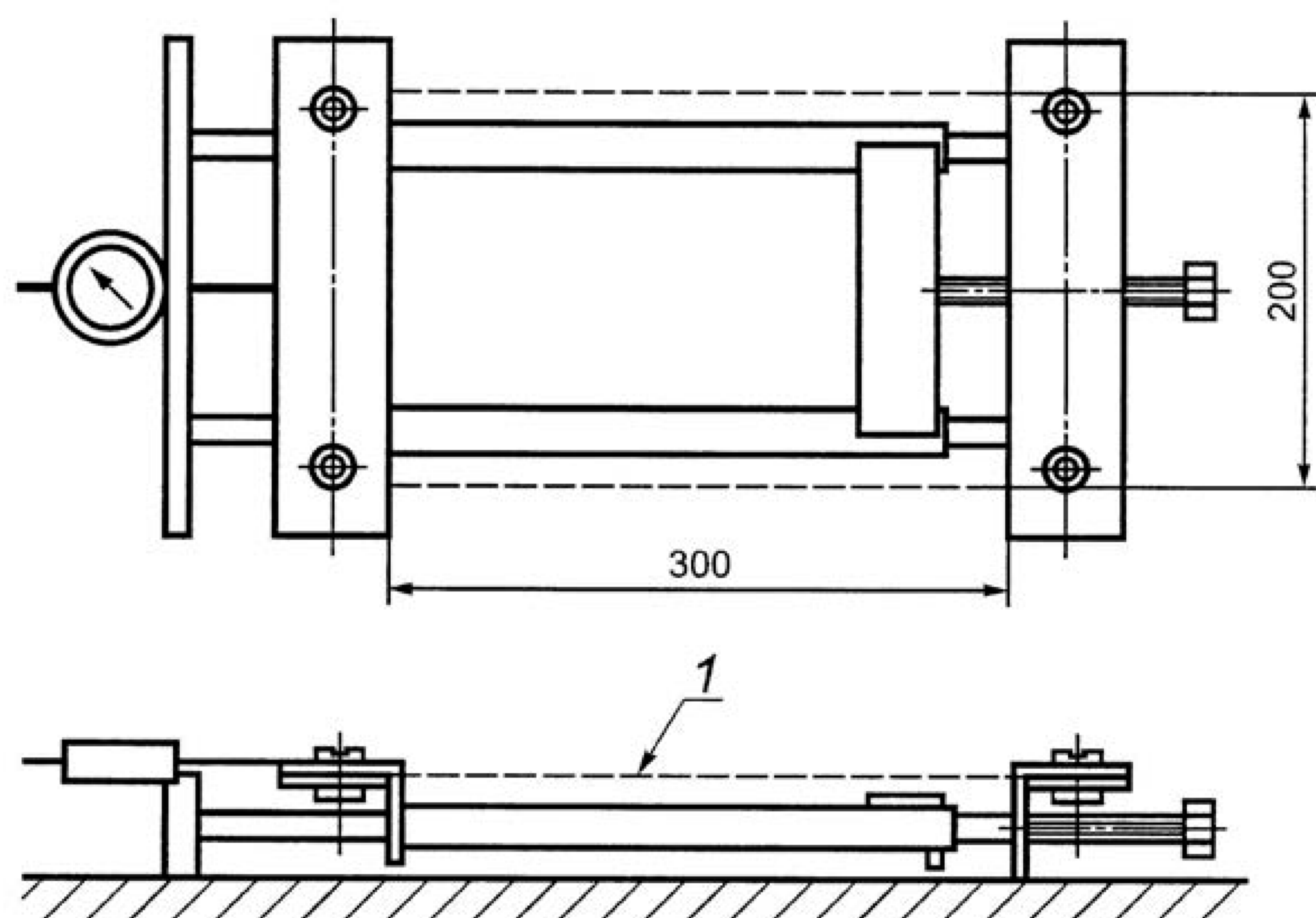
Рисунок 1 – Устройство для растяжения образца
