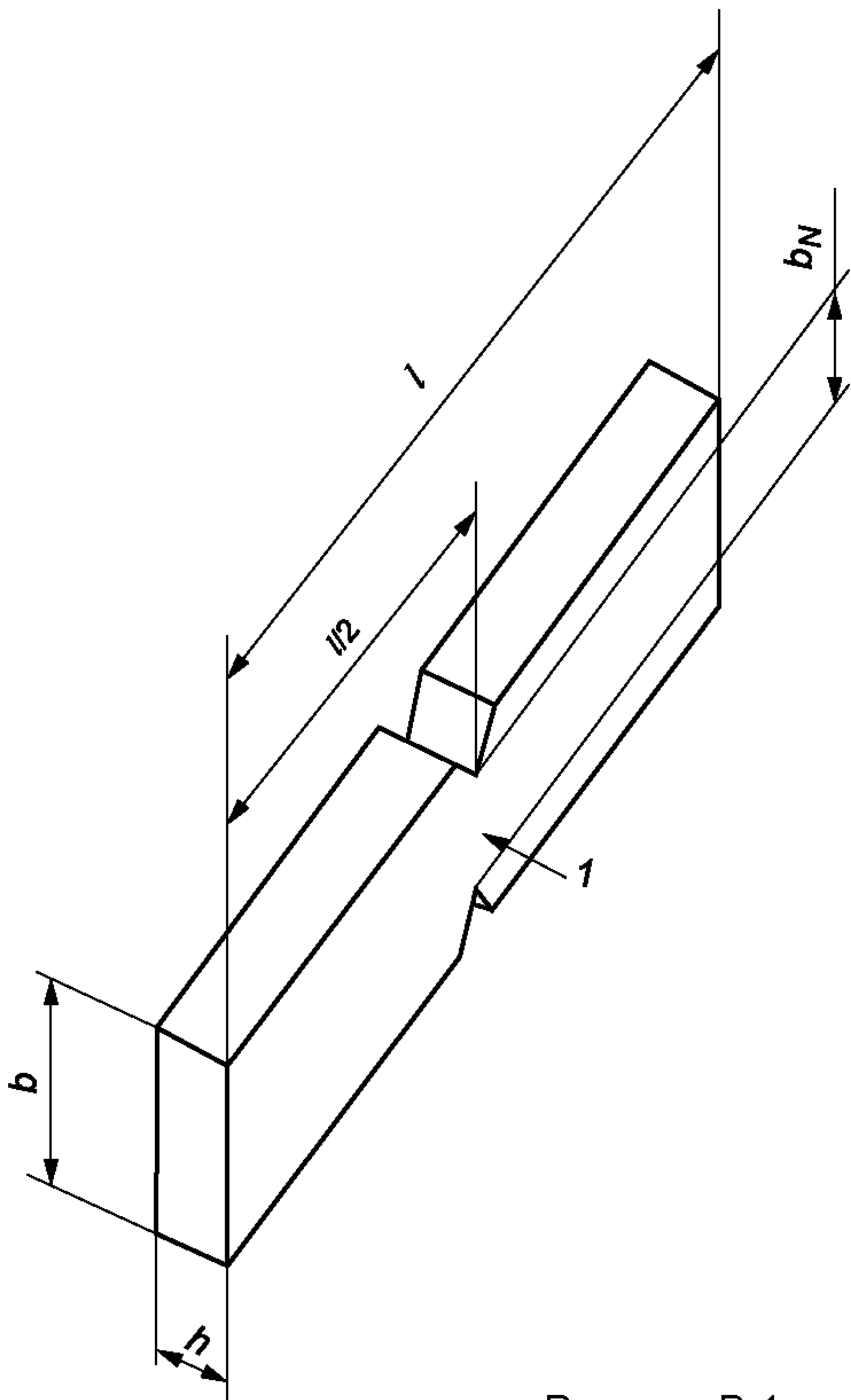
Рисунок В.1 — Образец с двойным V-образным надрезом
