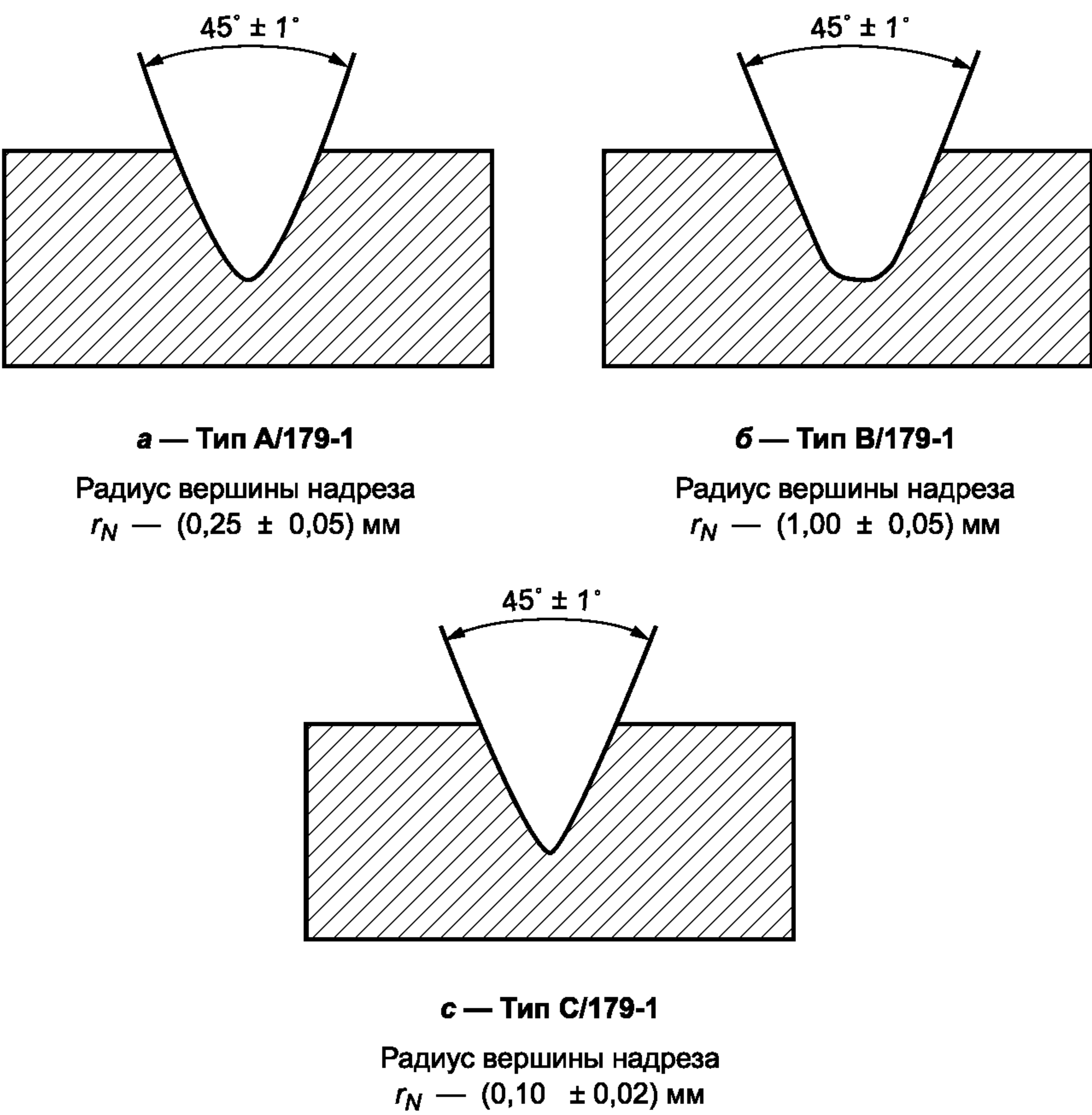
Рисунок 6 — Типы надрезов
