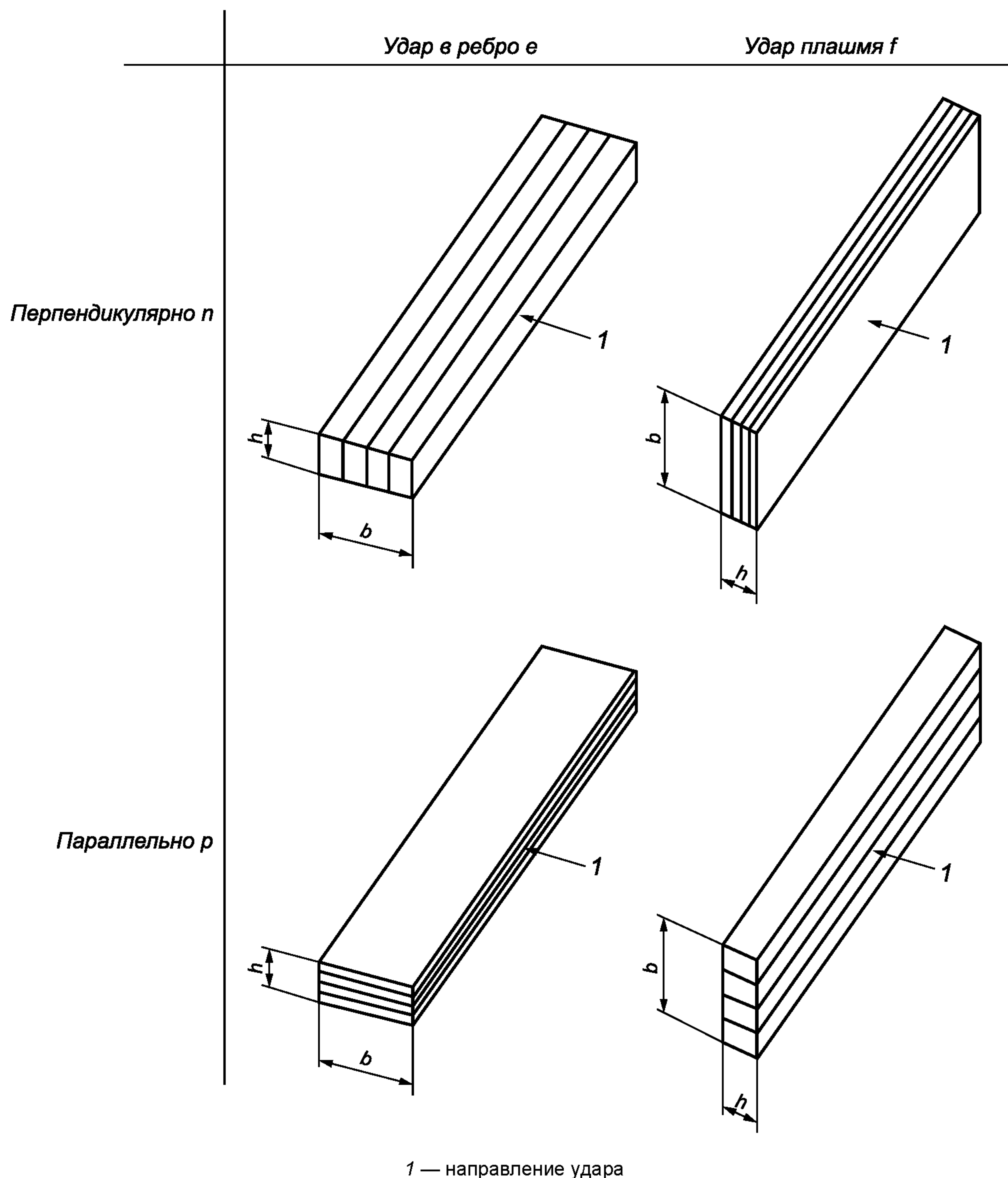
Рисунок 3 — Схема обозначений, описывающих направление удара
