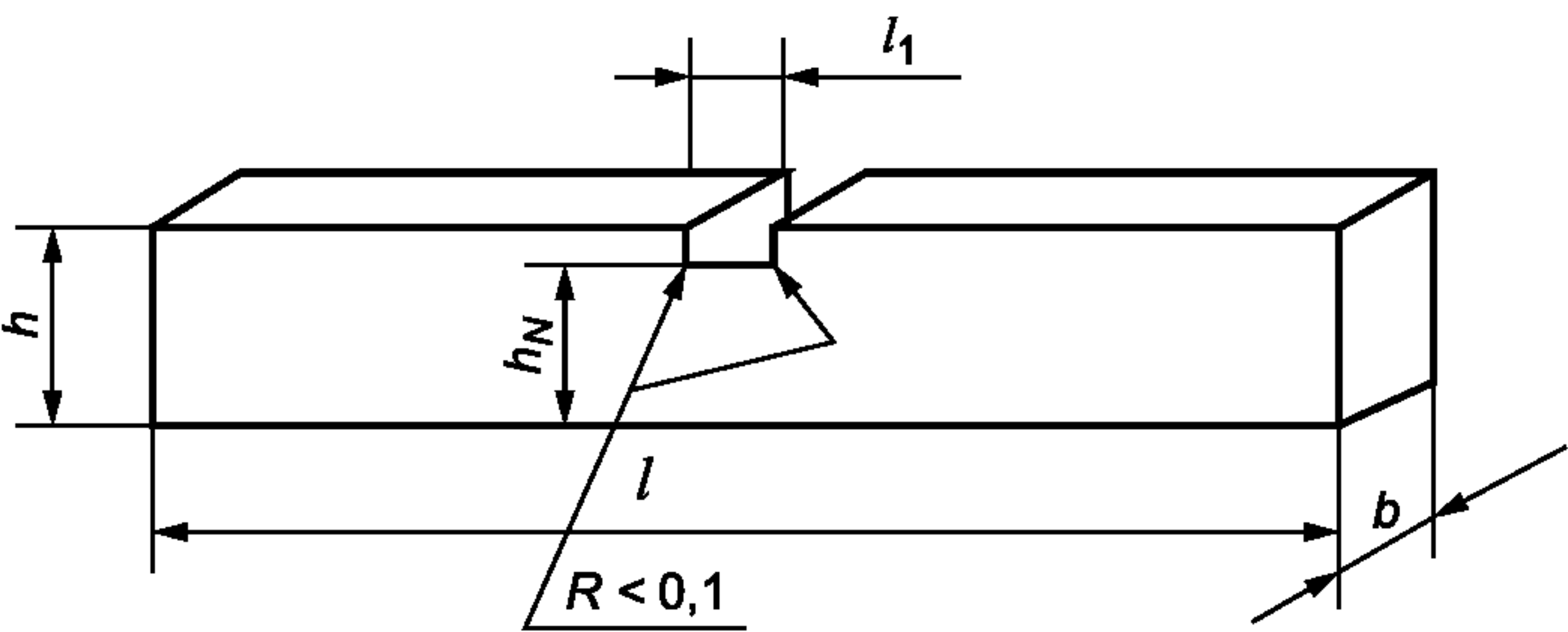
Рисунок 4 — Надрез типа А
