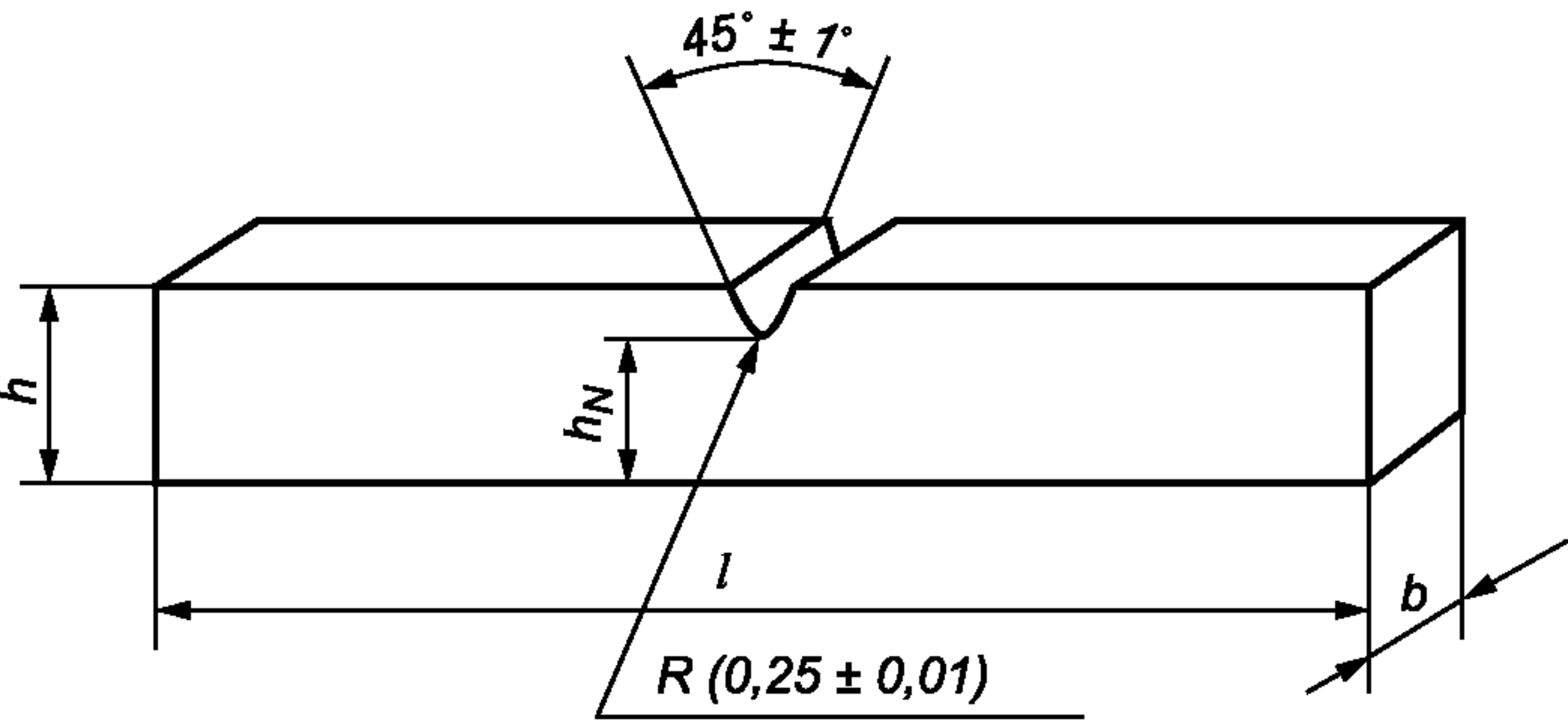
Рисунок 5 — Надрез типа В
