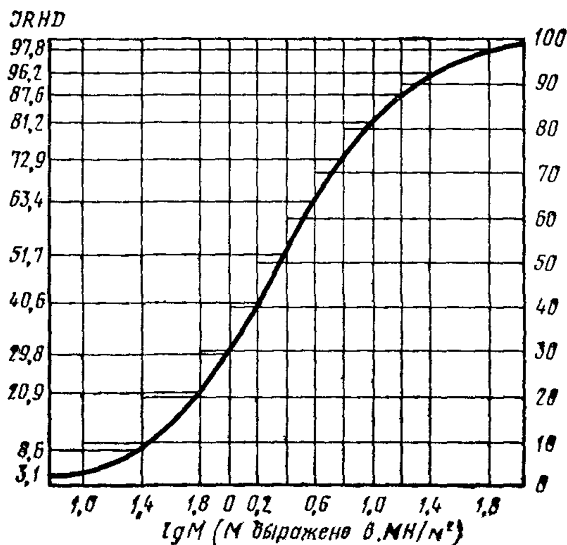
Зависимость твердости резины от модуля упругости
