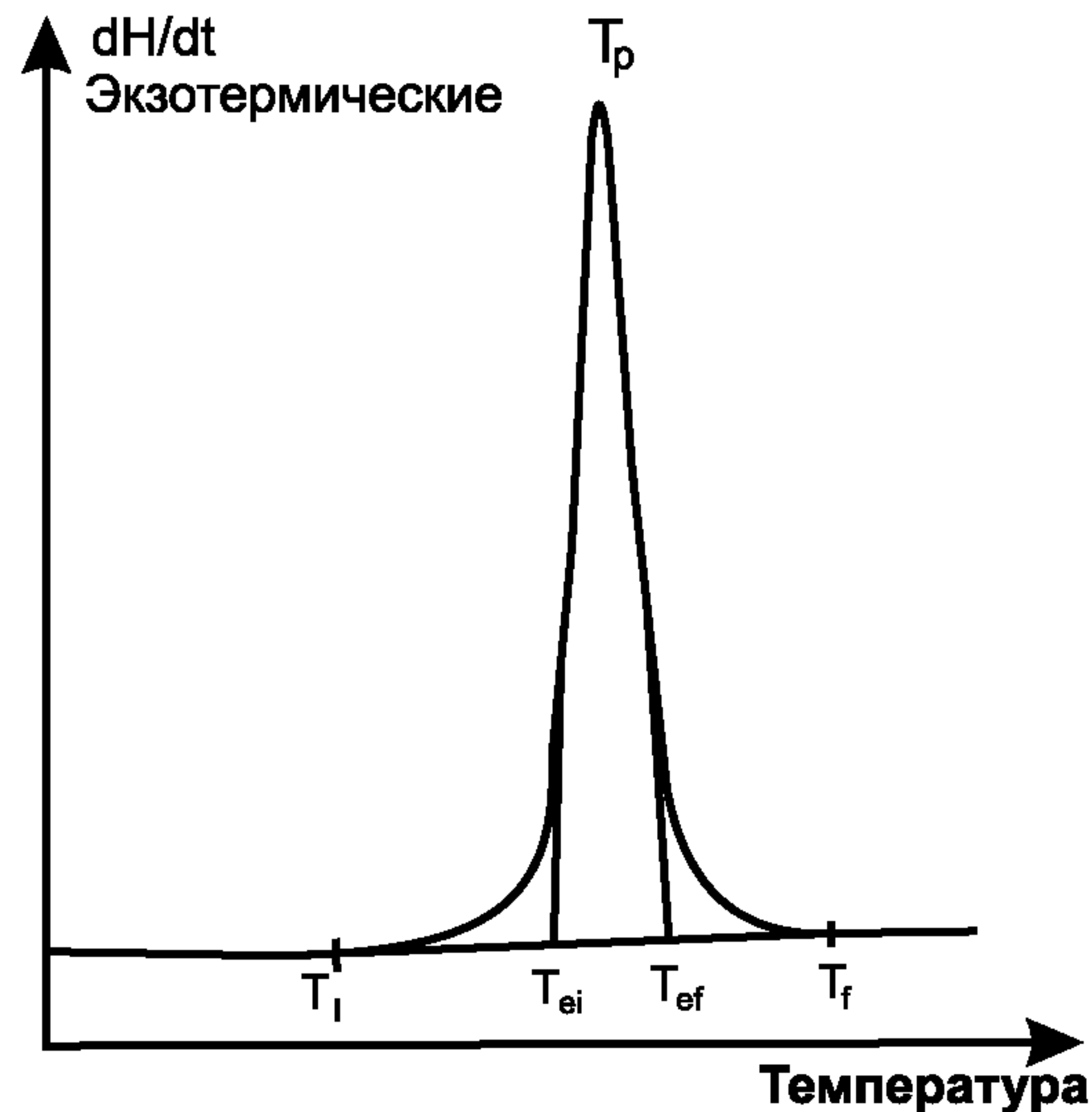
Рисунок ДБ.1 – ДСК кривая с экзотермическим пиком (метод сканирования, чувствительный к температуре)
