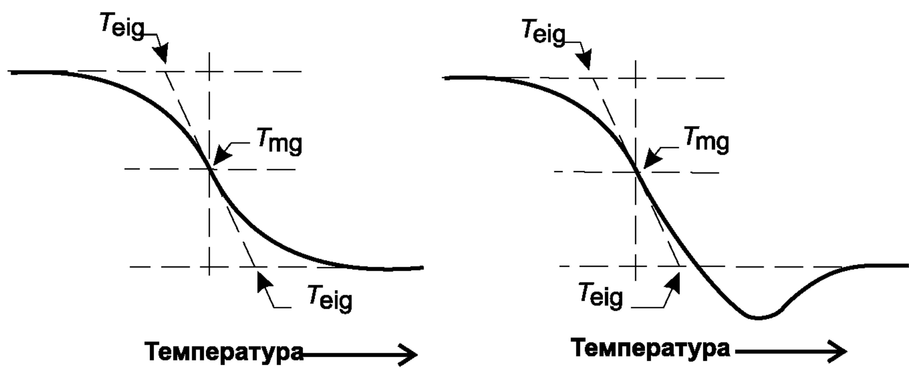
Рисунок ДА.1 – Примеры определений кривой температуры стеклования
