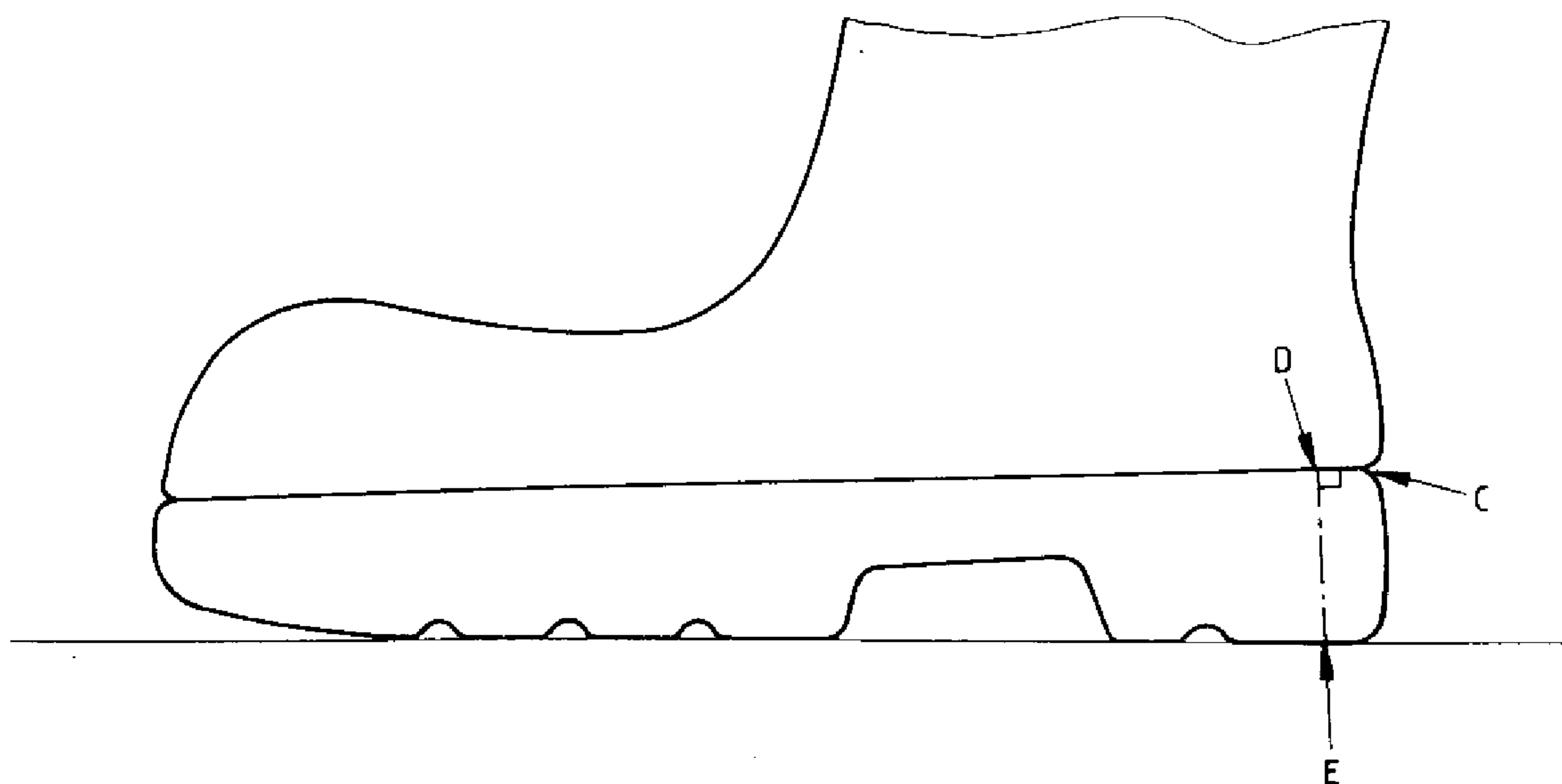
Рисунок А.1 – Измерение толщины каблука
