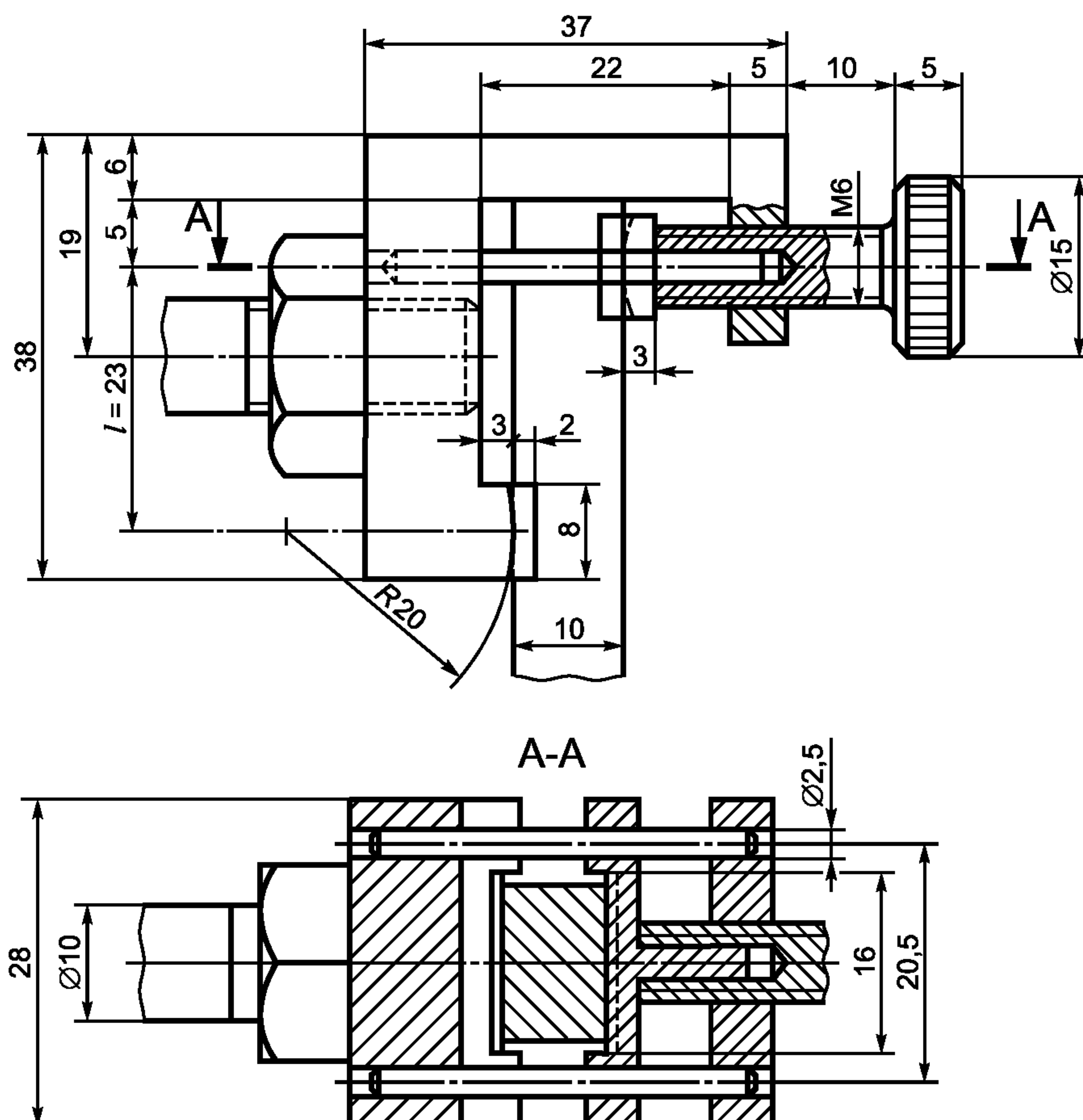
Рисунок 3 — Верхняя зажимная головка для образца 1
