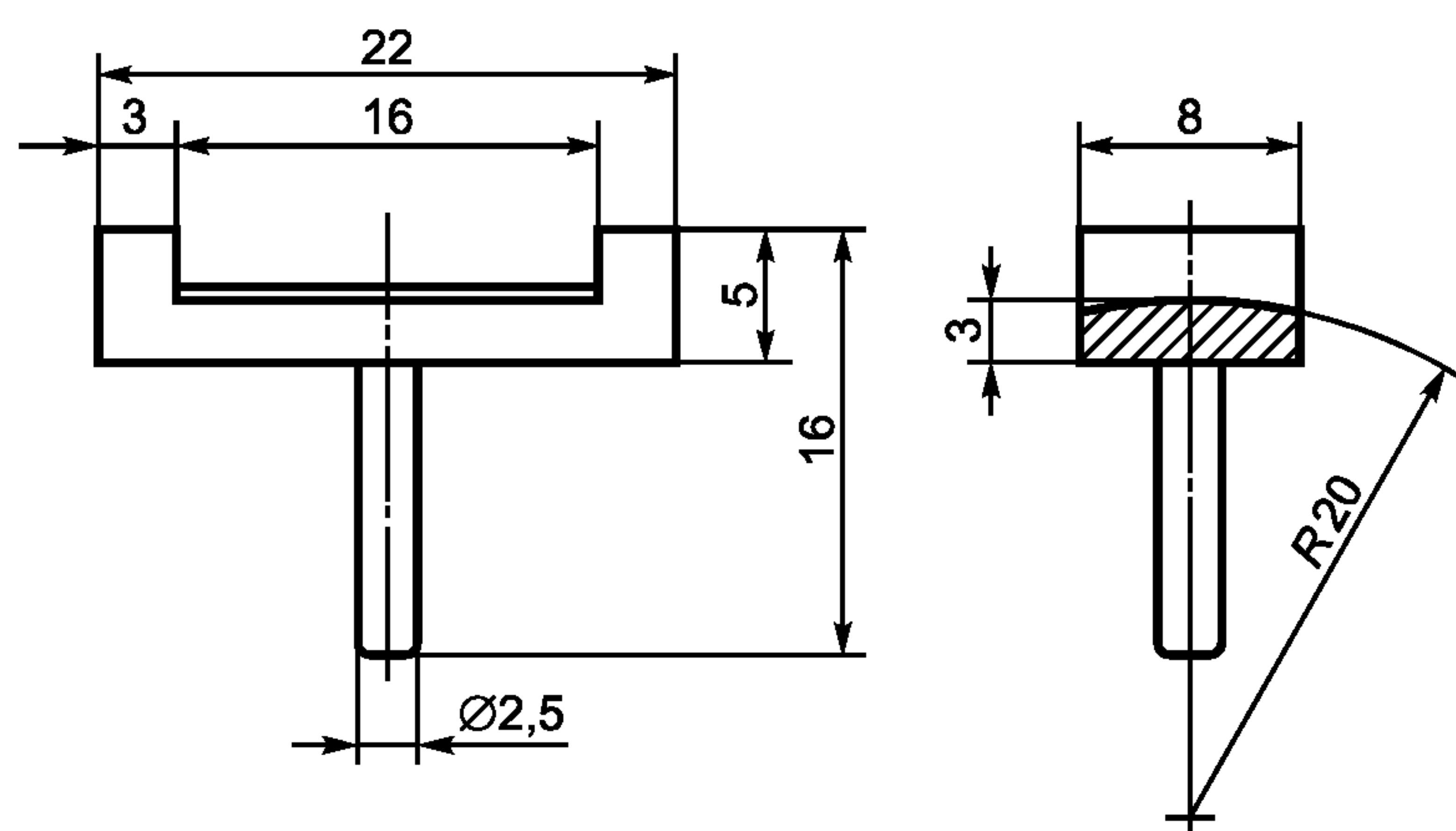
Рисунок 6 — Сменный упор для зажимной головки для образца 2
