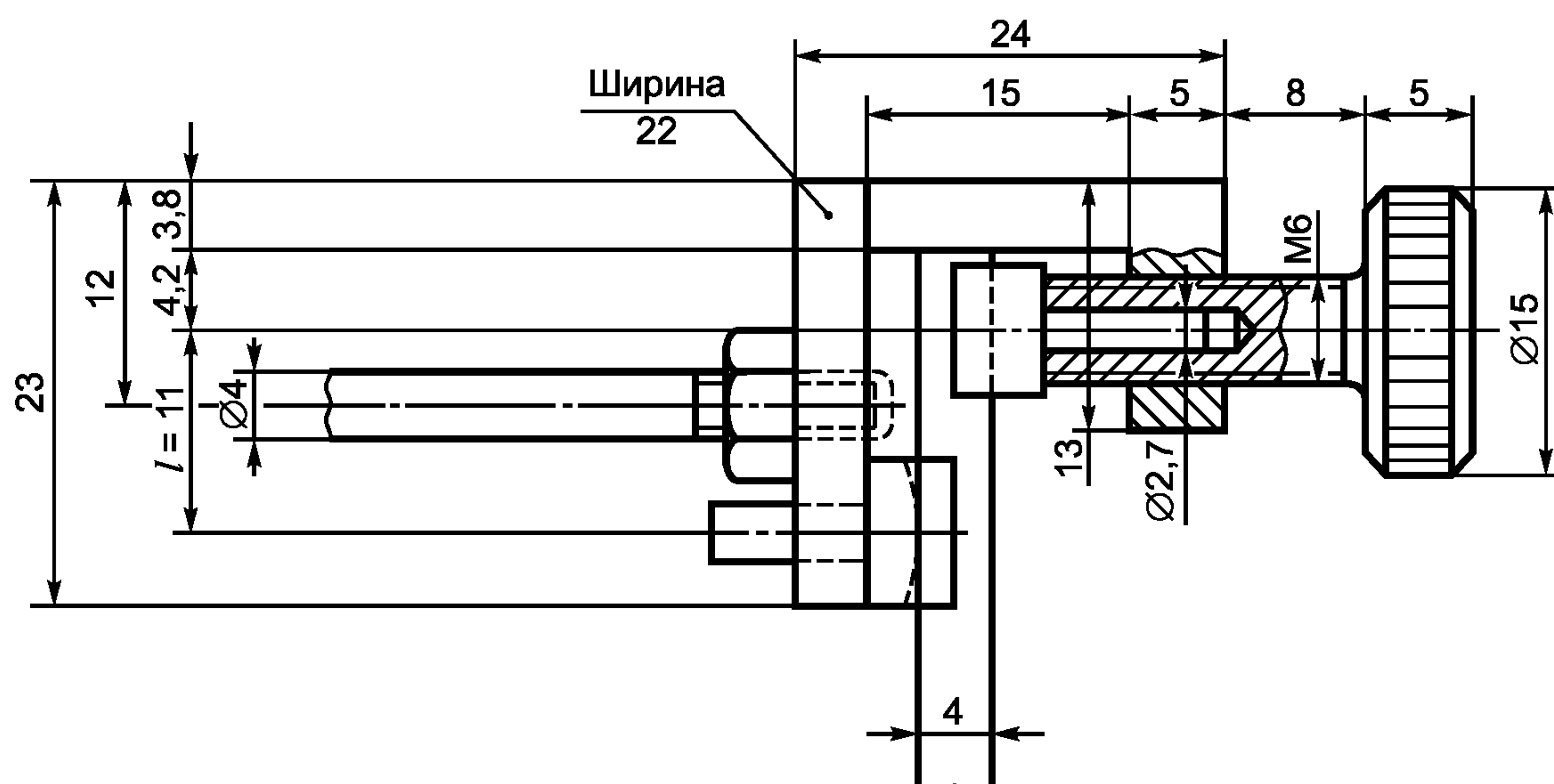
Рисунок 4 — Верхняя зажимная головка для образцов 2 и 3
