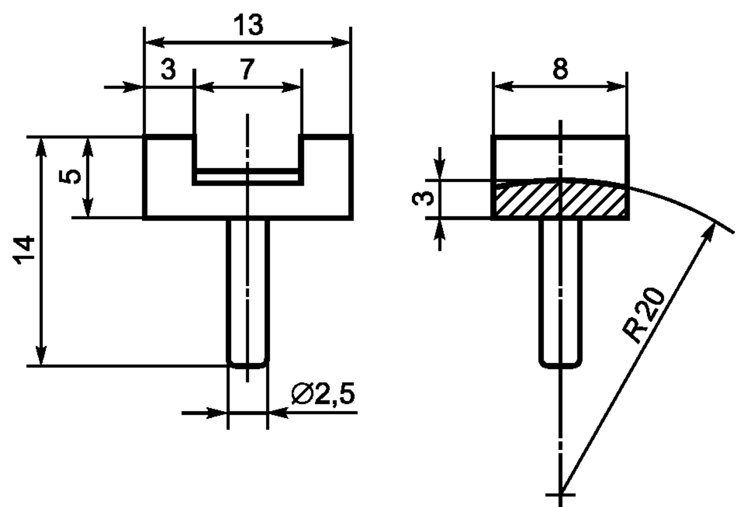
Рисунок 7 — Сменный упор для зажимной головки для образца 3
