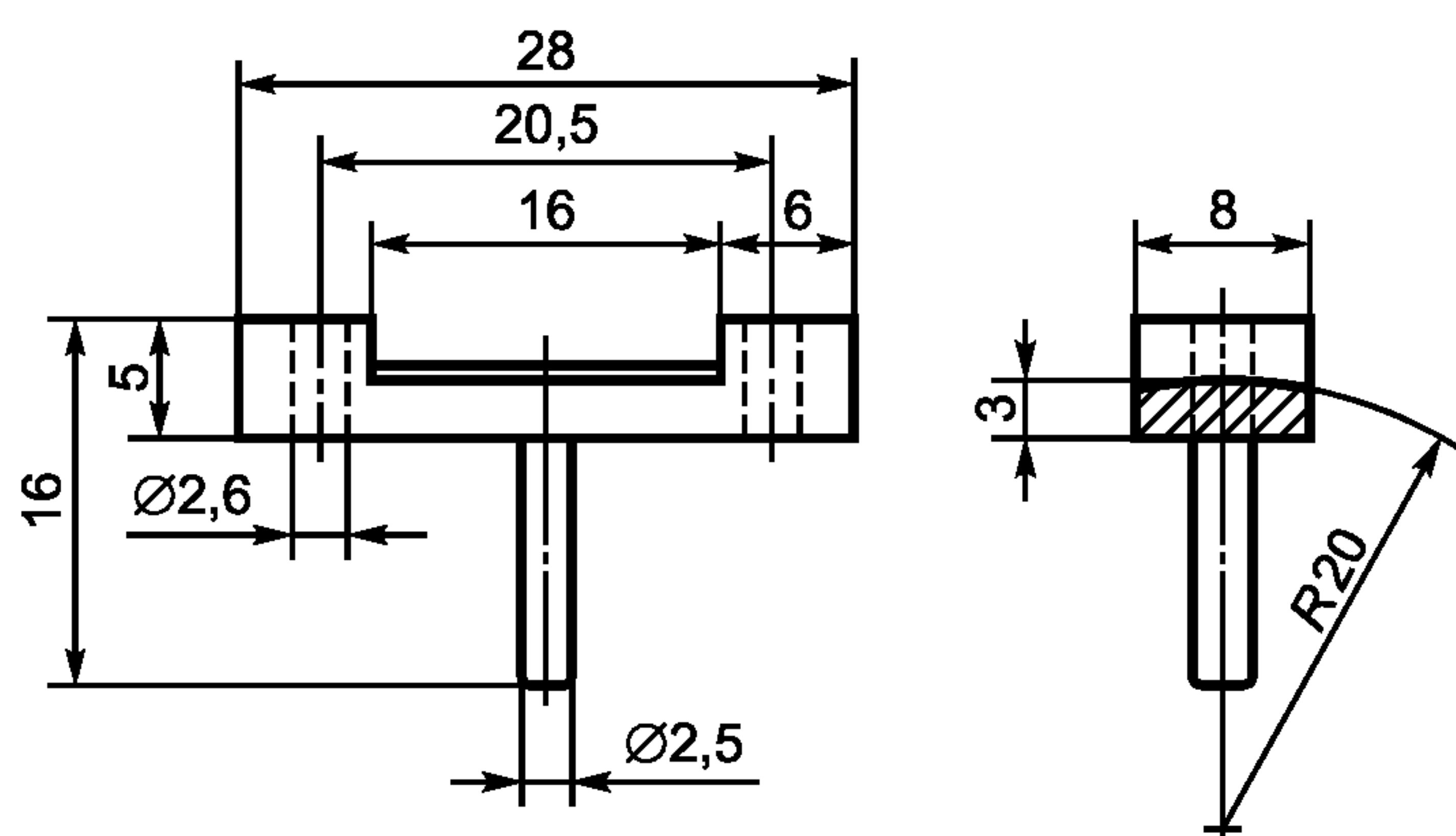
Рисунок 5 — Сменный упор для зажимной головки для образца 1
