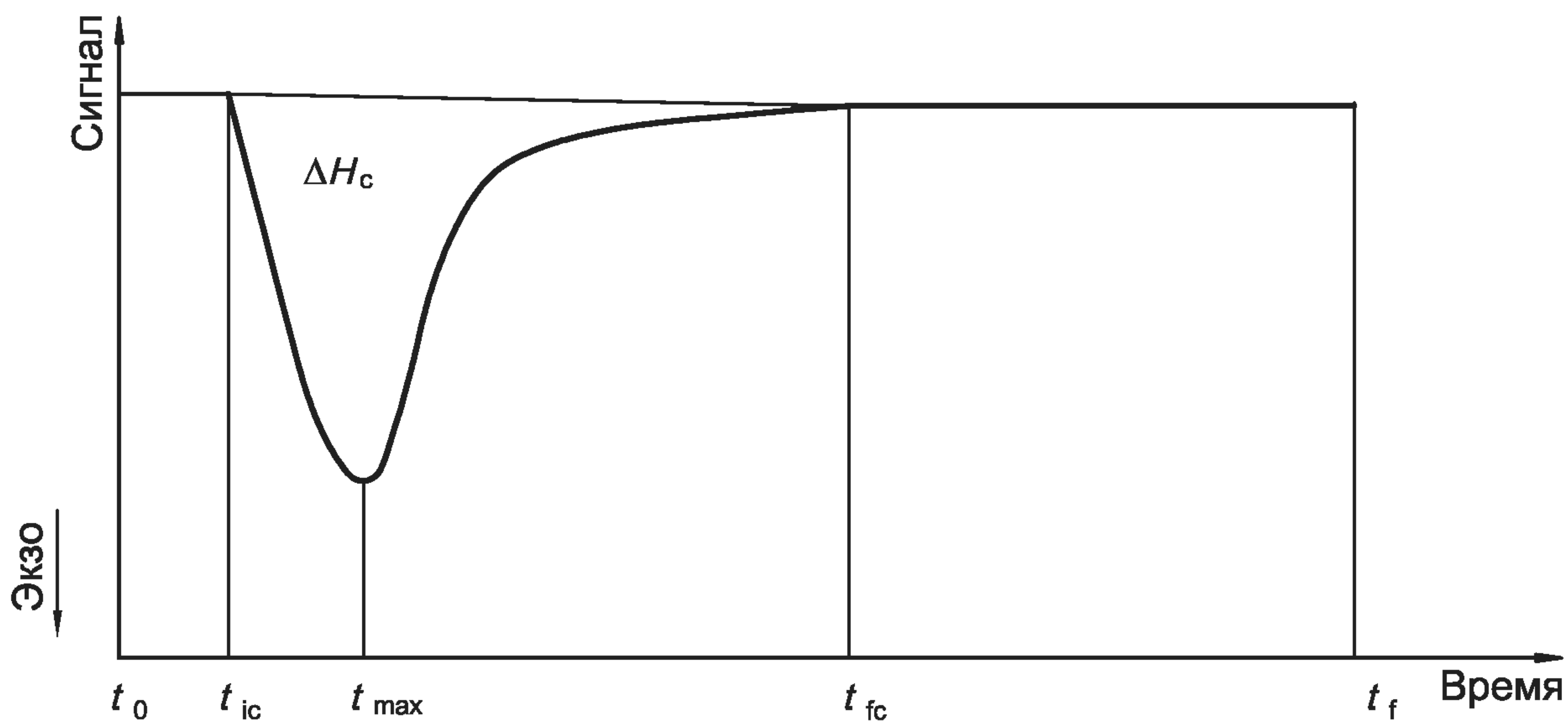
Рисунок 3 — Сигнал ДСК на изотермической стадии
