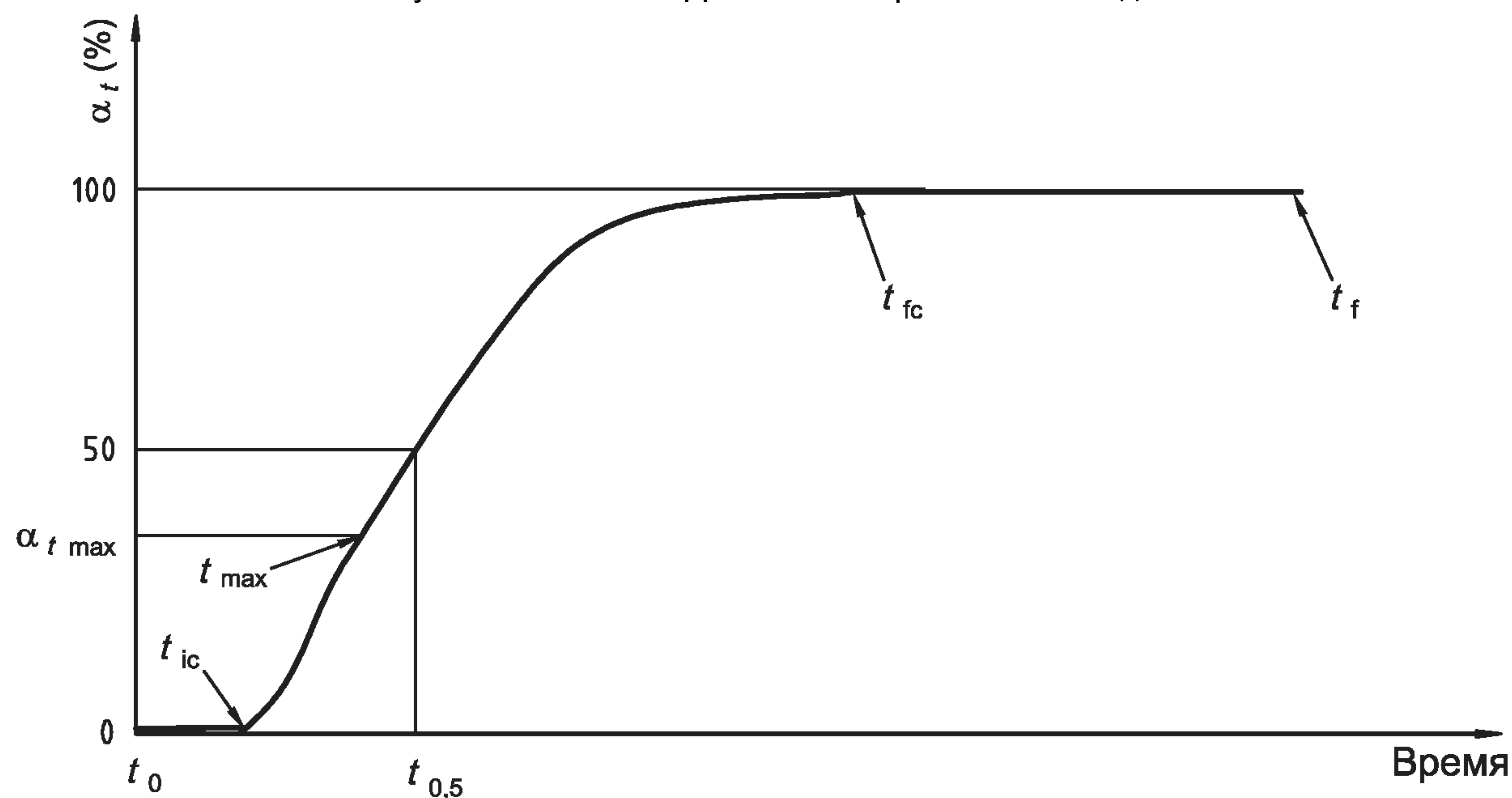
Рисунок 4 — Изменение \alpha_t на изотермической стадии
