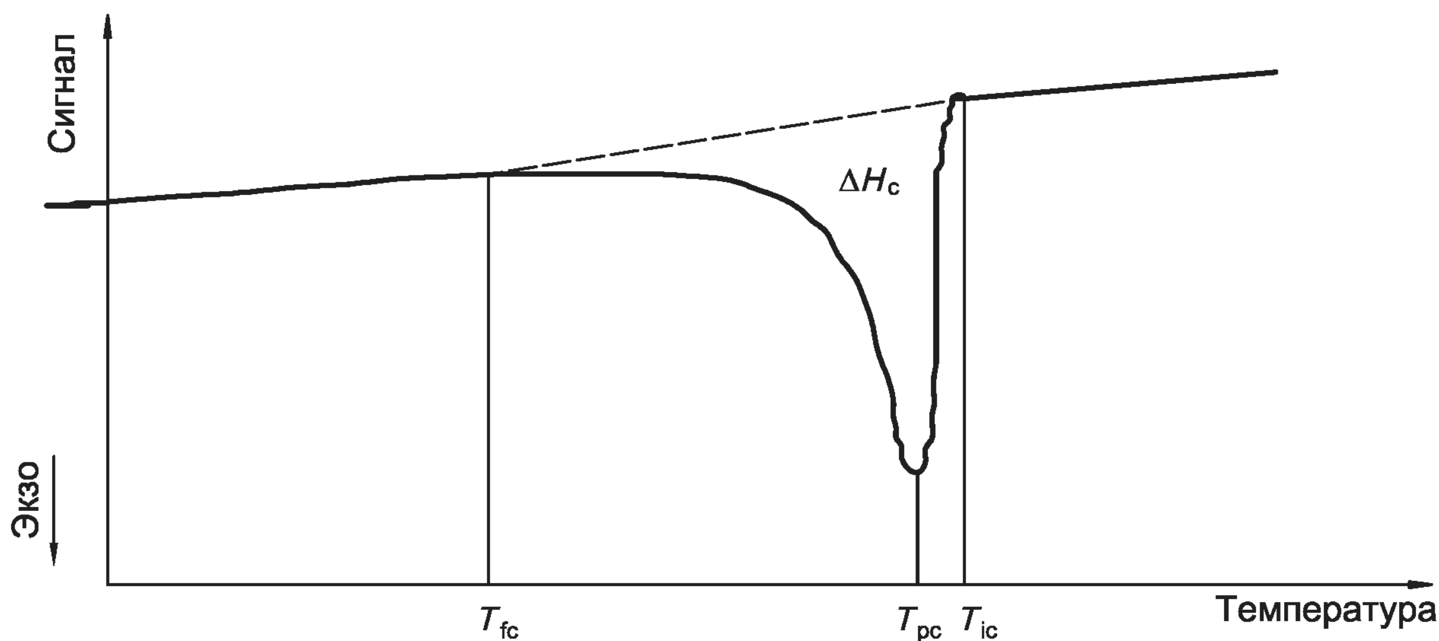
Рисунок 5 — Сигнал ДСК на стадии охлаждения
