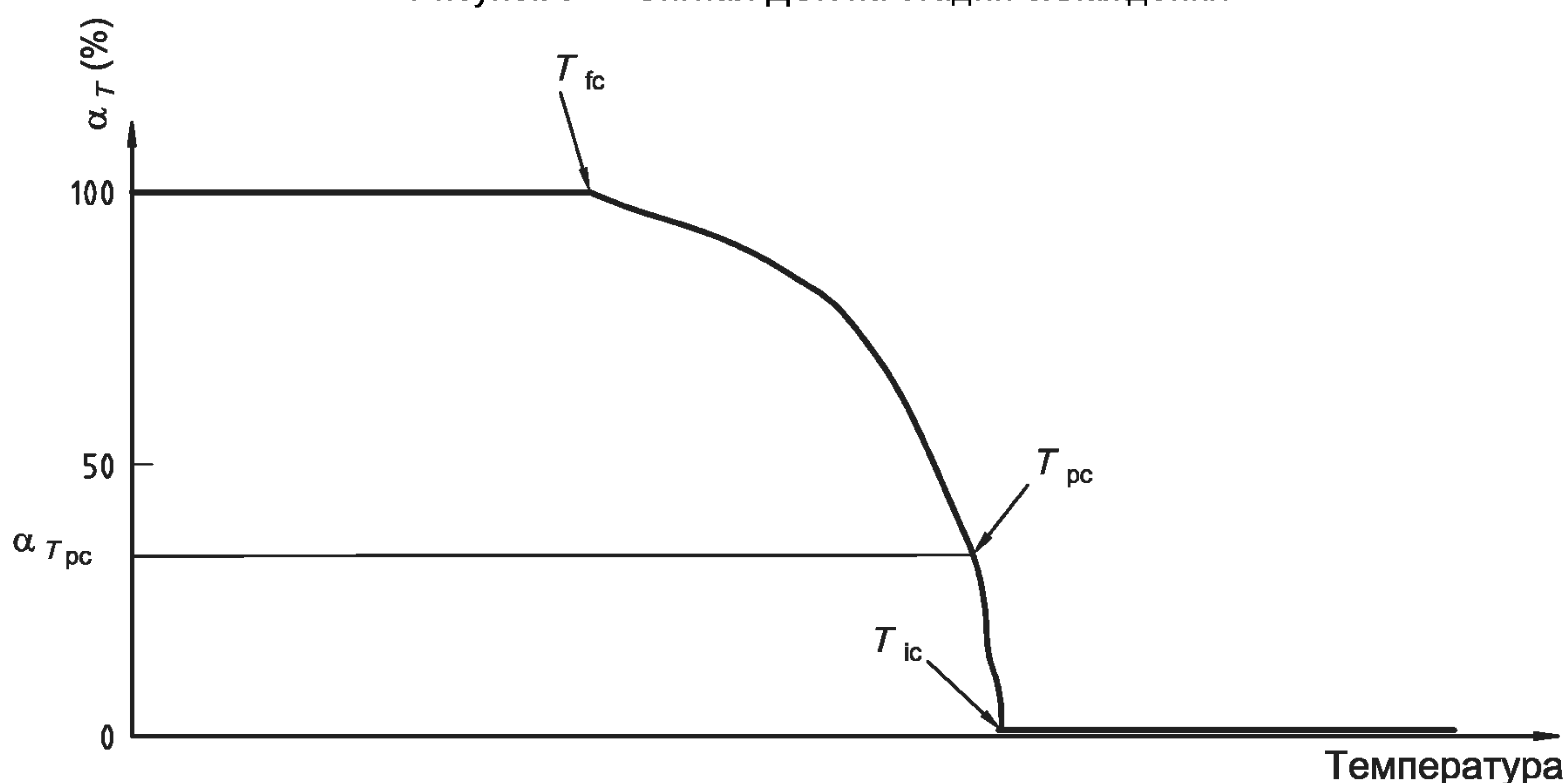
Рисунок 6 — Изменение \alpha_T на стадии охлаждения
