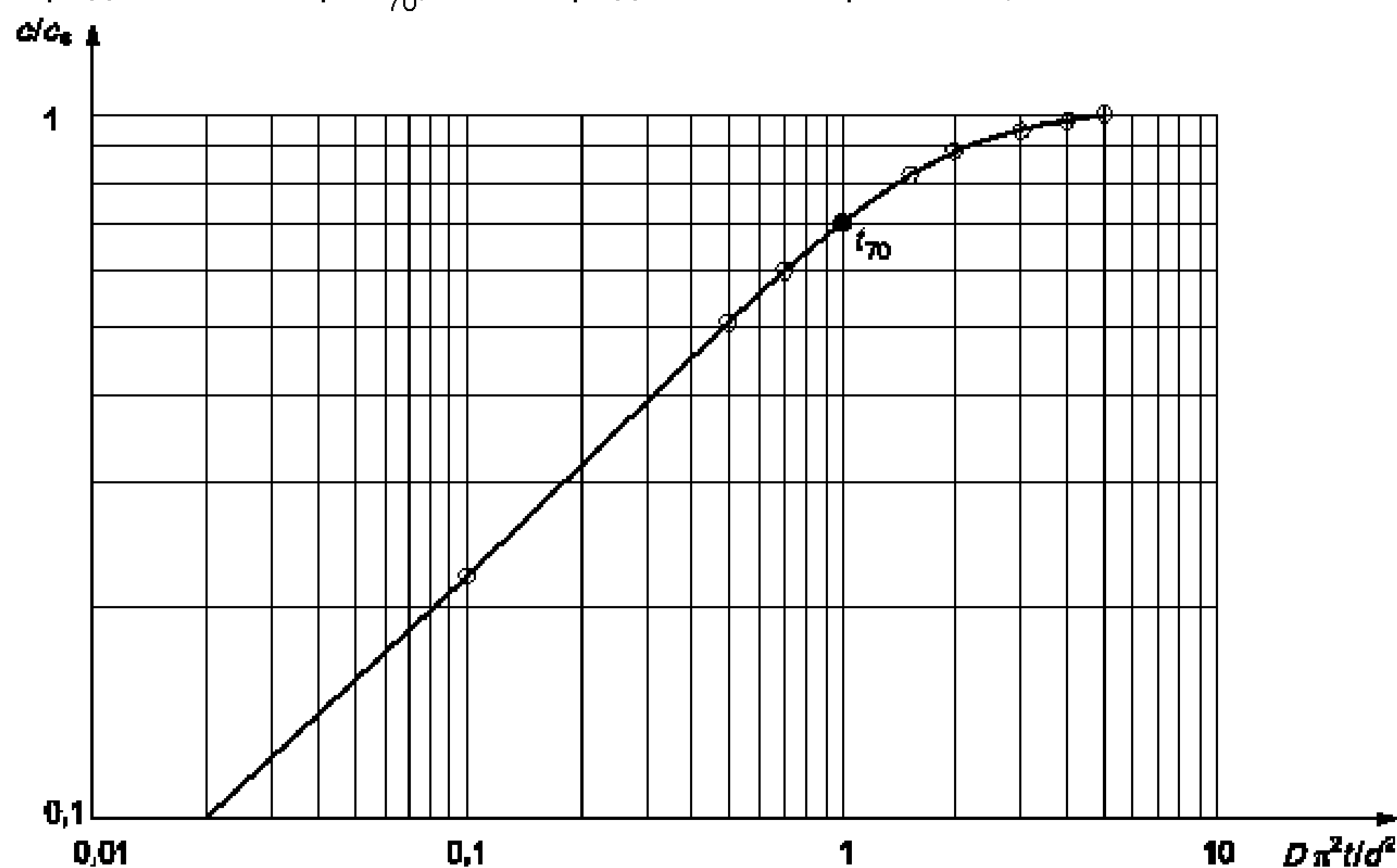
Рисунок А.1 — Водопоглощение c/c_s листов в зависимости от безразмерной функции D\pi^2 t/d^2 ( D – коэффициент диффузии; t – продолжительность выдерживания в воде; d – толщина образца)
