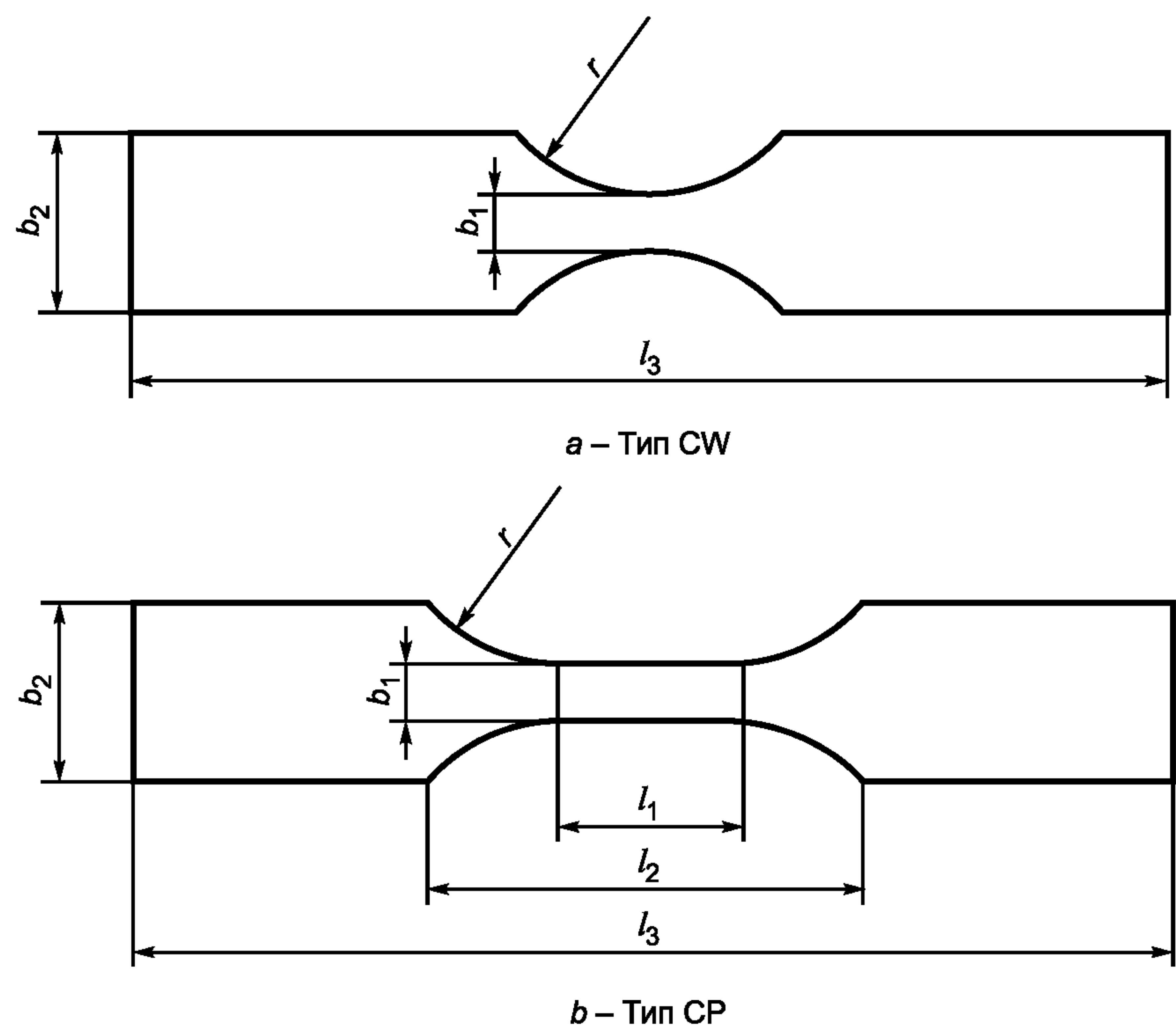
Рисунок 2 — Образцы для испытания типа CW и типа CP
