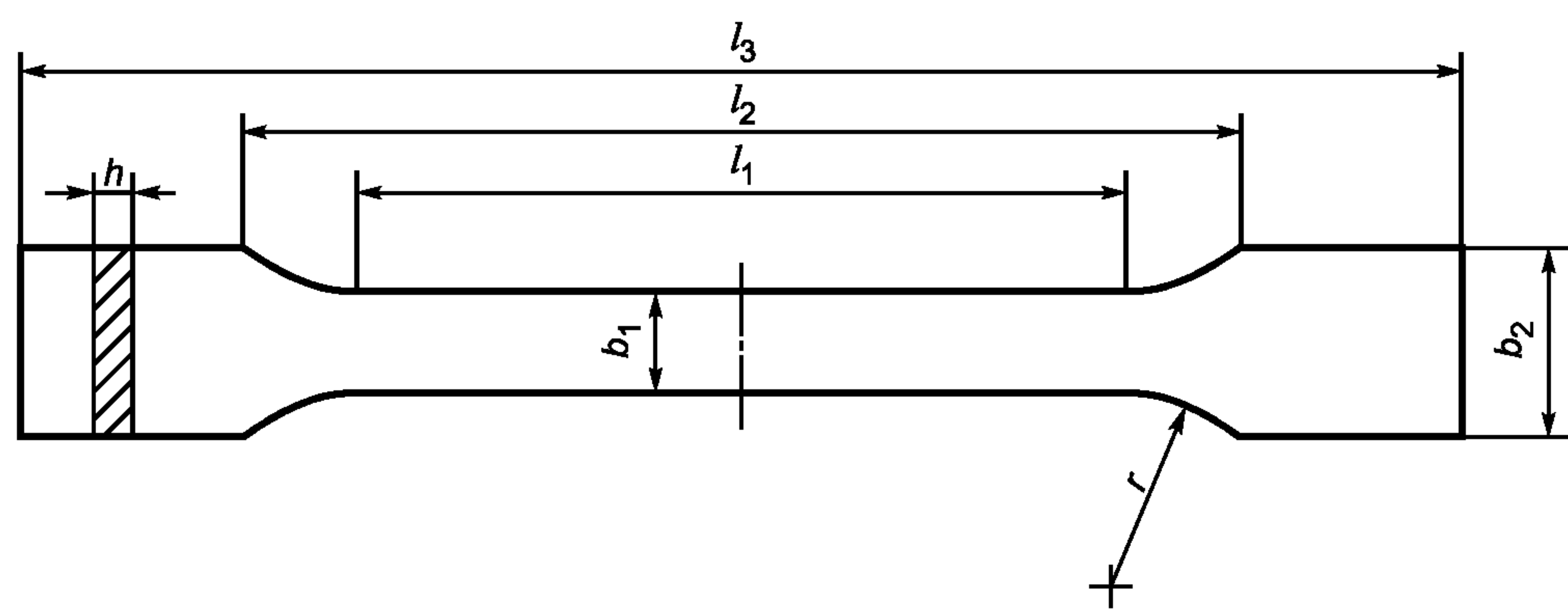
Рисунок 1 — Типовой образец для испытания на растяжение
