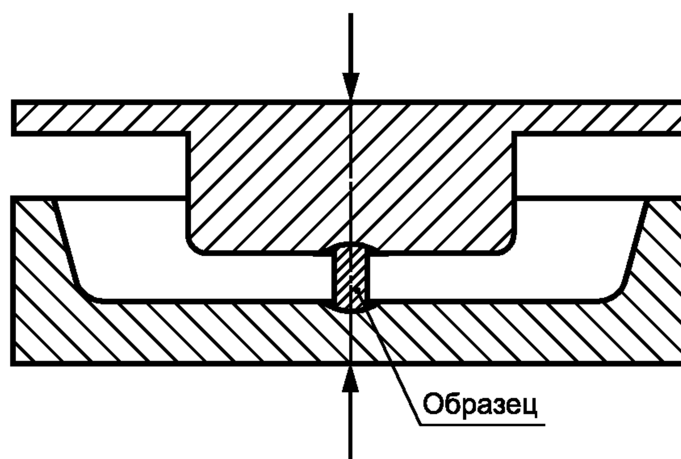
Рисунок ДА.1 — Штамповка для измельчения
