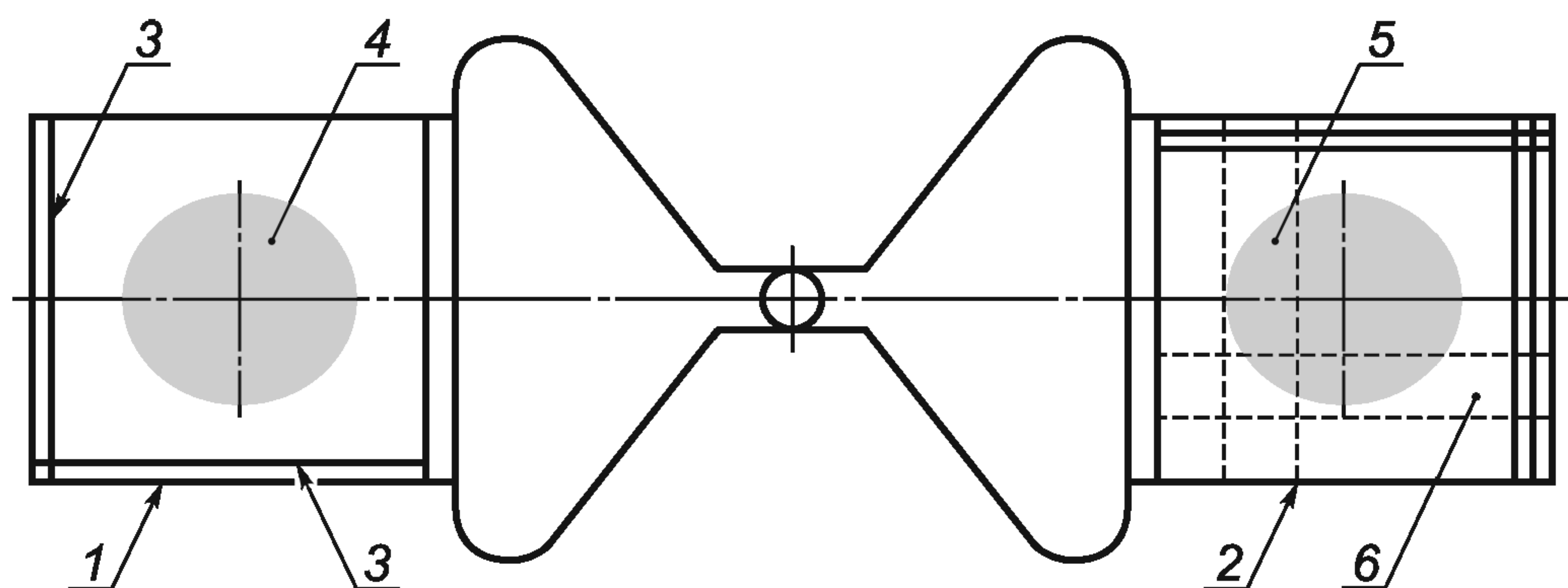
1 — полость 1; 2 — полость 2; 3 — линии разметки; 4 — зона испытания (диаметр 50 мм); 5 — n -образец; 6 — p -образец
