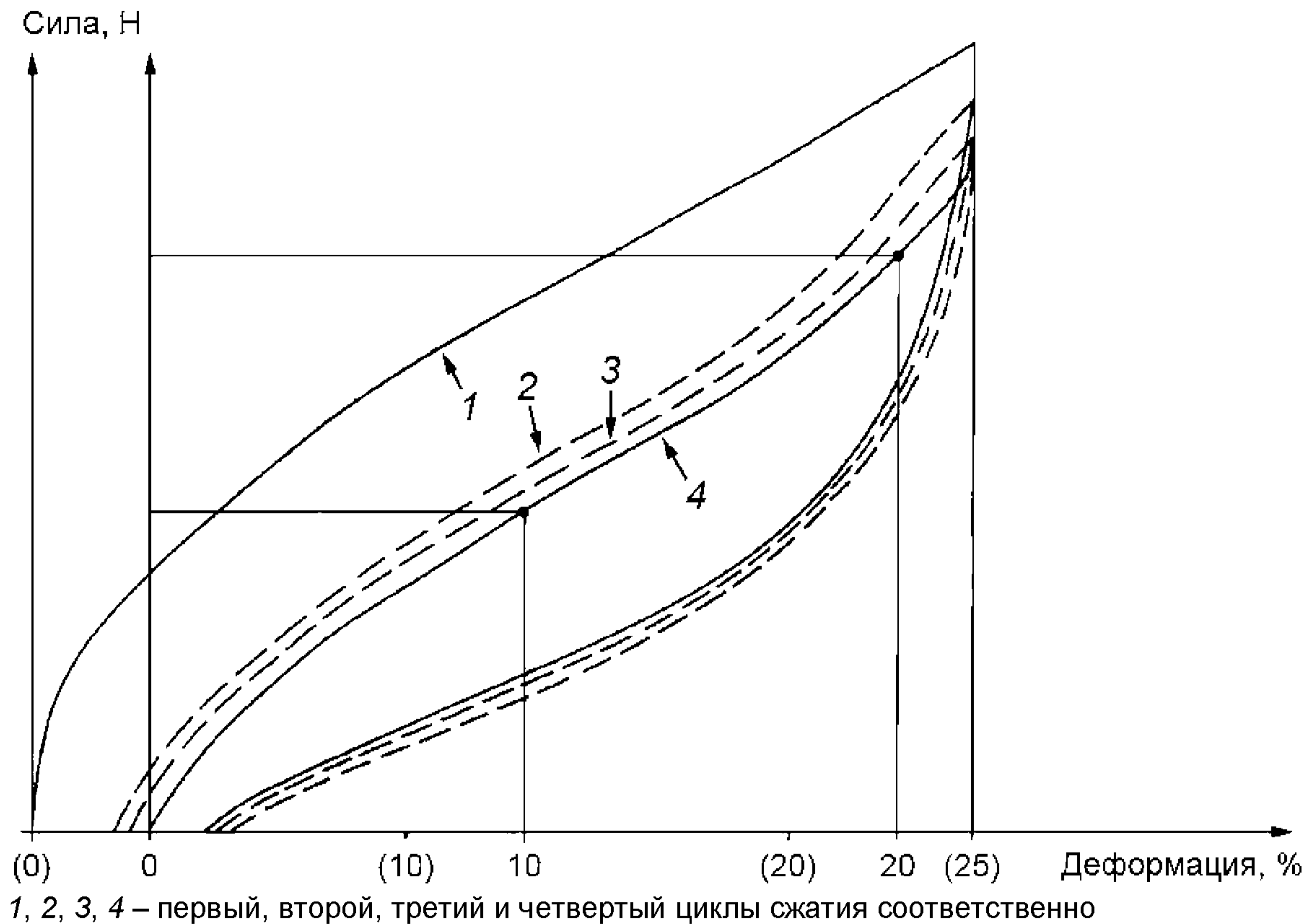
Рисунок 1 – Вычисление модуля сжатия
