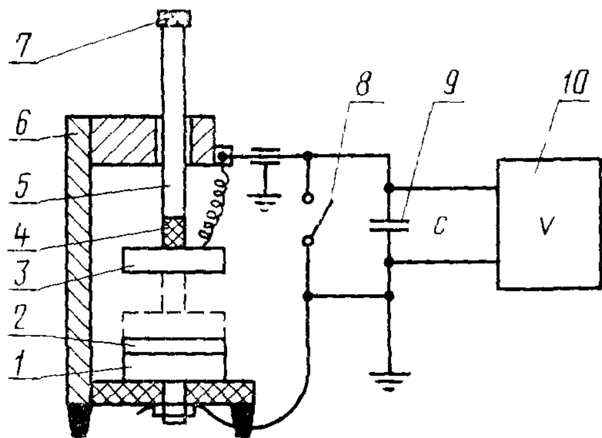
1—нижний неподвижный электрод; 2—образец электрета; 3—верхний подвижной электрод; 4—изолятор; 5—штук; 6—штатив; 7—ручка для подъема электрода; 8—переключатель; 9—конденсатор; 10—вольтметр-электрометр
