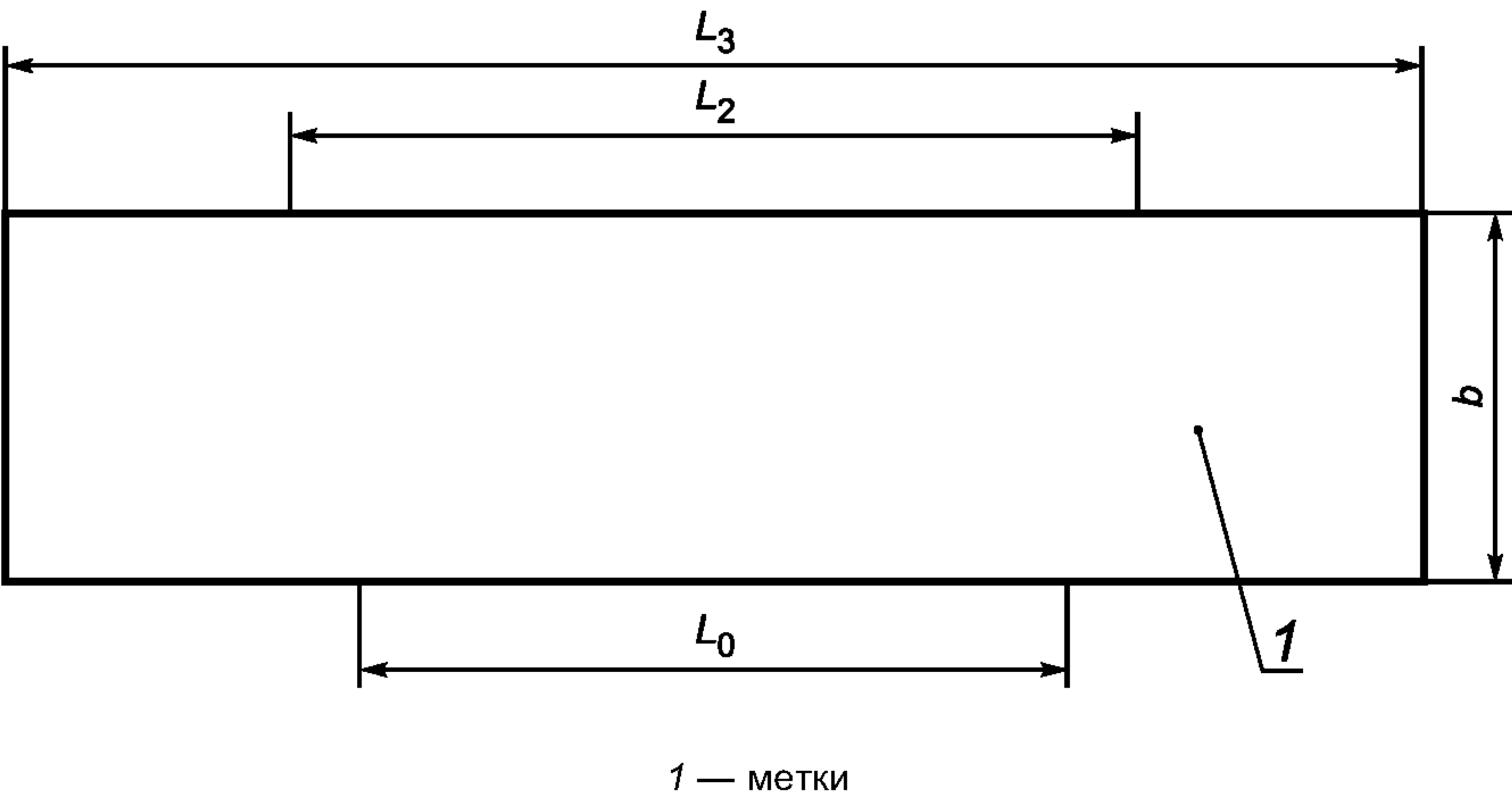
Рисунок 1 — Образец-полоска (метод А)
