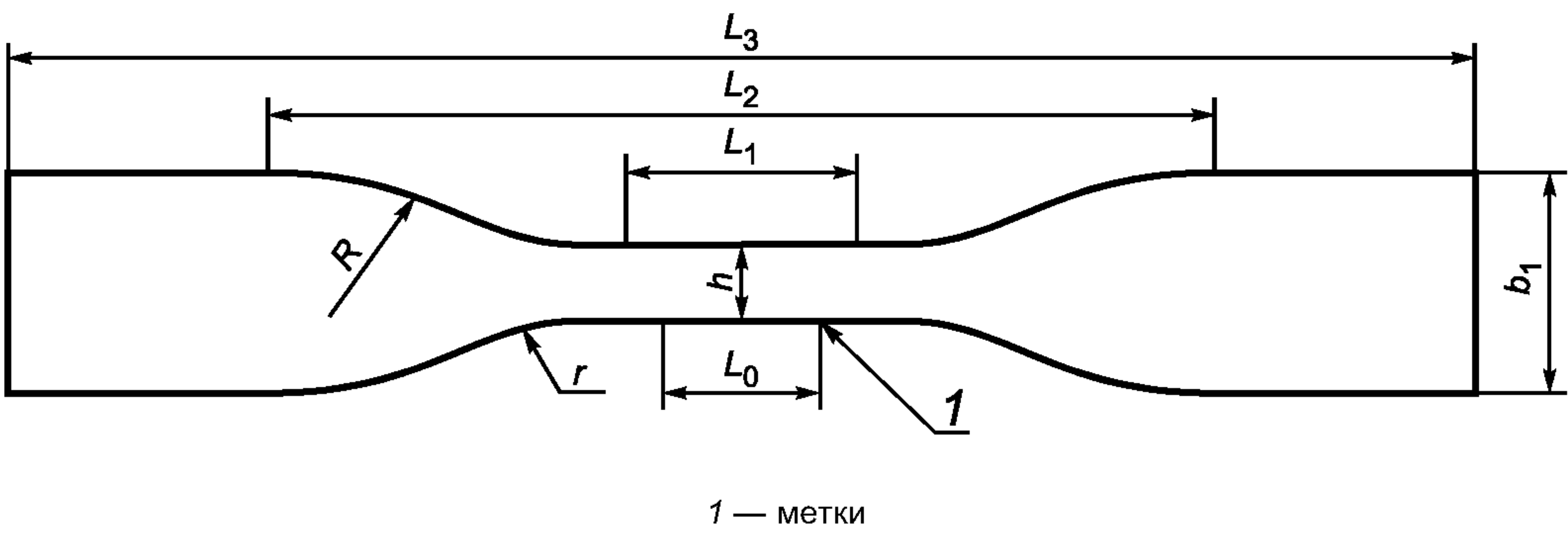
Рисунок 2 — Образец-лопатка (метод В)
