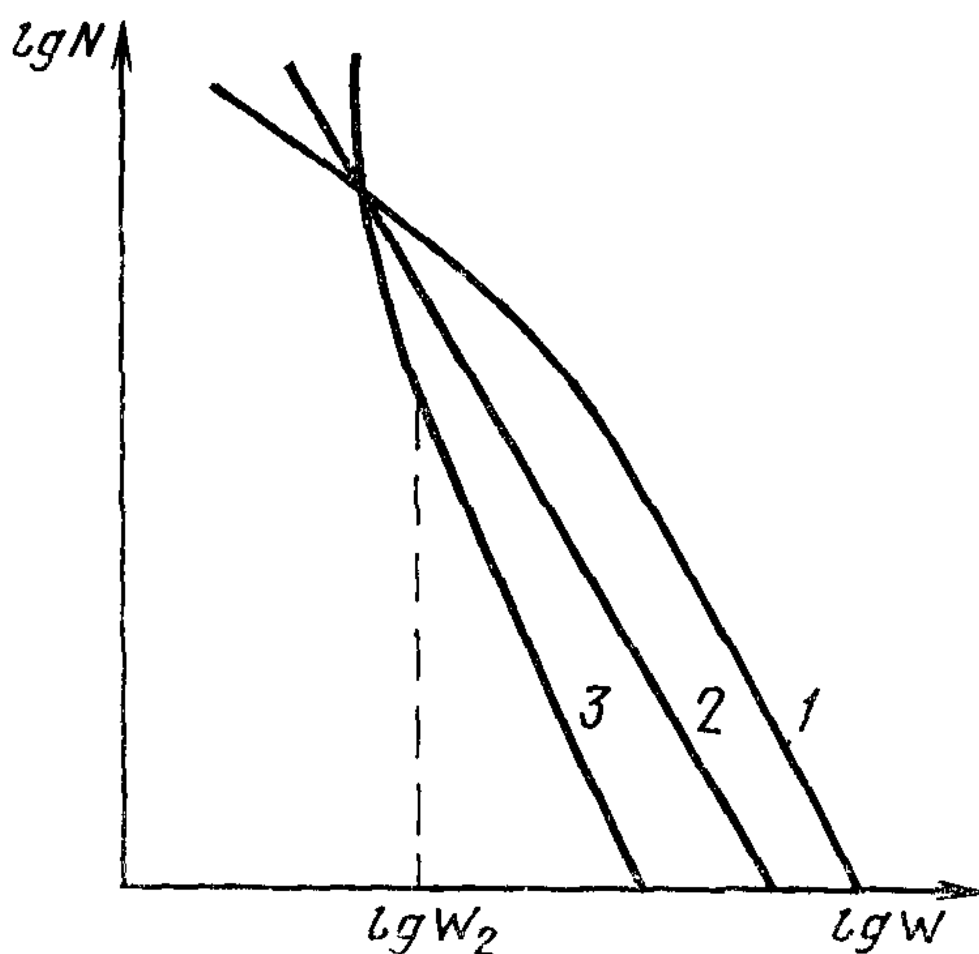
Зависимость усталостной выносливости от удельной энергии деформации для резины разного типа
