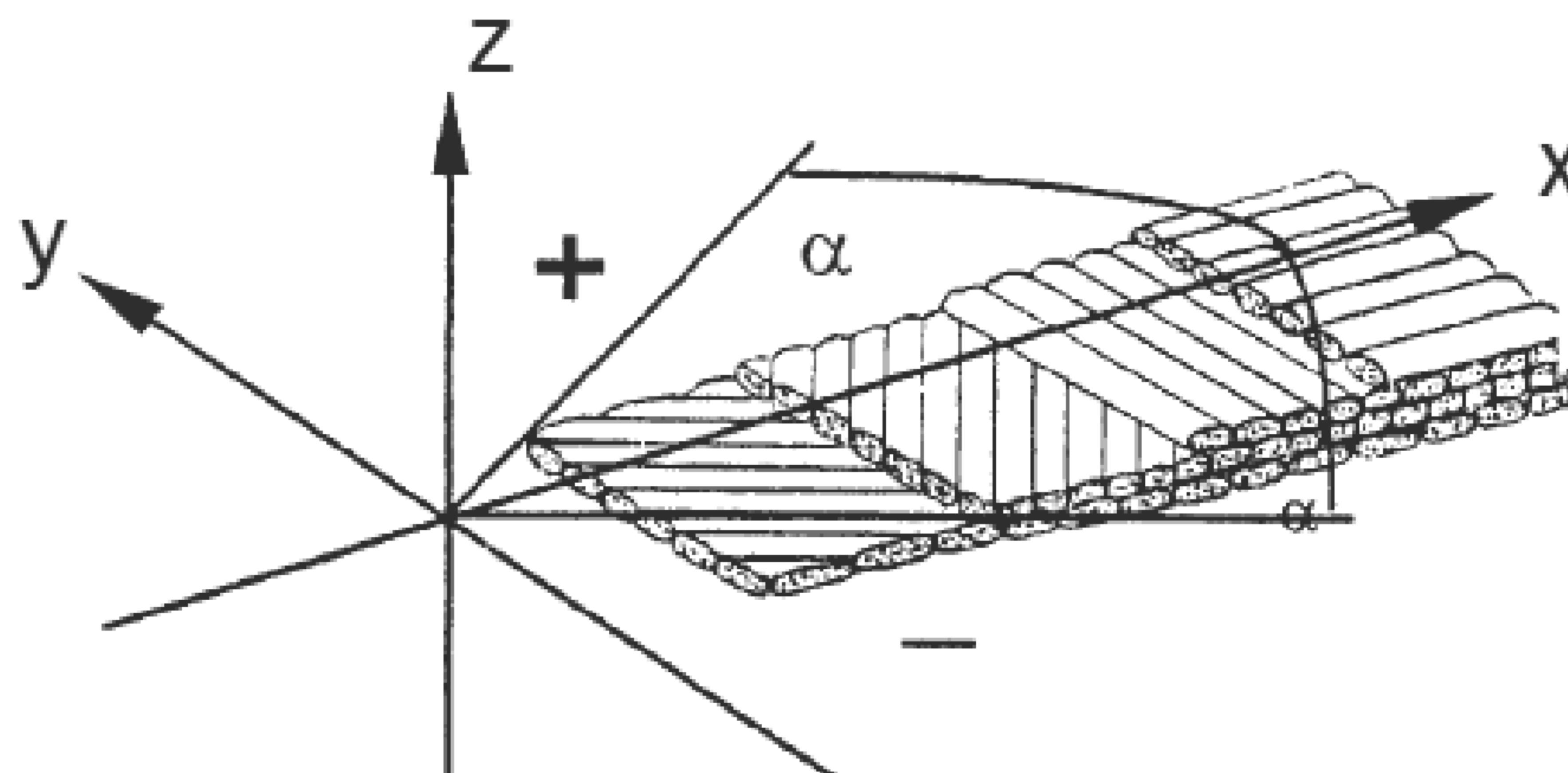
у– 90°; z– направление волокна; х – 0°, направление производства Рисунок 1 – Определение ориентации направления волокон
