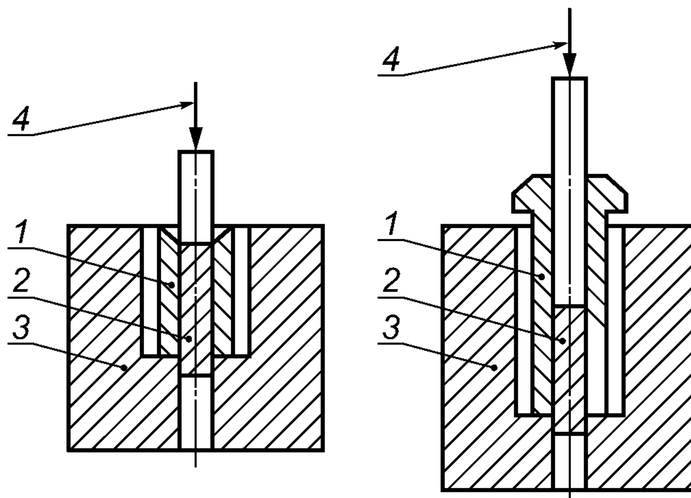
1 — корпус шипа; 2 — износостойкий элемент; 3 — подставка; 4 — направление выдавливания
