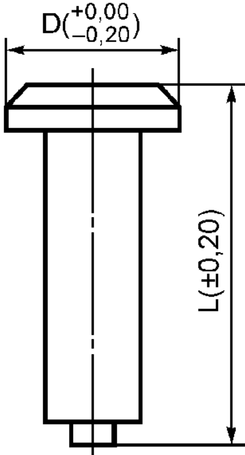
Рисунок 2 — Рекомендуемые размеры шипа с предельно допустимыми отклонениями
