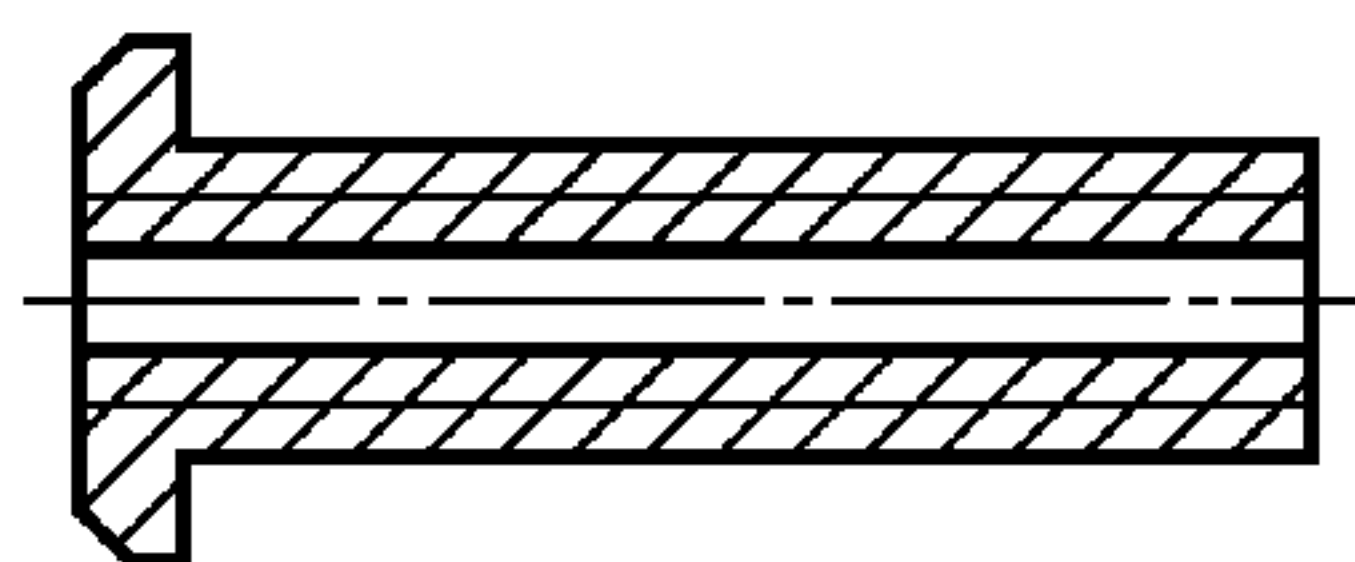
Рисунок Б.2 — Корпус шипа без износостойкого элемента
