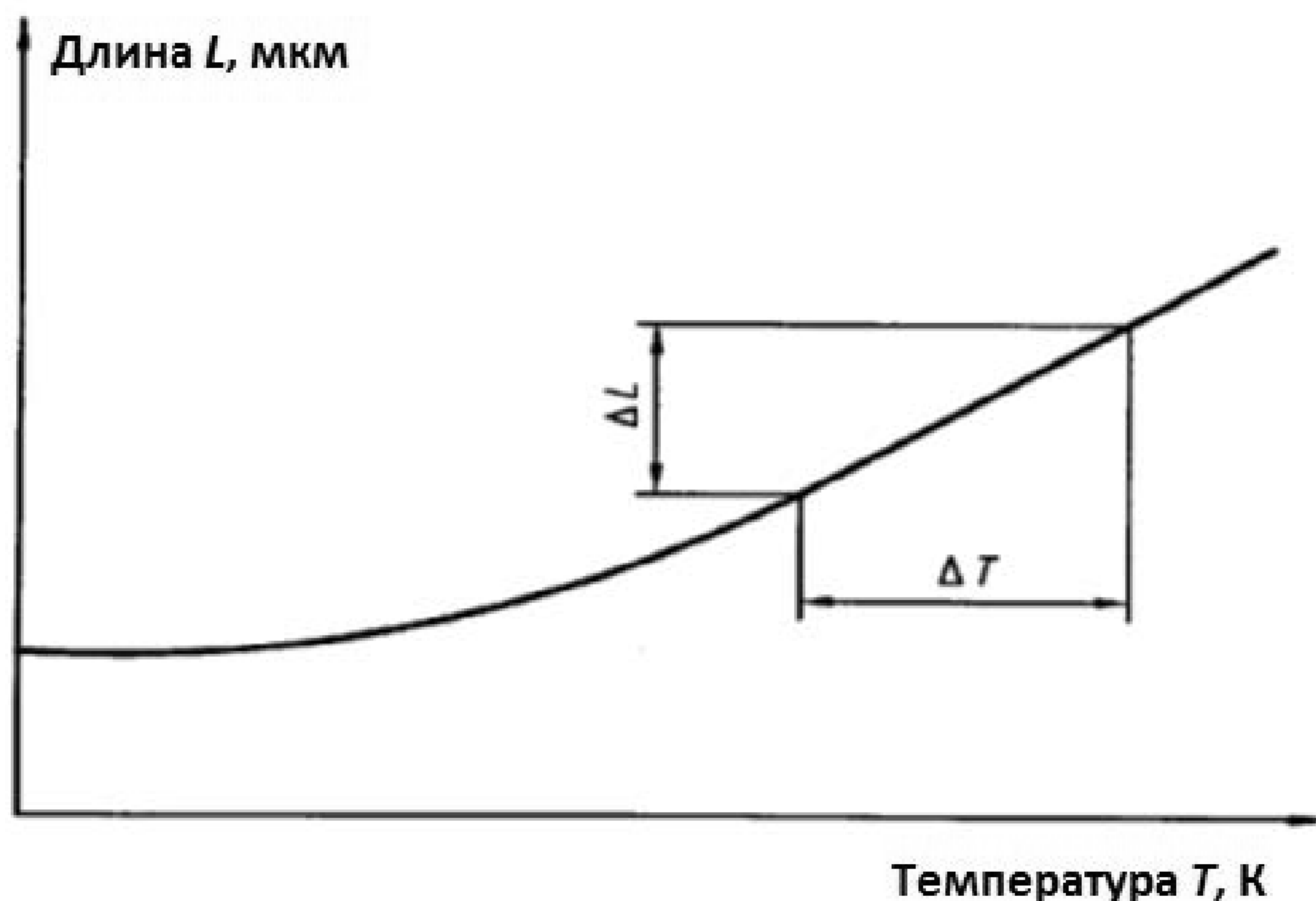
Рисунок 2 – Определение среднего коэффициента линейного теплового расширения \bar{\alpha}
