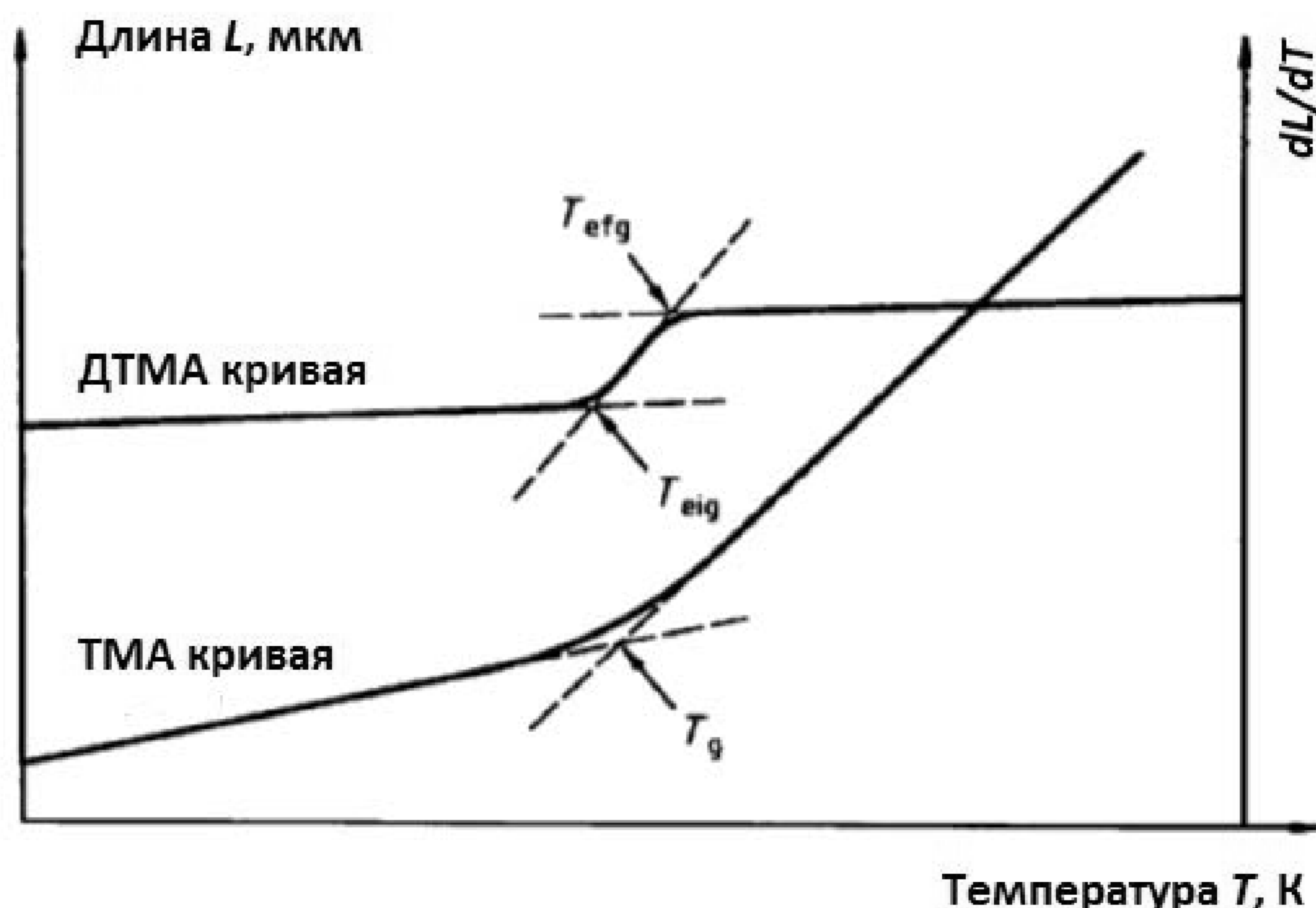
Рисунок 3 – Определение температуры стеклования
