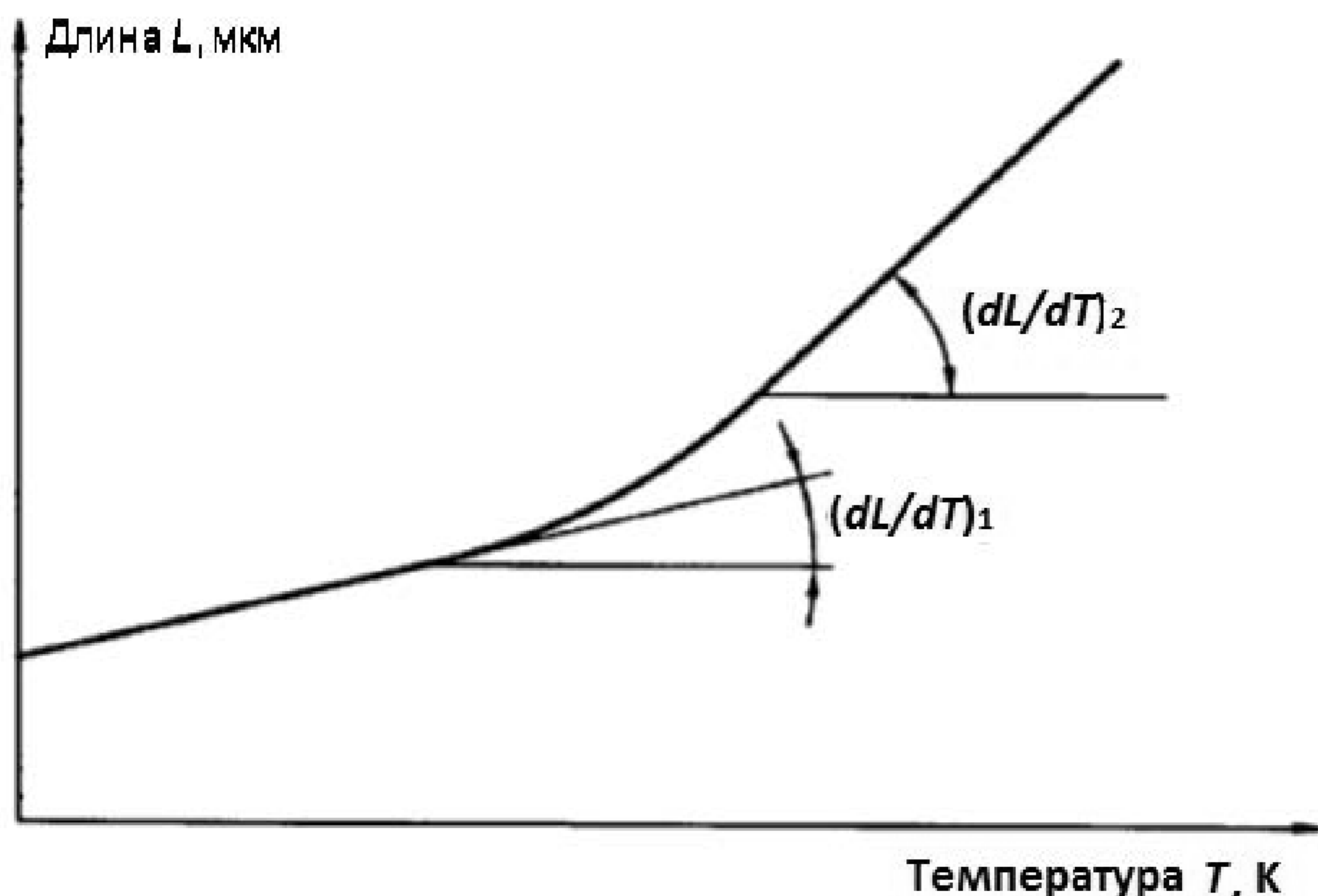
Рисунок 1 – Определение коэффициента линейного теплового расширения
