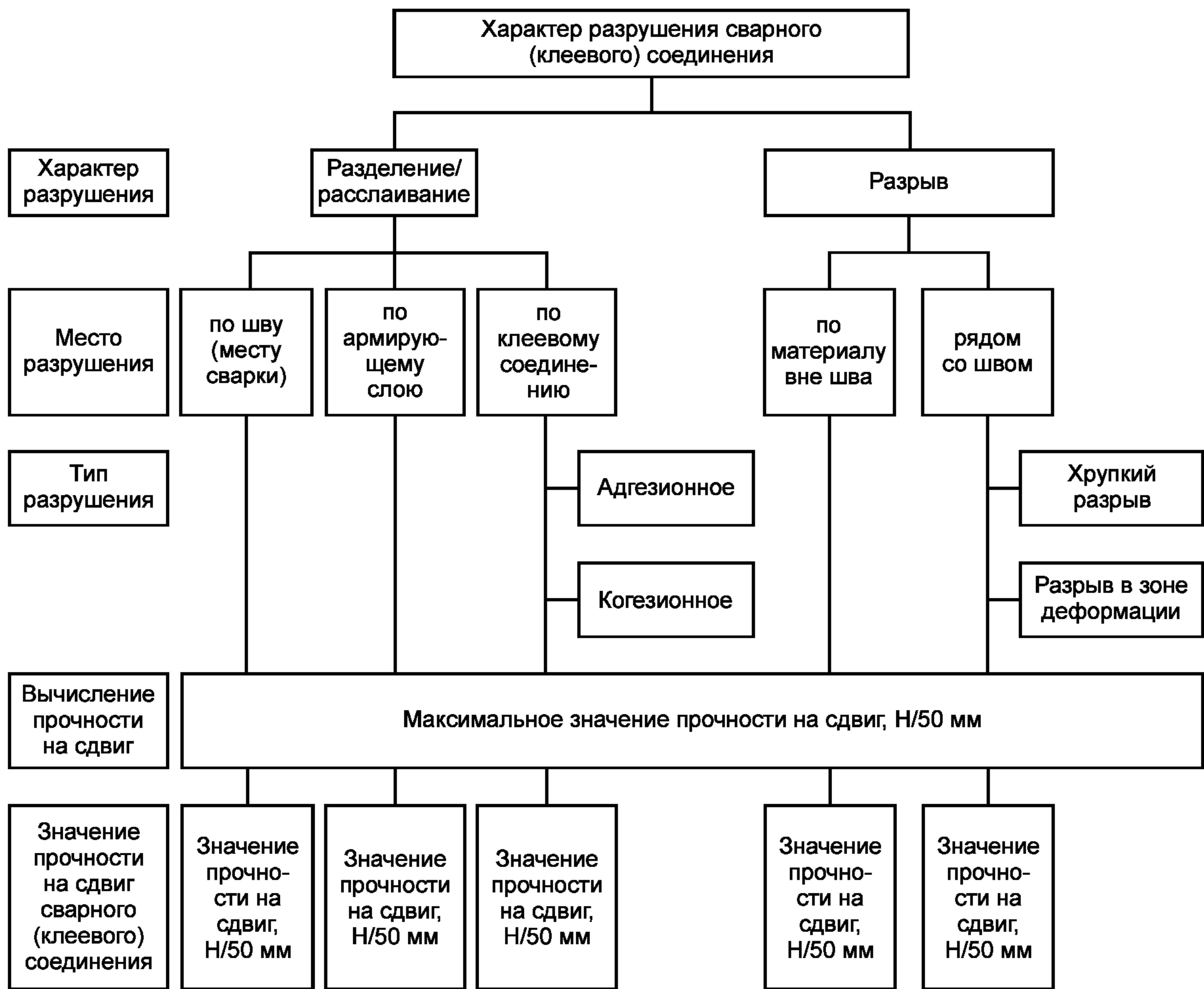
Рисунок А.1 — Характер разрушения сварного (клеевого) соединения
