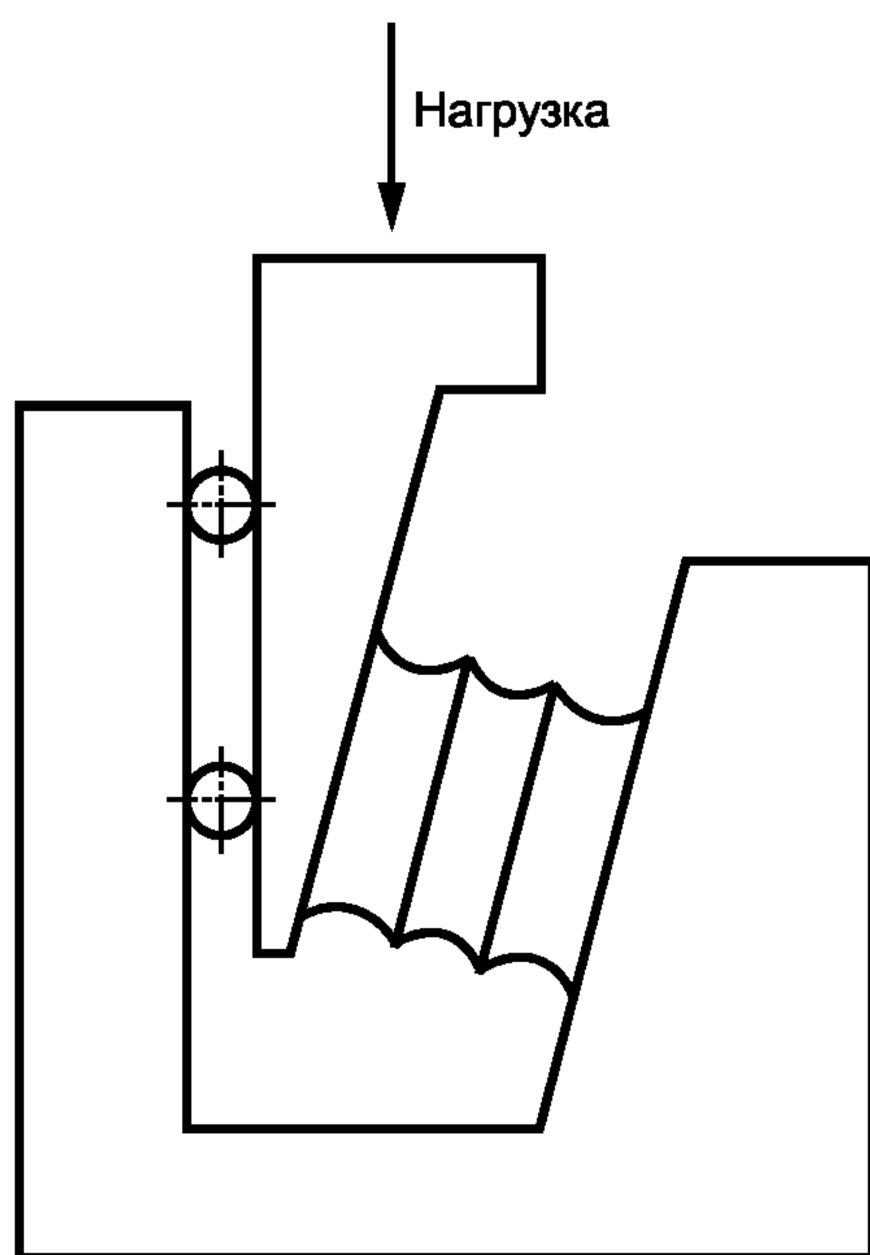
Рисунок 2 — Установка рессоры на стенде
