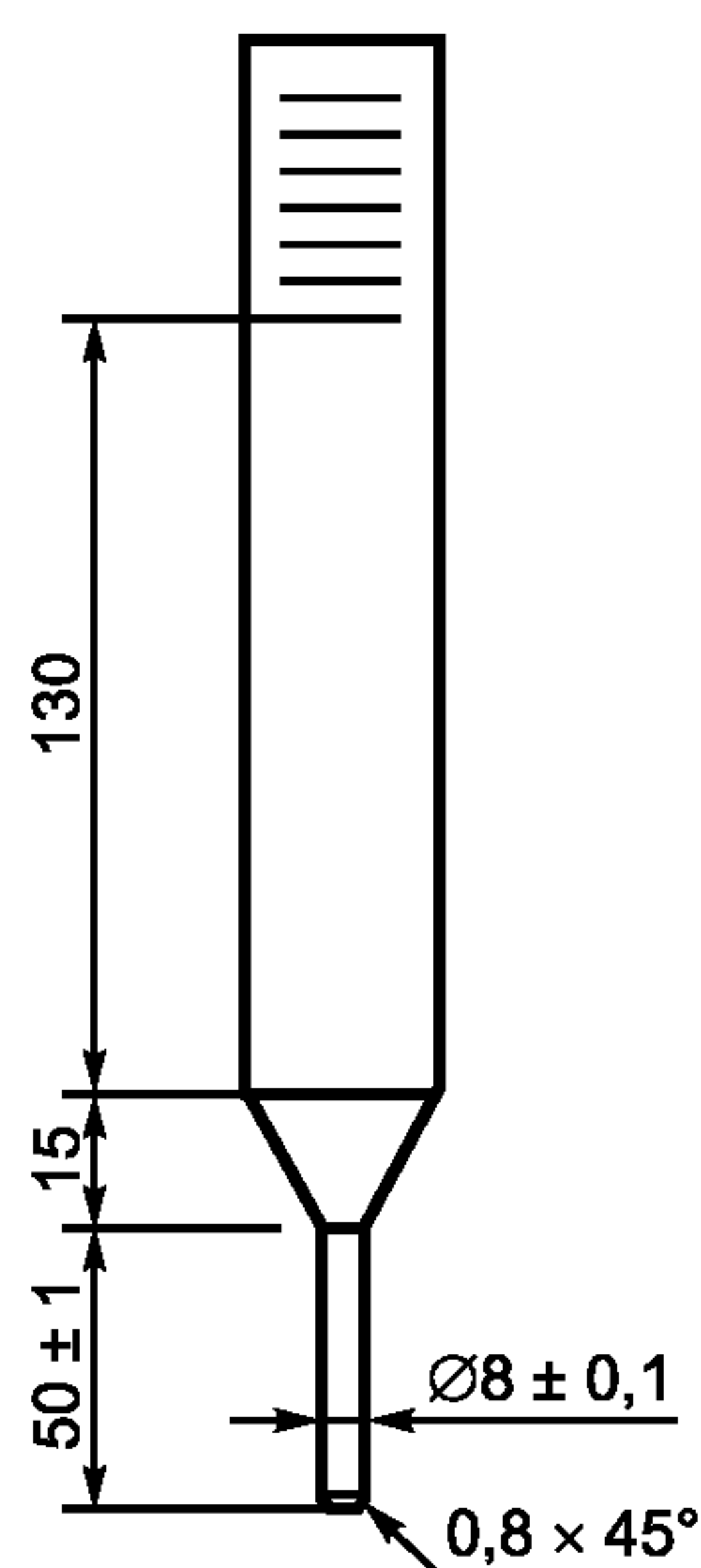
Рисунок 2 — Стальной цилиндрический штамп
