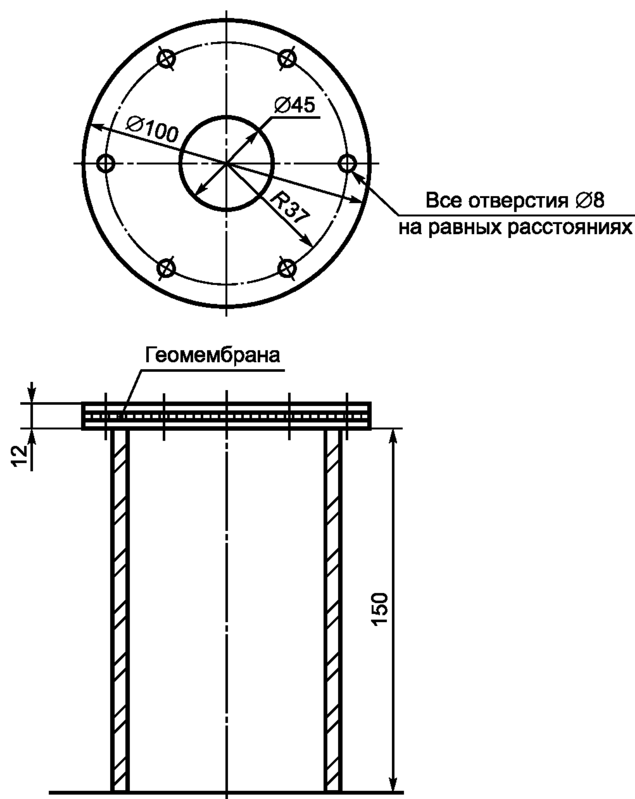
Рисунок 3 — Кольцевой зажим
