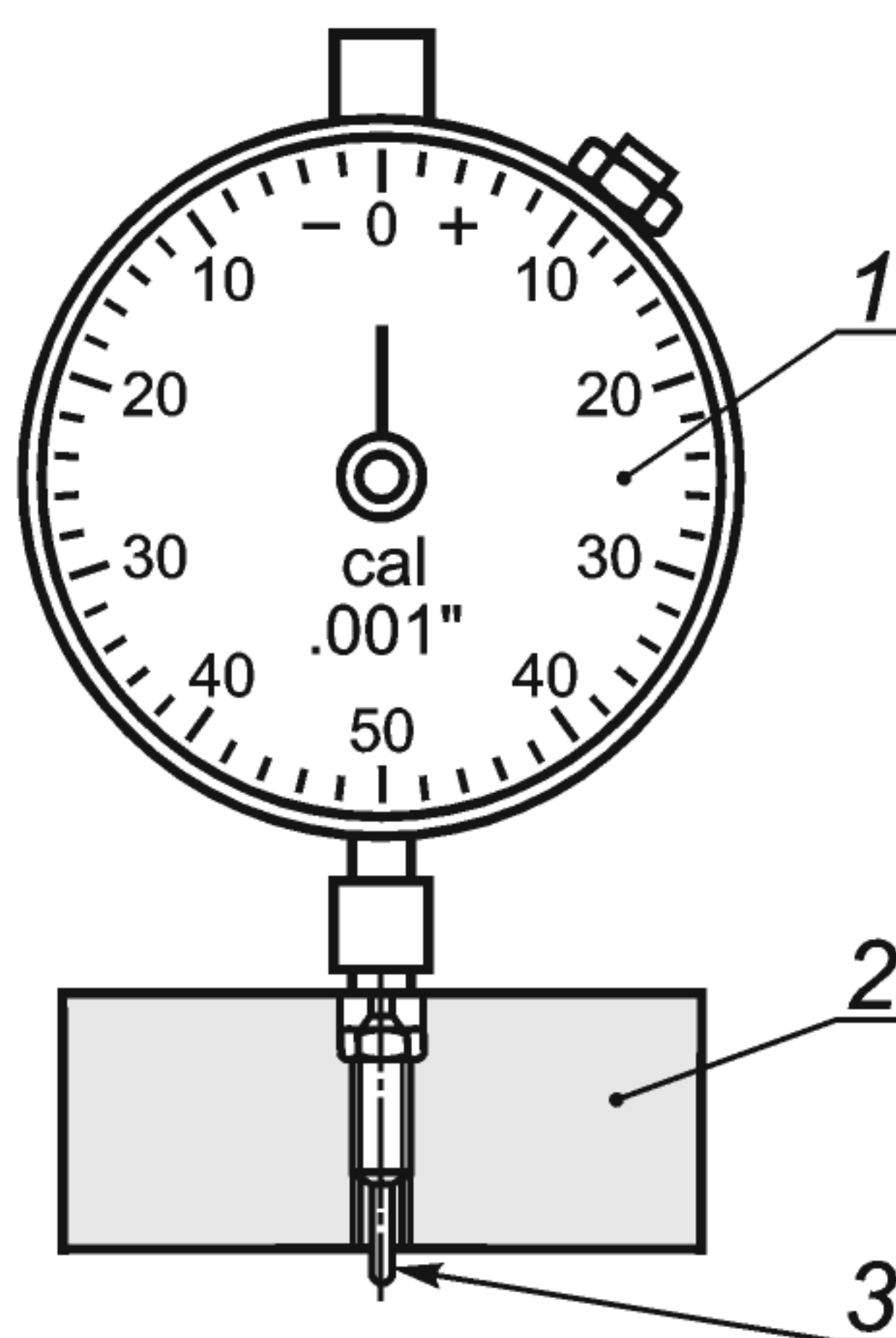
1 — индикатор; 2 — установочный блок; 3 — металлический стержень
