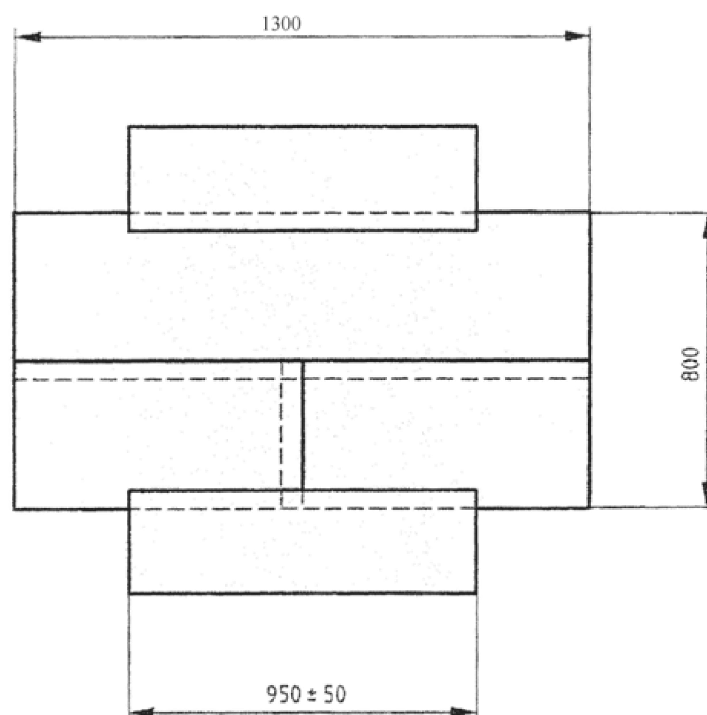
Рисунок 2 – Расположение швов в испытуемом образце
