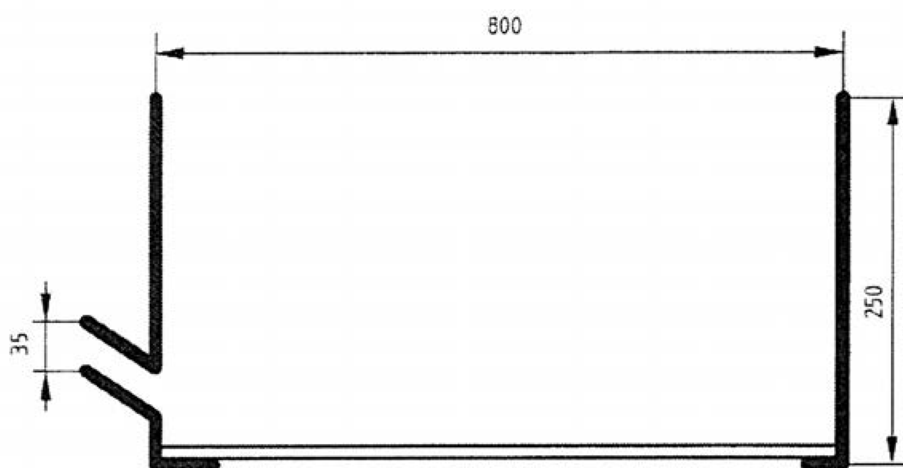
Рисунок 1 – Конструкция контейнера
