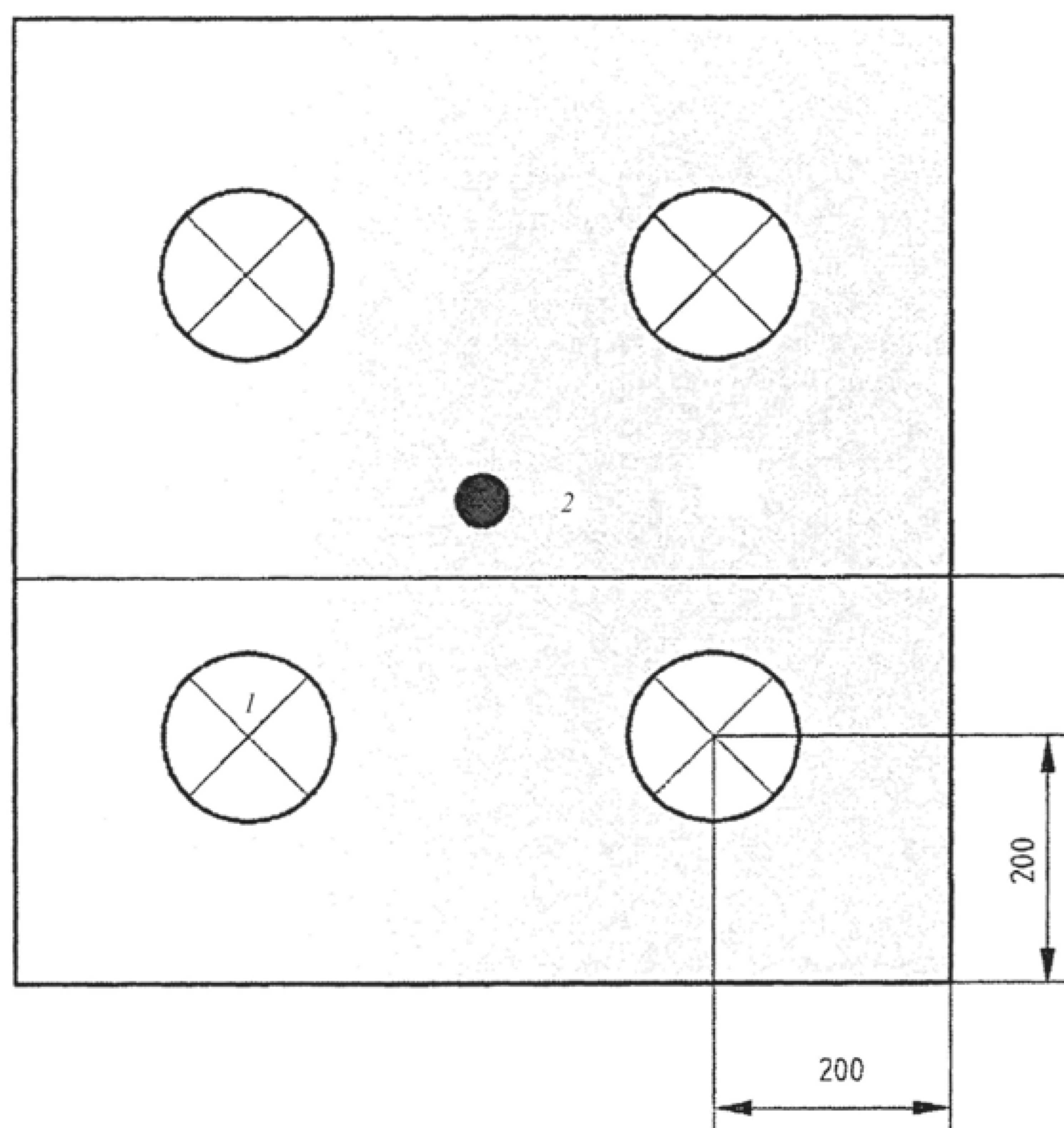
1 – испытуемый образец; 2 – тензиометр
