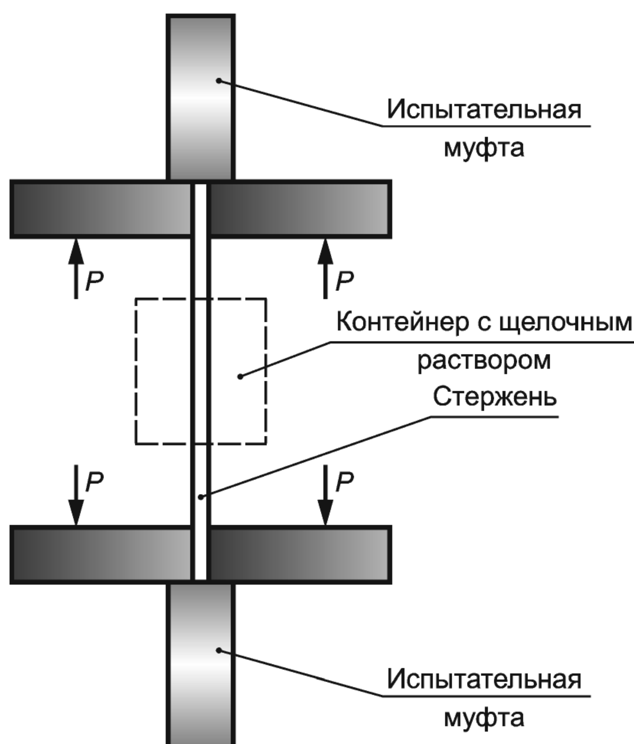
Рисунок 6.1 — Схема испытания образцов на длительную прочность
