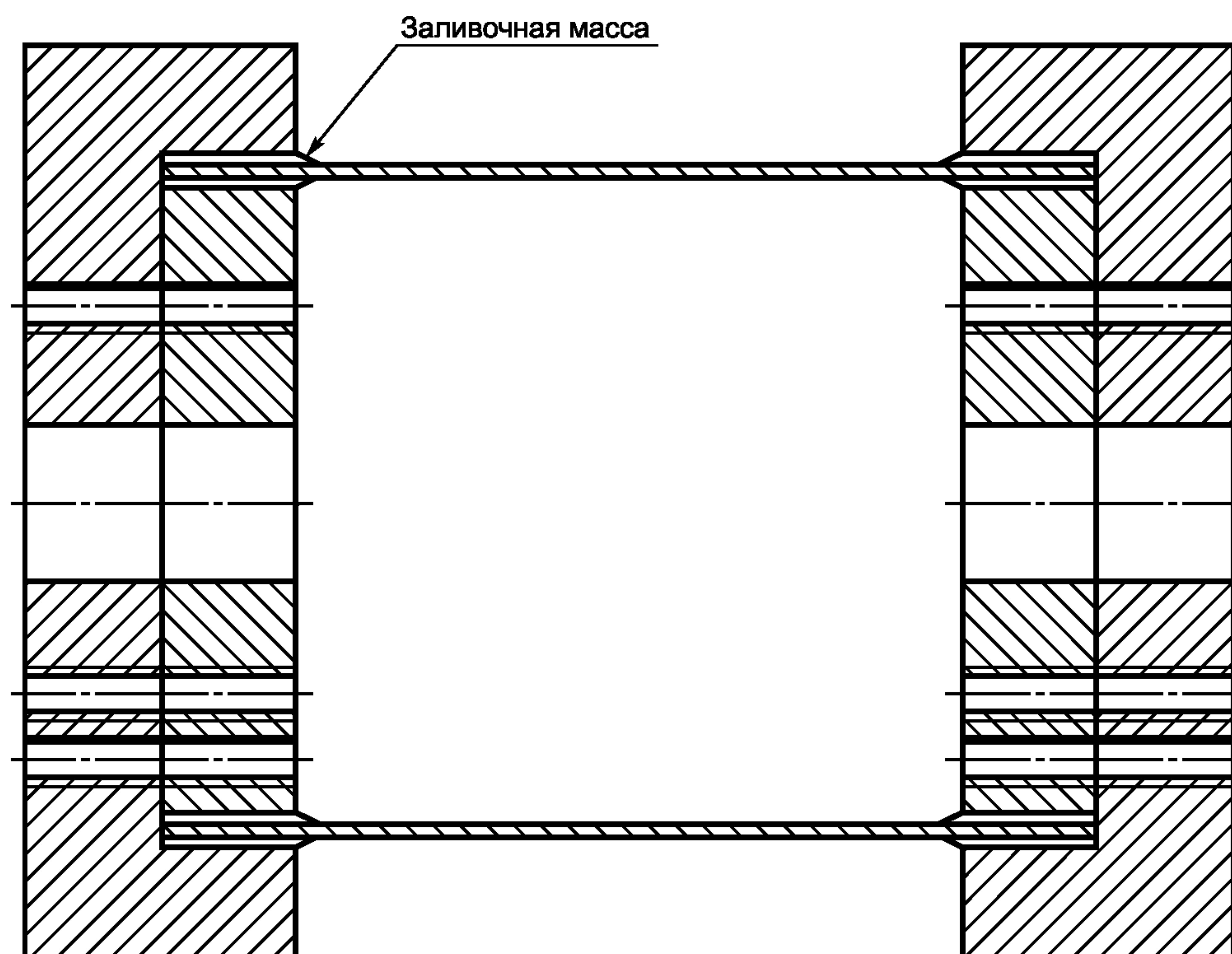
Рисунок 3 — Образец ПКМ, закрепленный в приспособлении для сжатия
