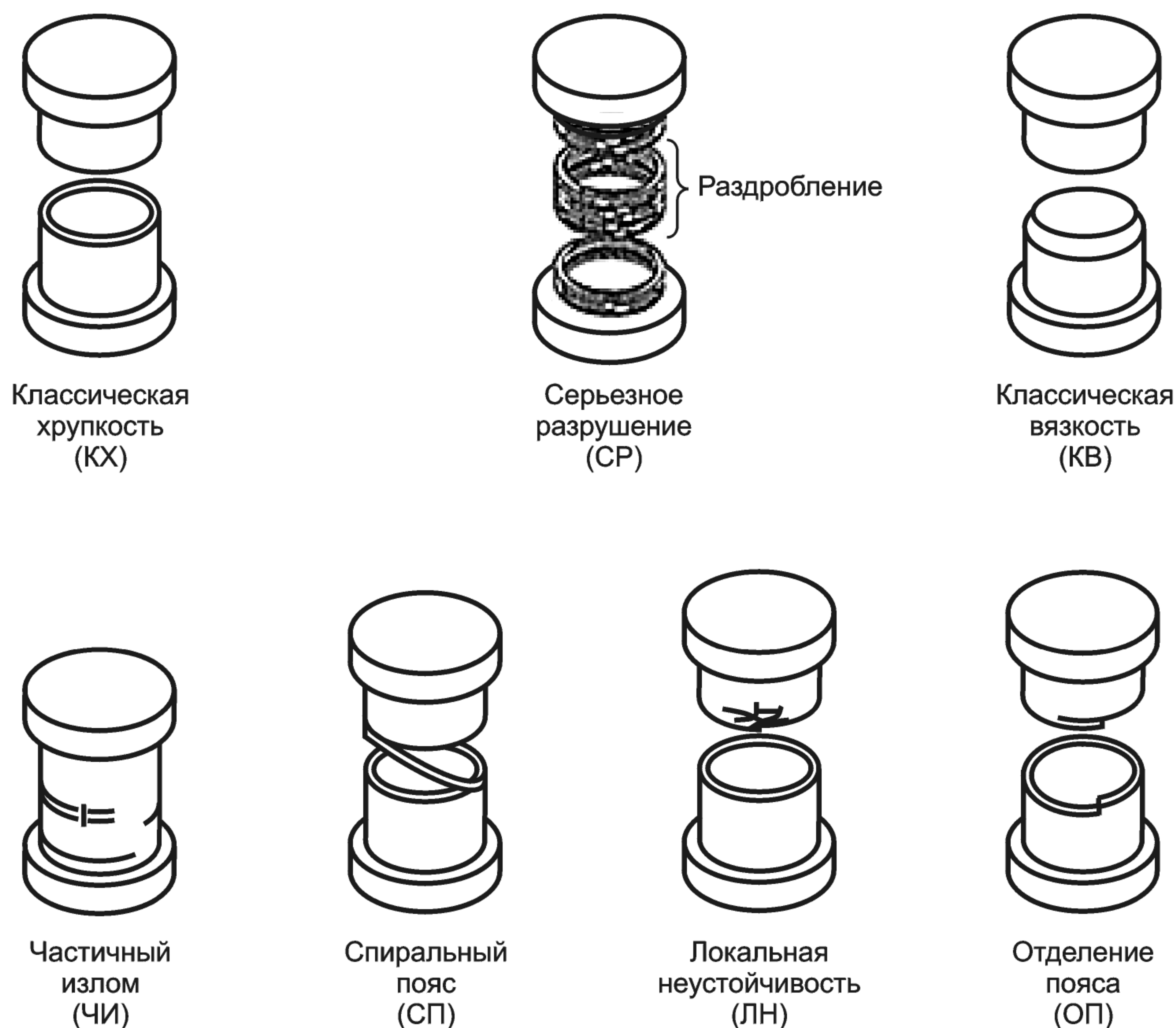
Рисунок 4 — Виды разрушения образцов кольцевой намотки при сжатии
