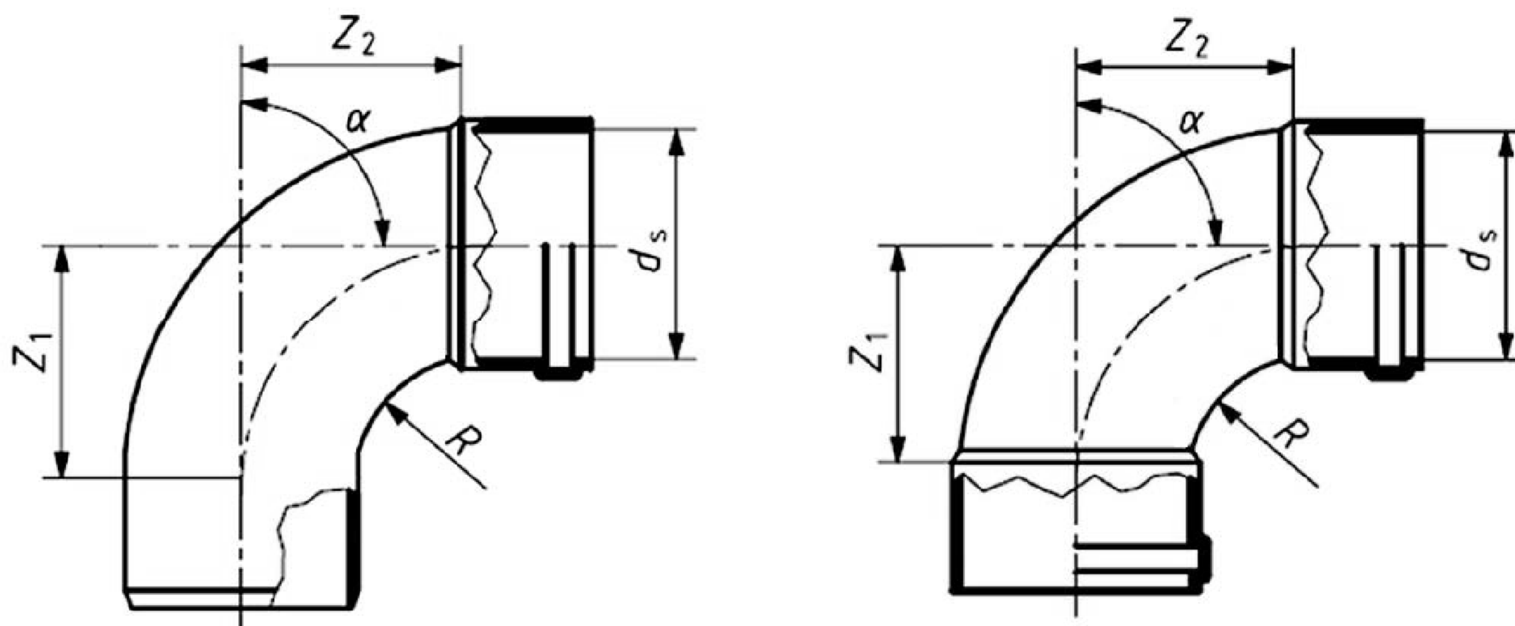
Рисунок 6 – Отвод
