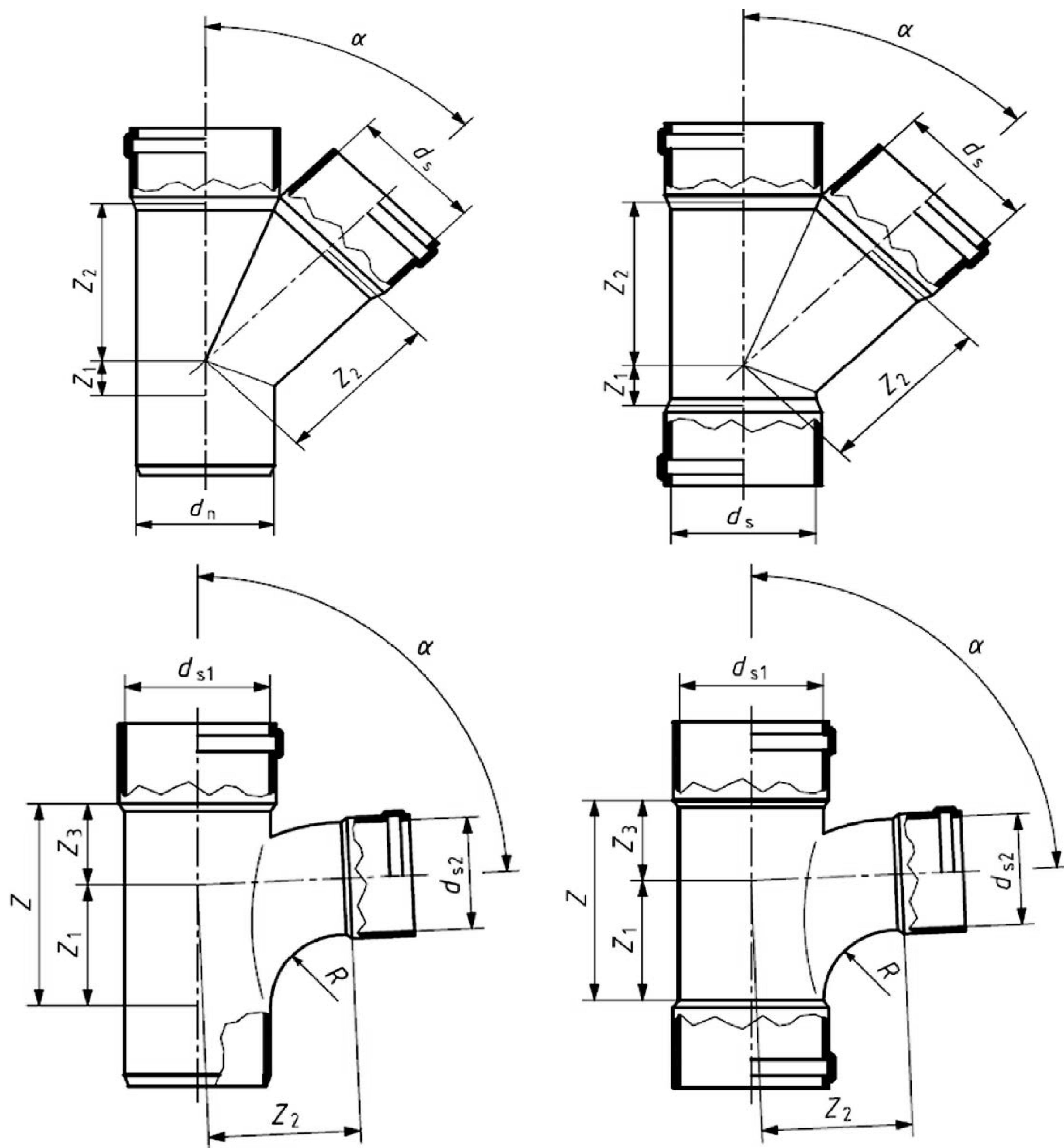
Рисунок 9 – Тройник
