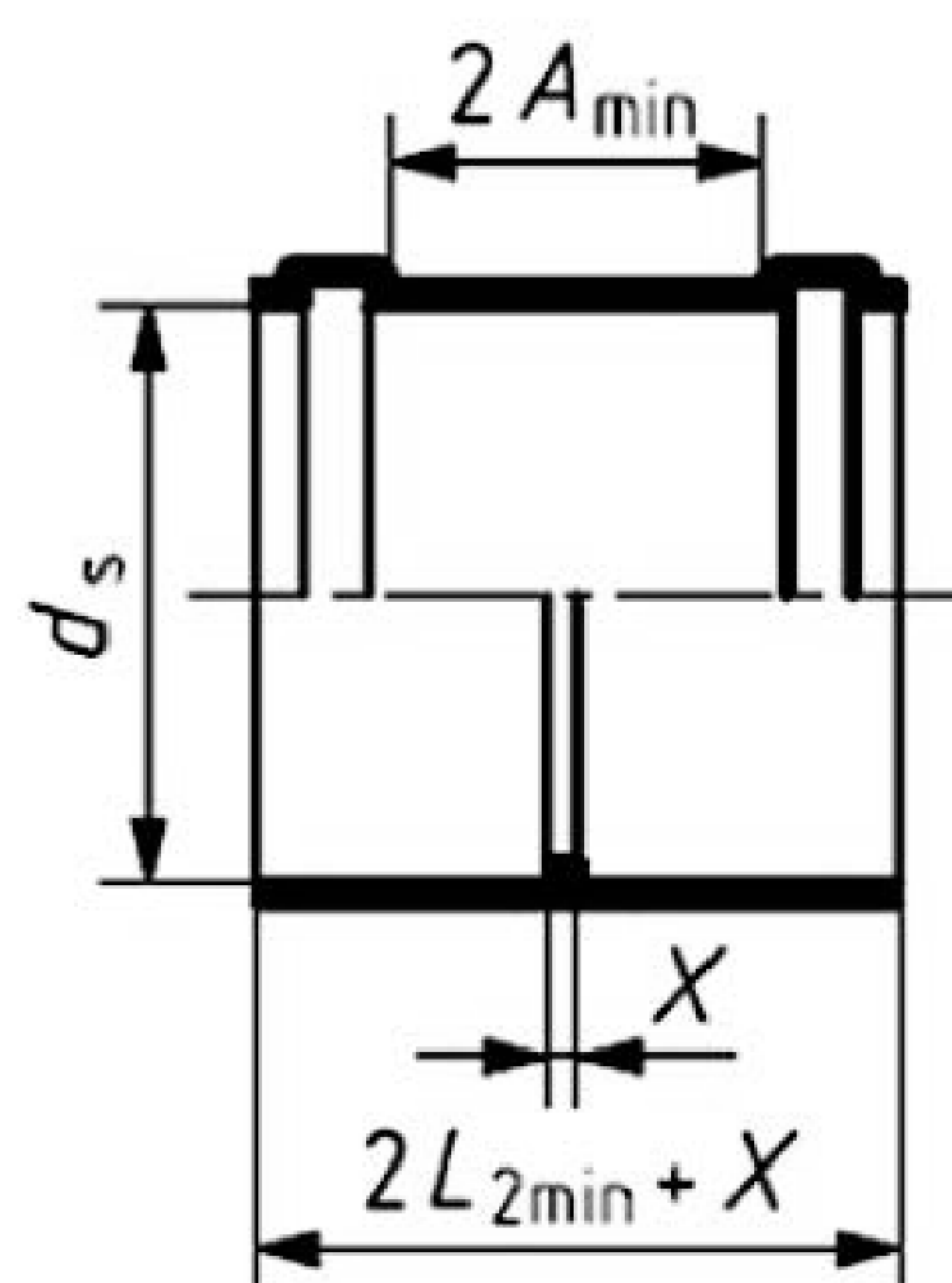
Рисунок 7 – Муфта
