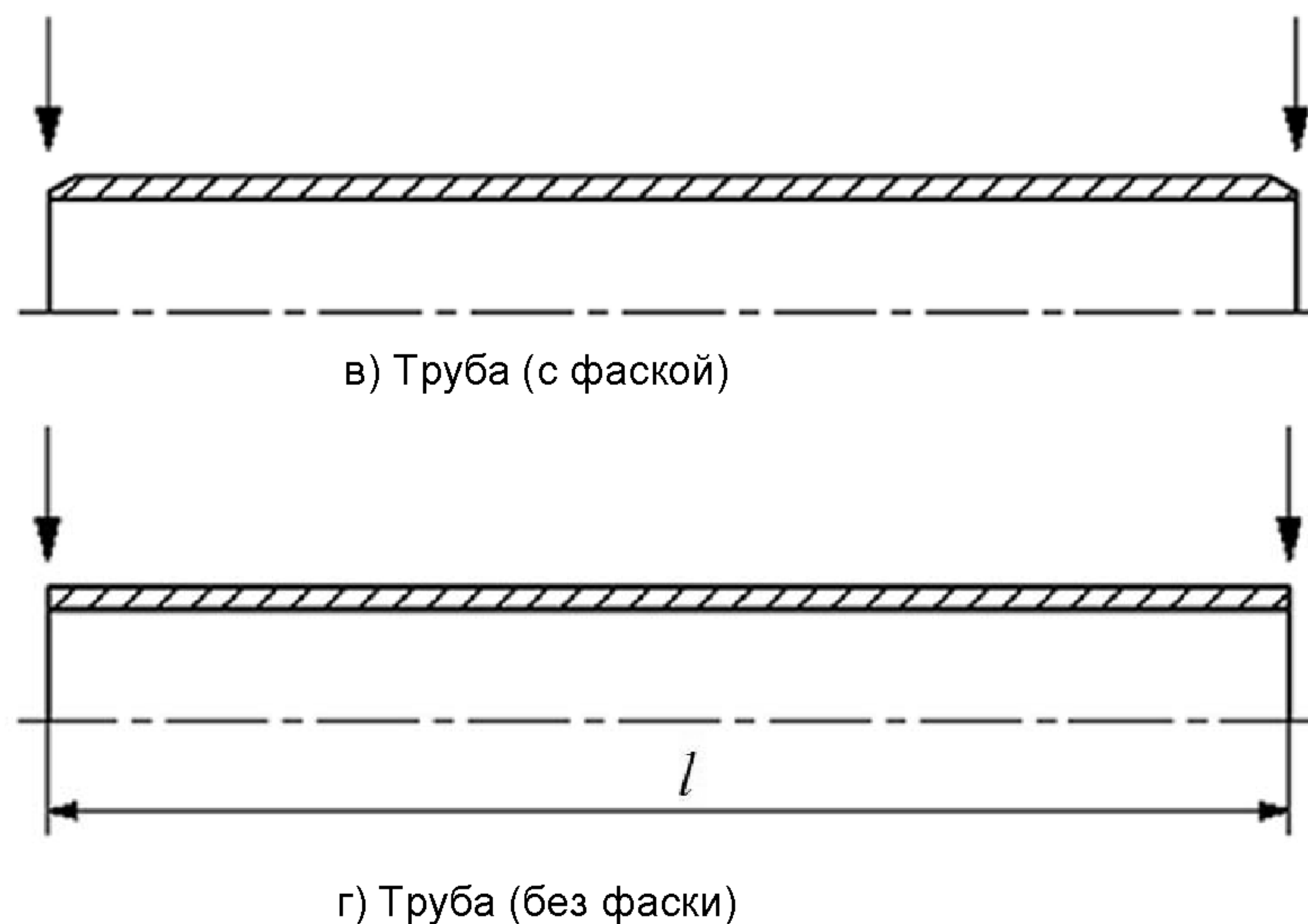
Рисунок 1 – Эффективная длина труб
