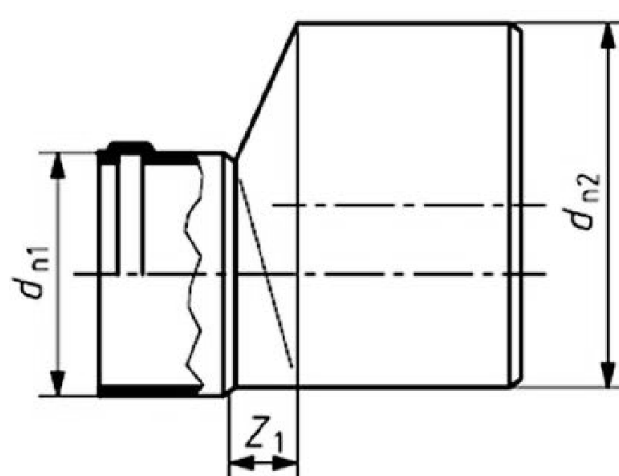
Рисунок 8 – Патрубок переходной
