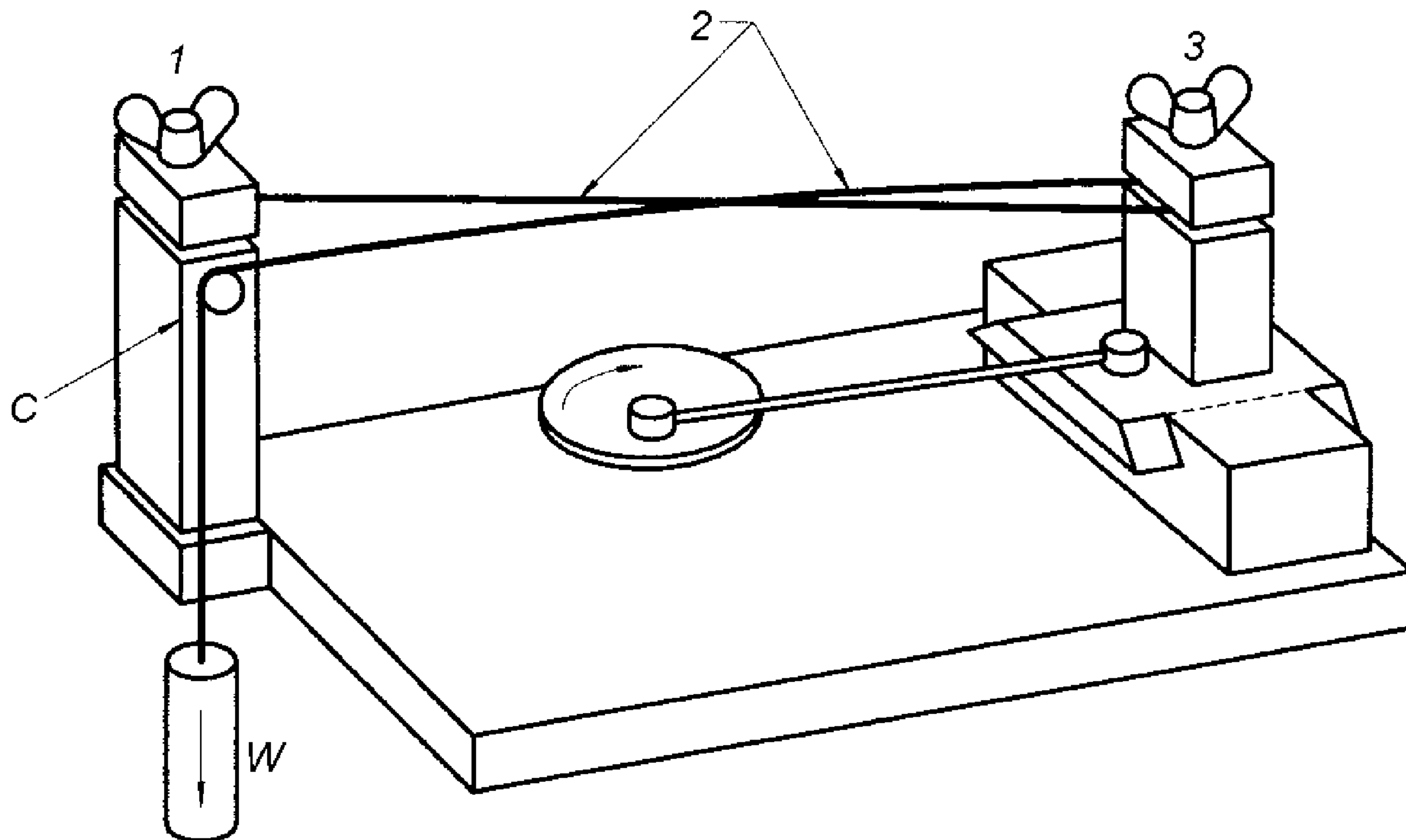
Рисунок В.1 – Машина для истирания шнурков
