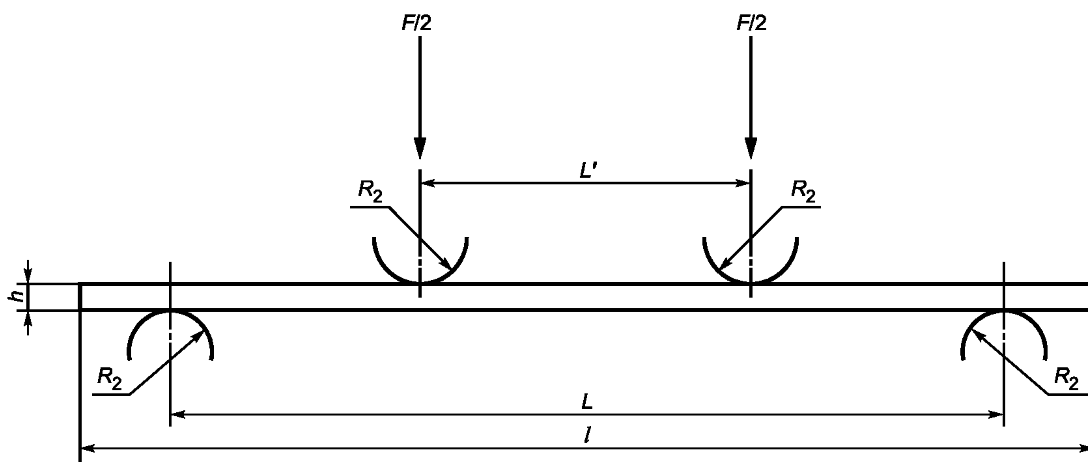
Рисунок 2 — Схема трехточечного нагружения
