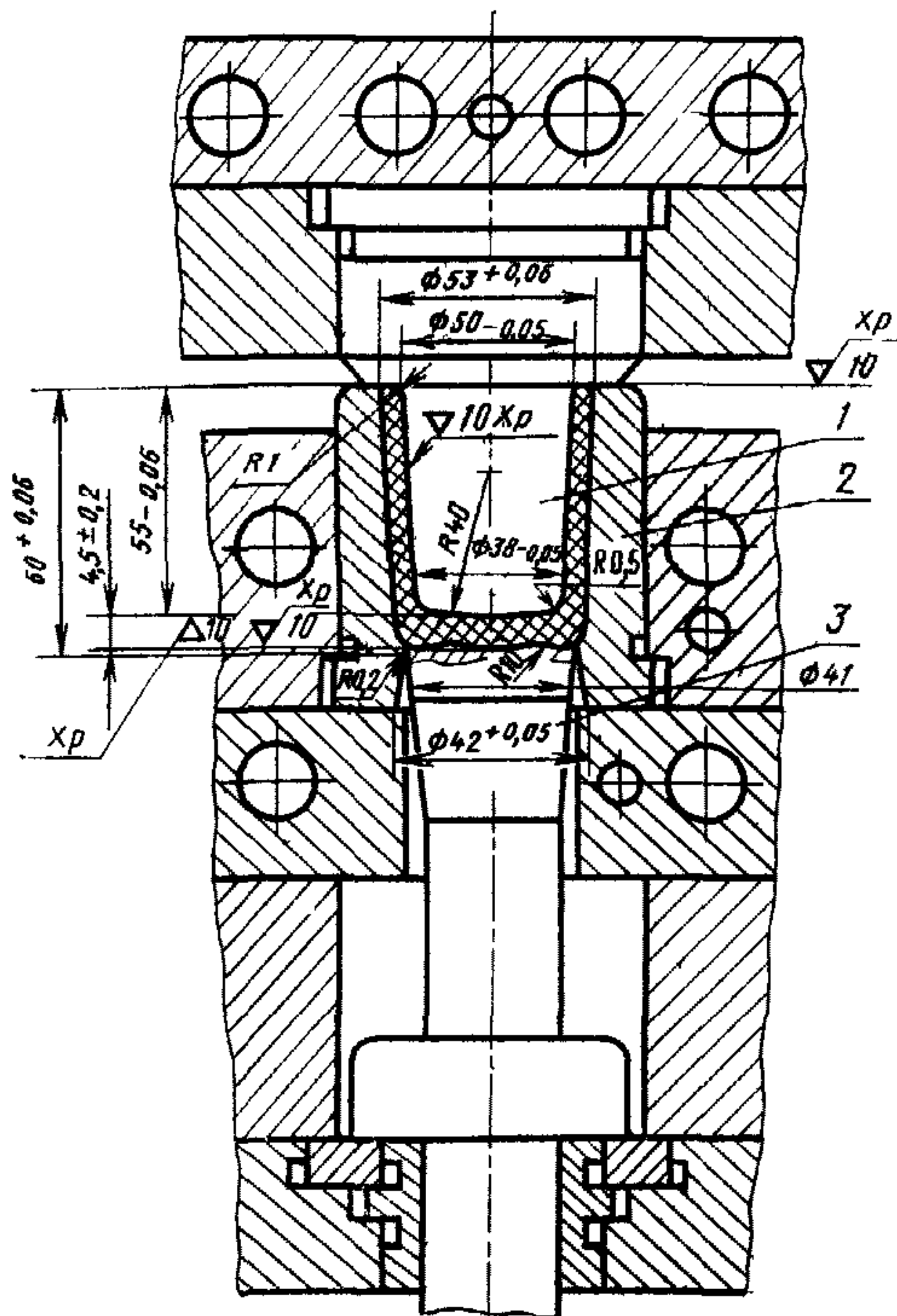
1—пуансон; 2—матрица; 3—выталкиватель
