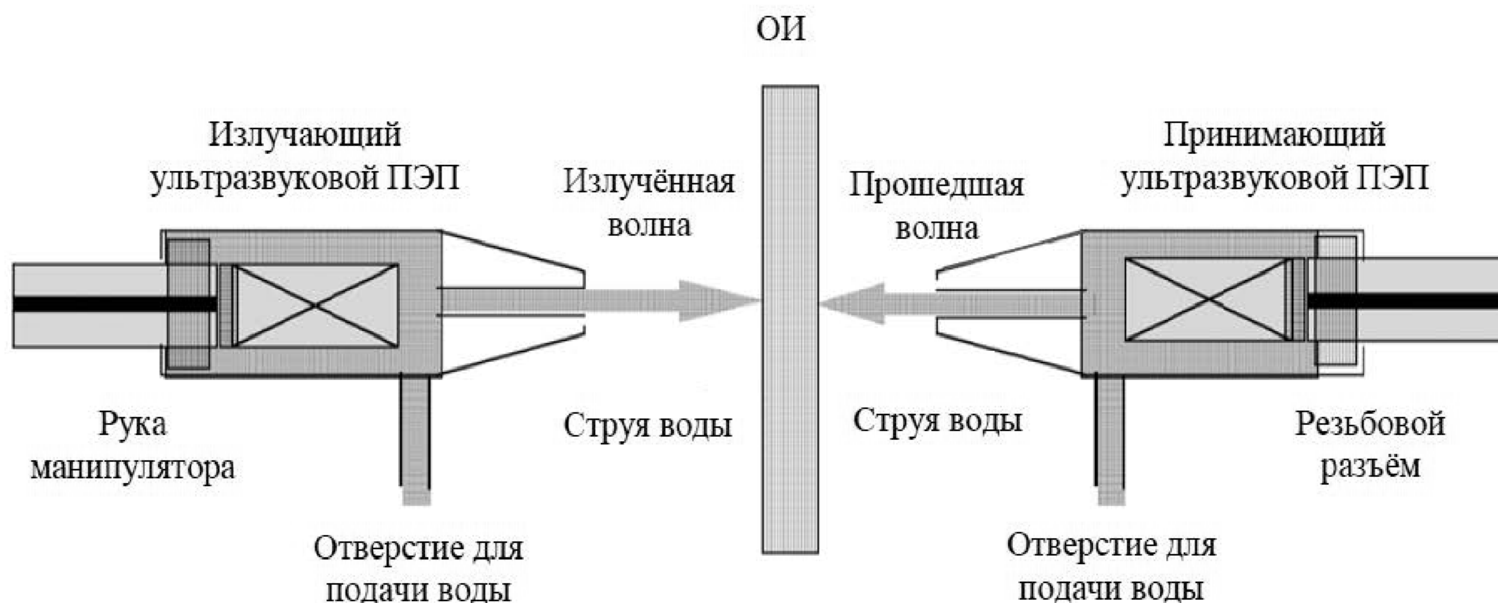
Рисунок 3 — Метод Б. Автоматизированный теневой метод со струйным контактом
