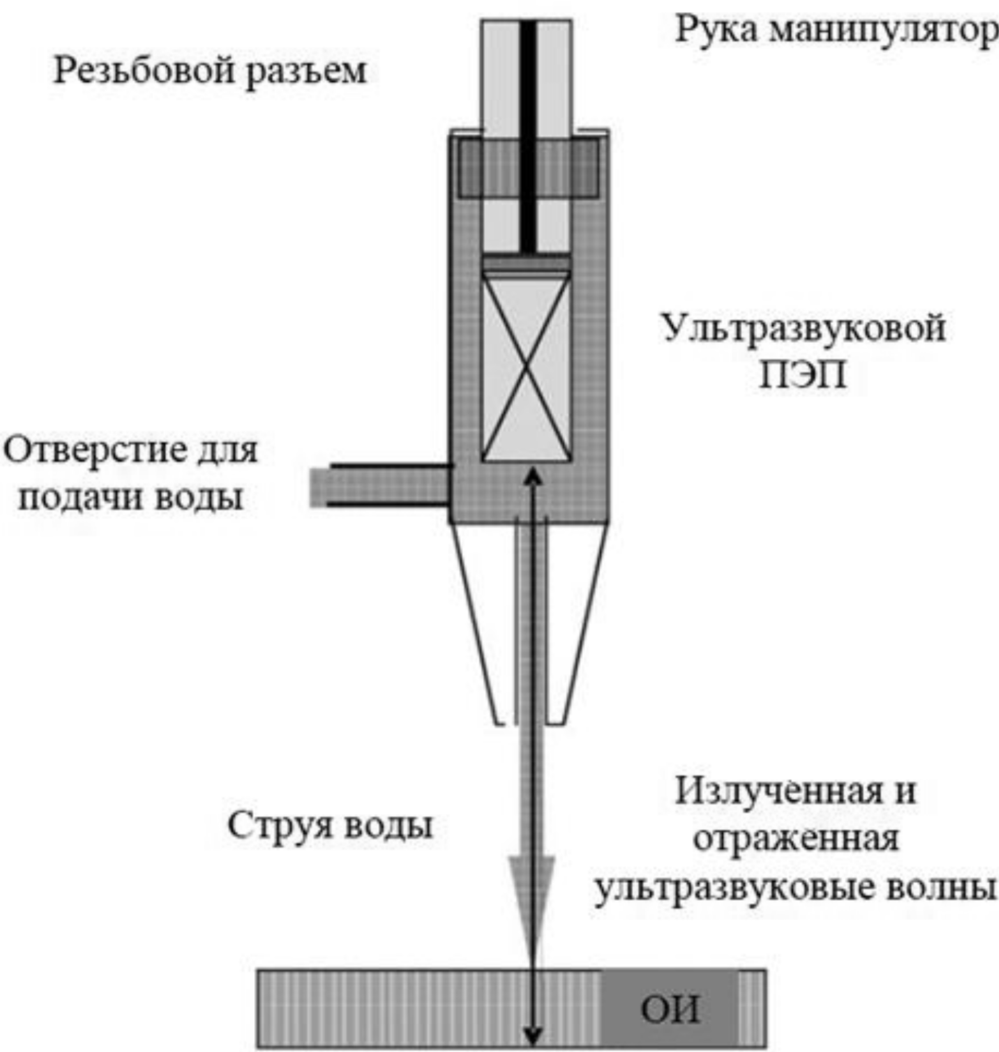
Рисунок 1 — Метод А. Автоматизированный ультразвуковой эхо-импульсный метод
