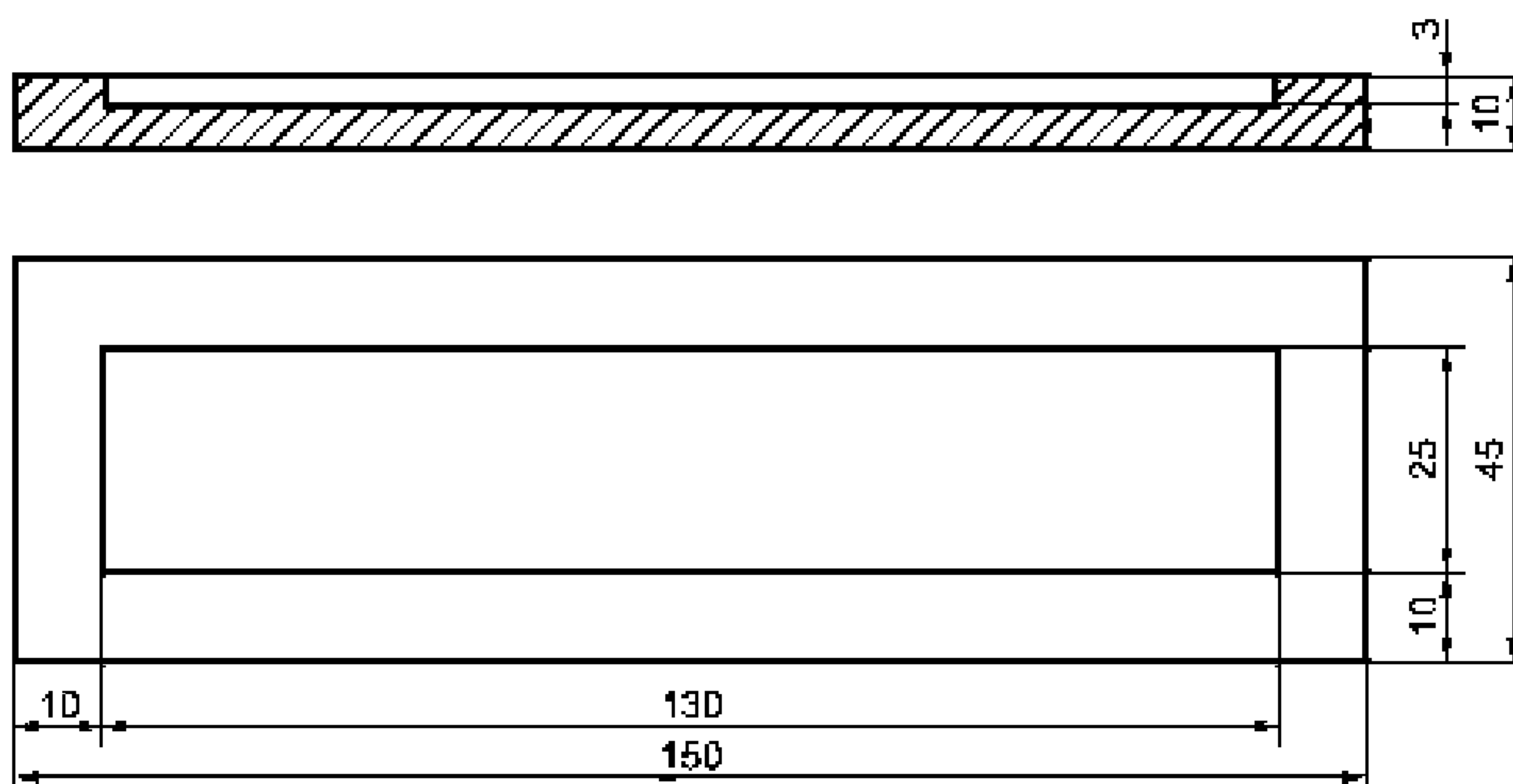
Рисунок 3 — Лоток для определения рабочего времени оттискового материала
