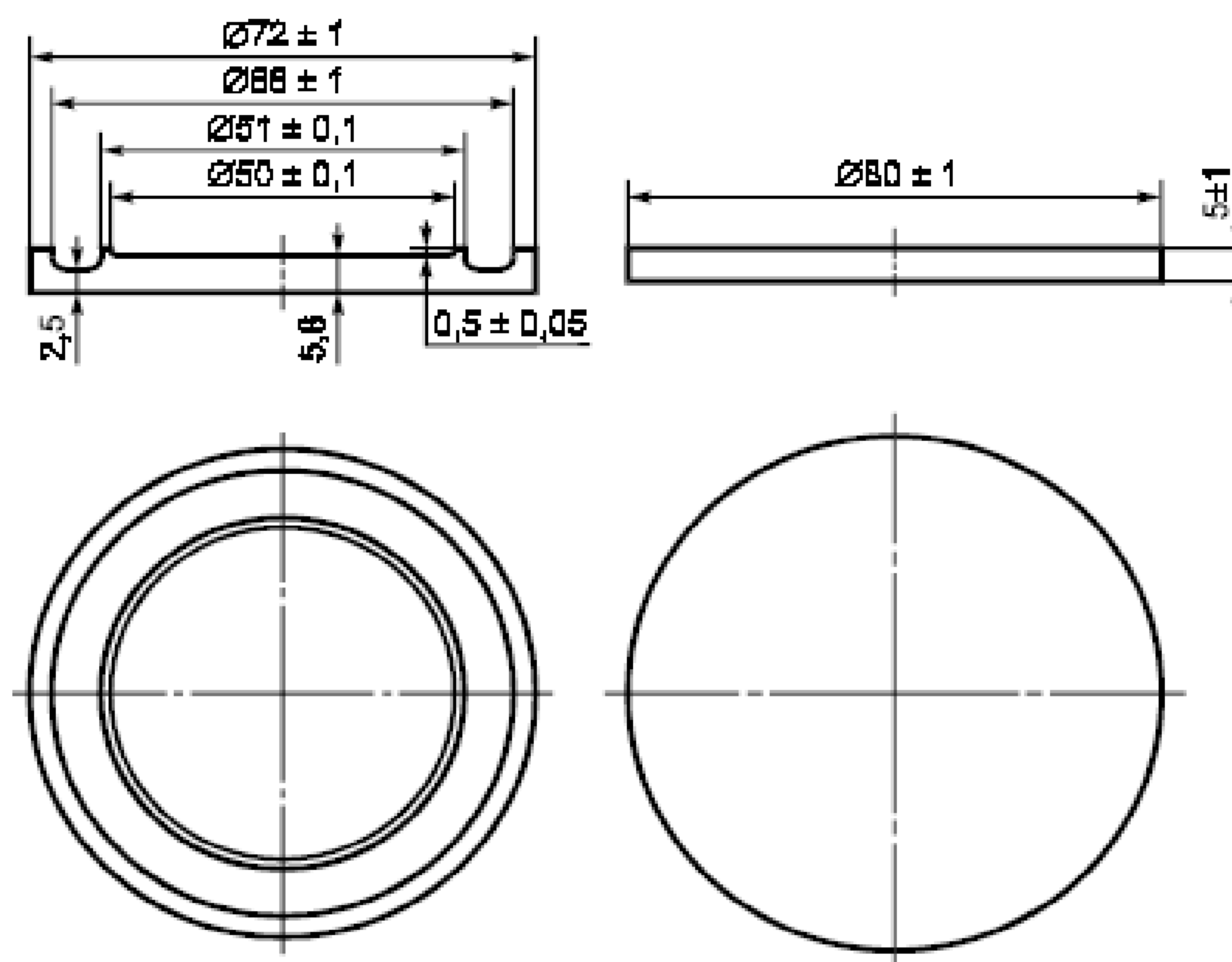
1 — форма; 2 — крышка
