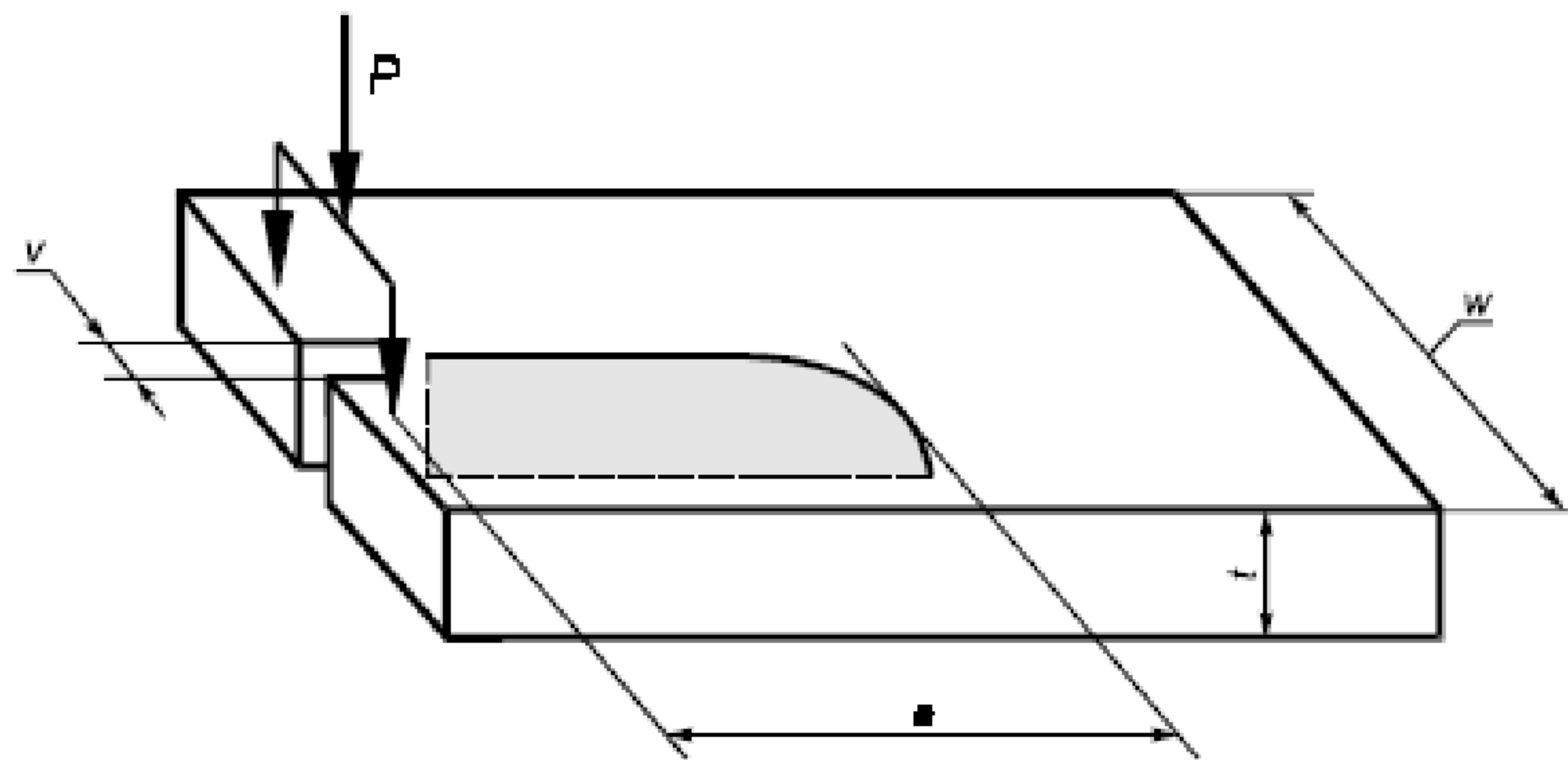
a – Схема испытания
