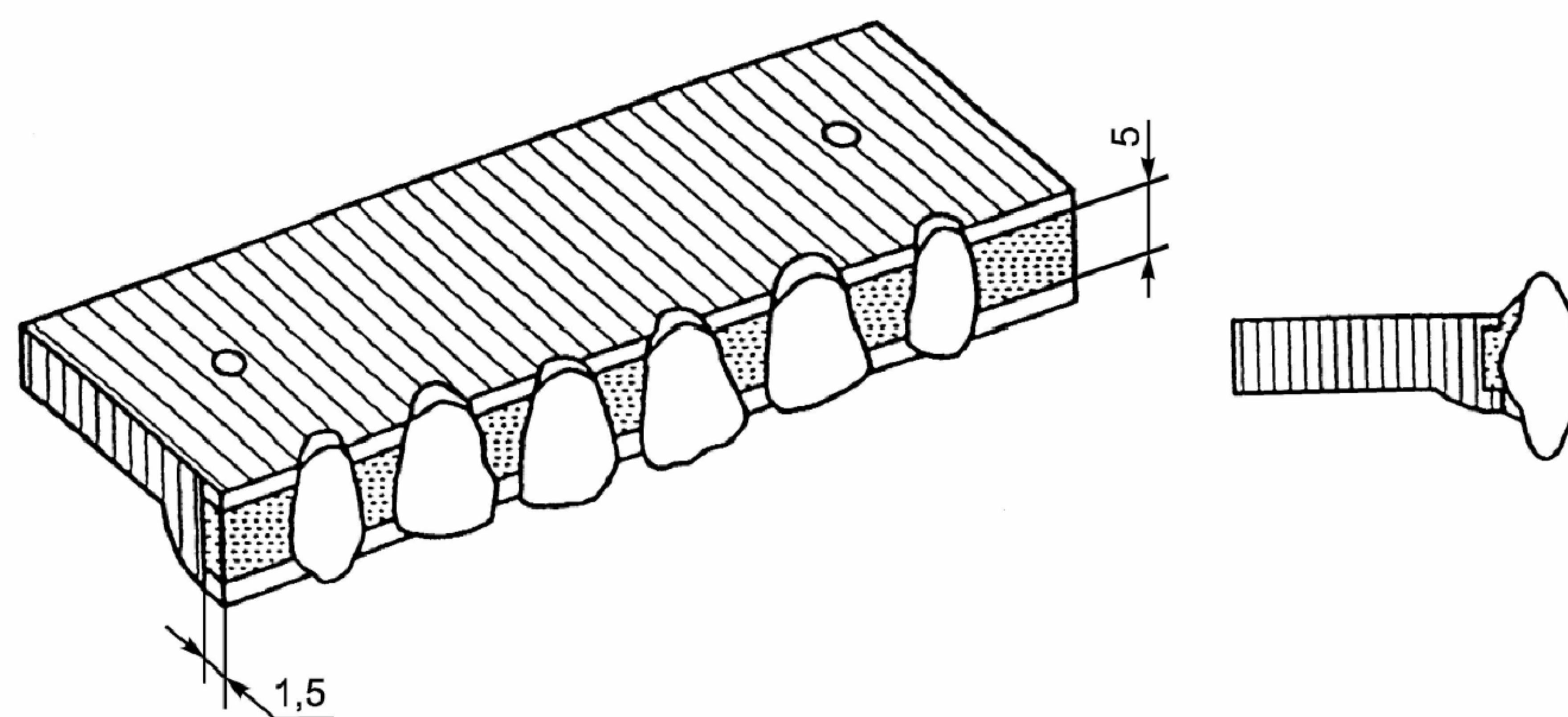
а - Металлическая форма для монтирования зубов
