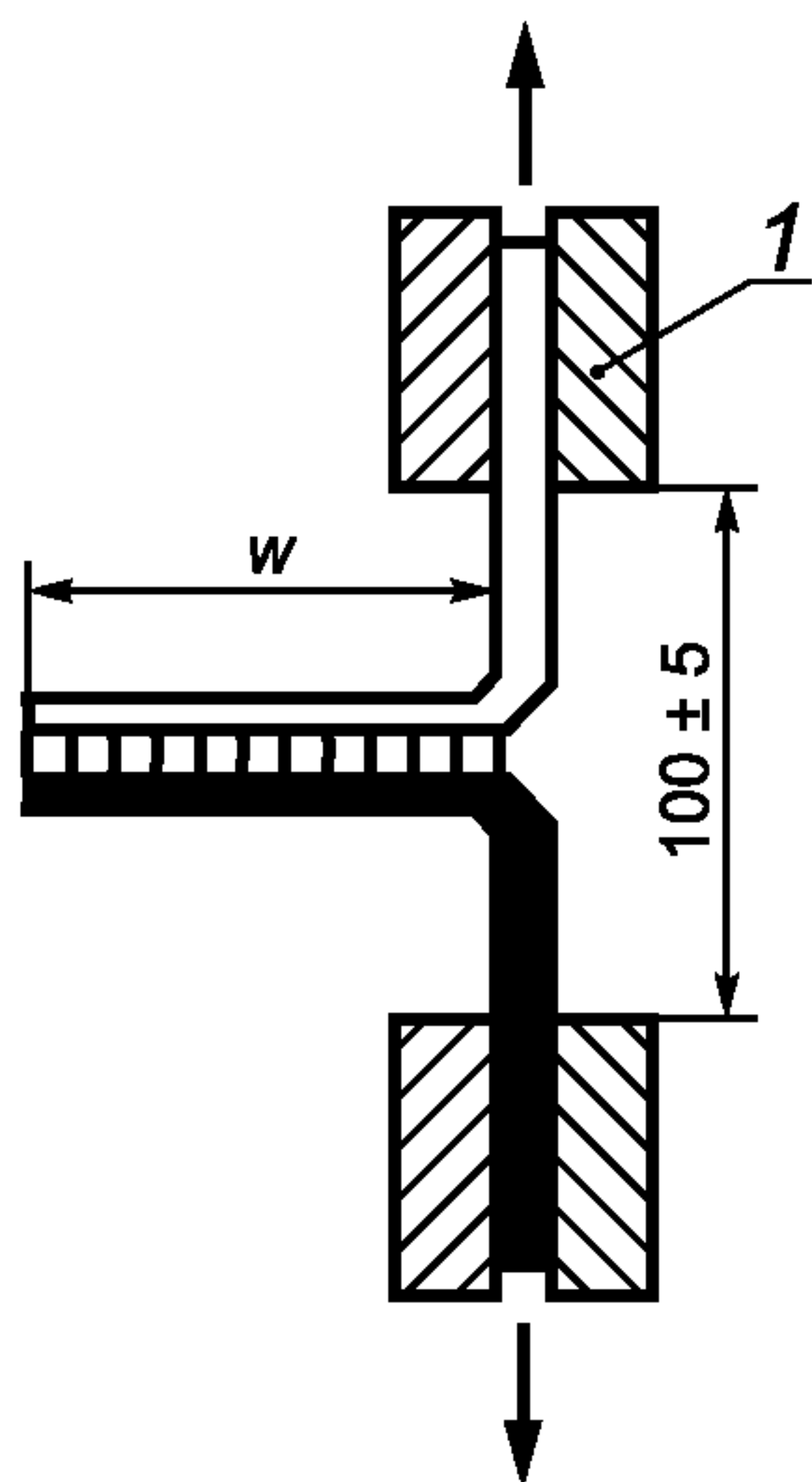
1 — зажим; w — ширина сварного (клеевого) соединения
