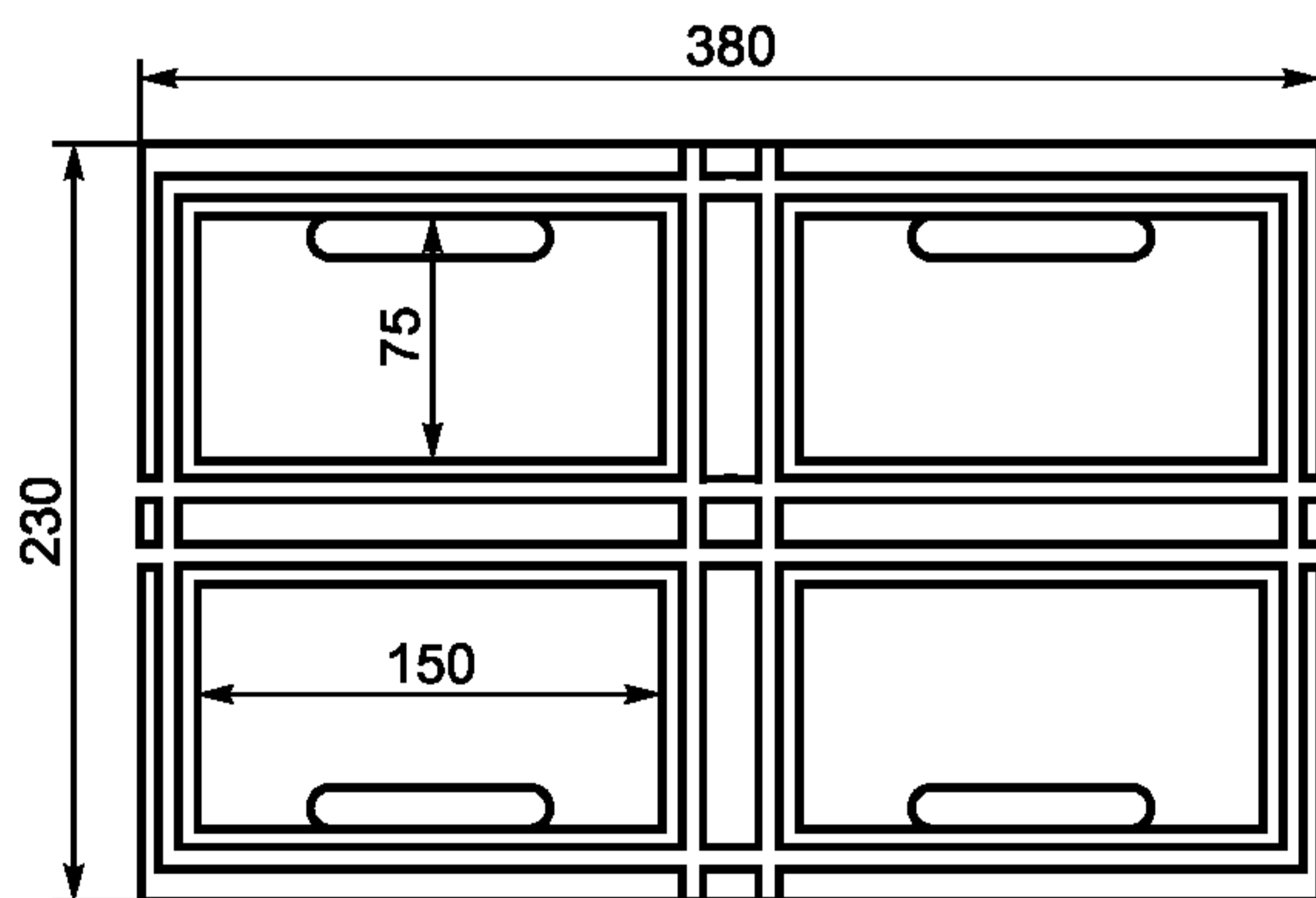
Рисунок 3 — Четырехгнездная пресс-форма для пластин небольшого размера
