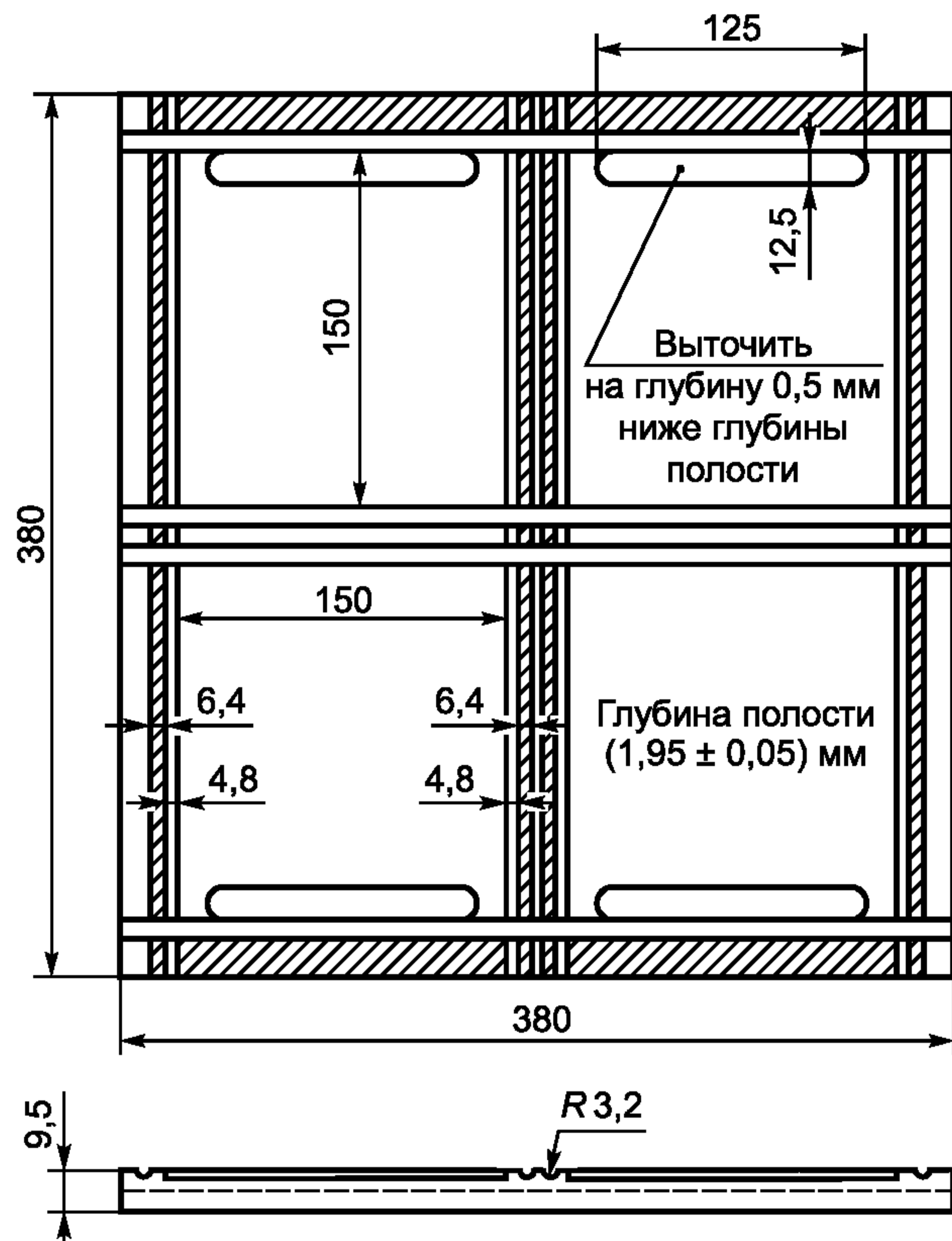
Рисунок 2 — Пресс-форма для гнезд, изготовленных в плите прессы
