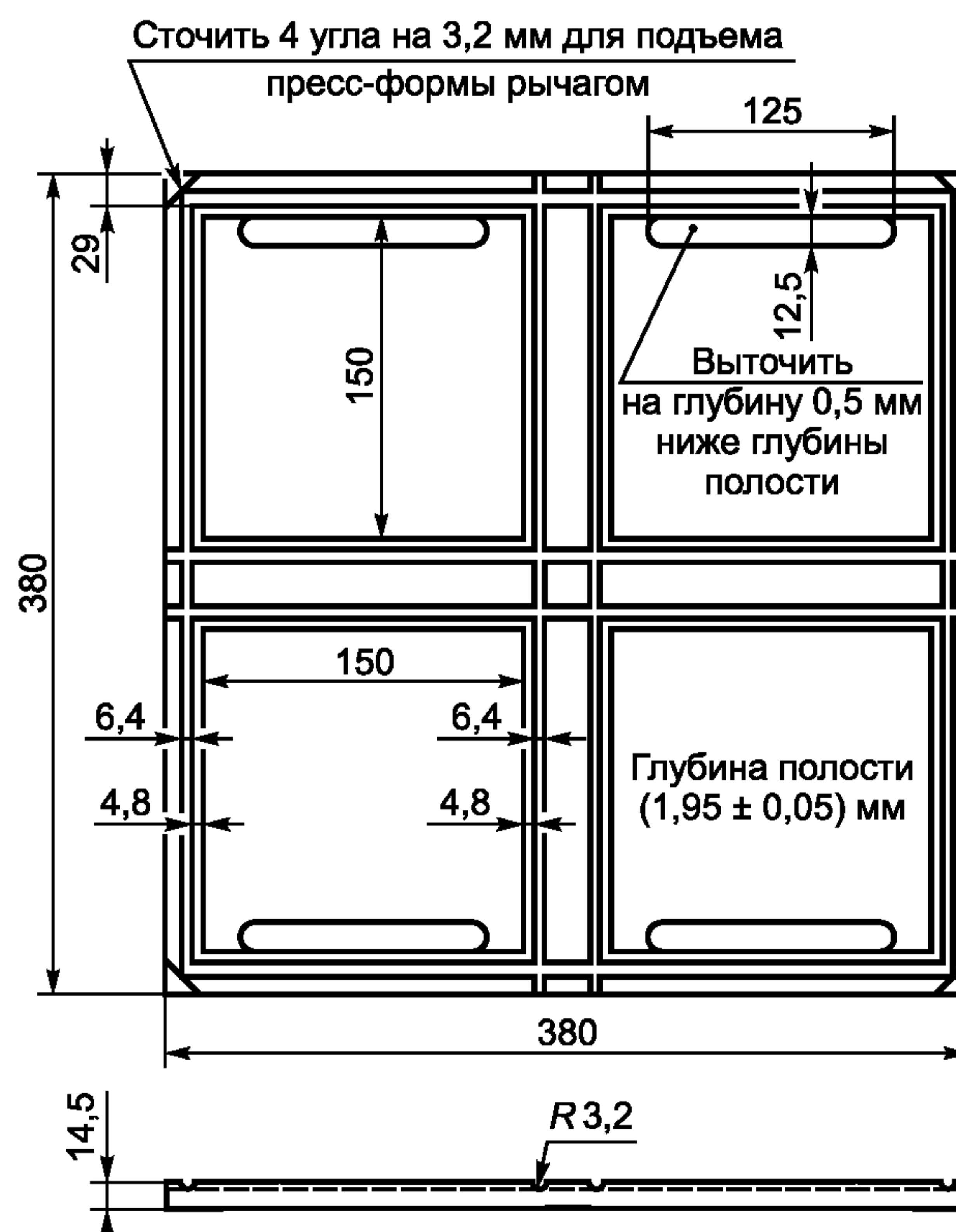
Рисунок 1 — Четырехполосная пресс-форма
